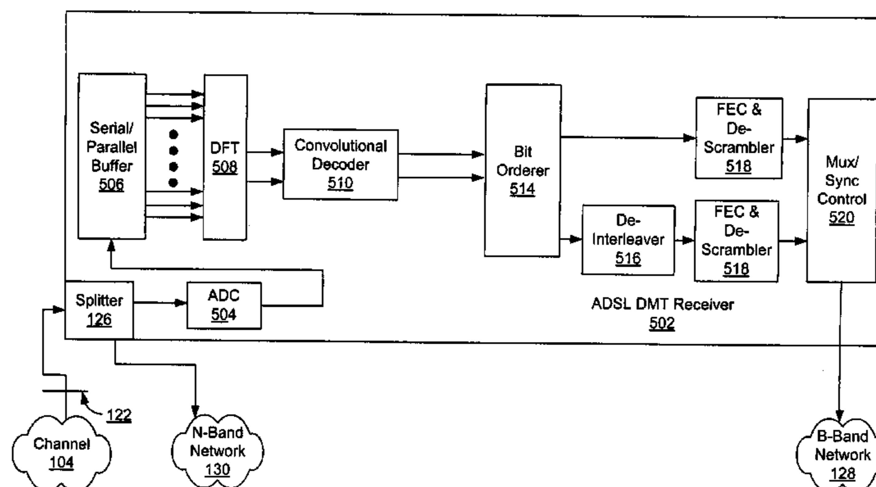
Discrete Multitone Deinterleaver
