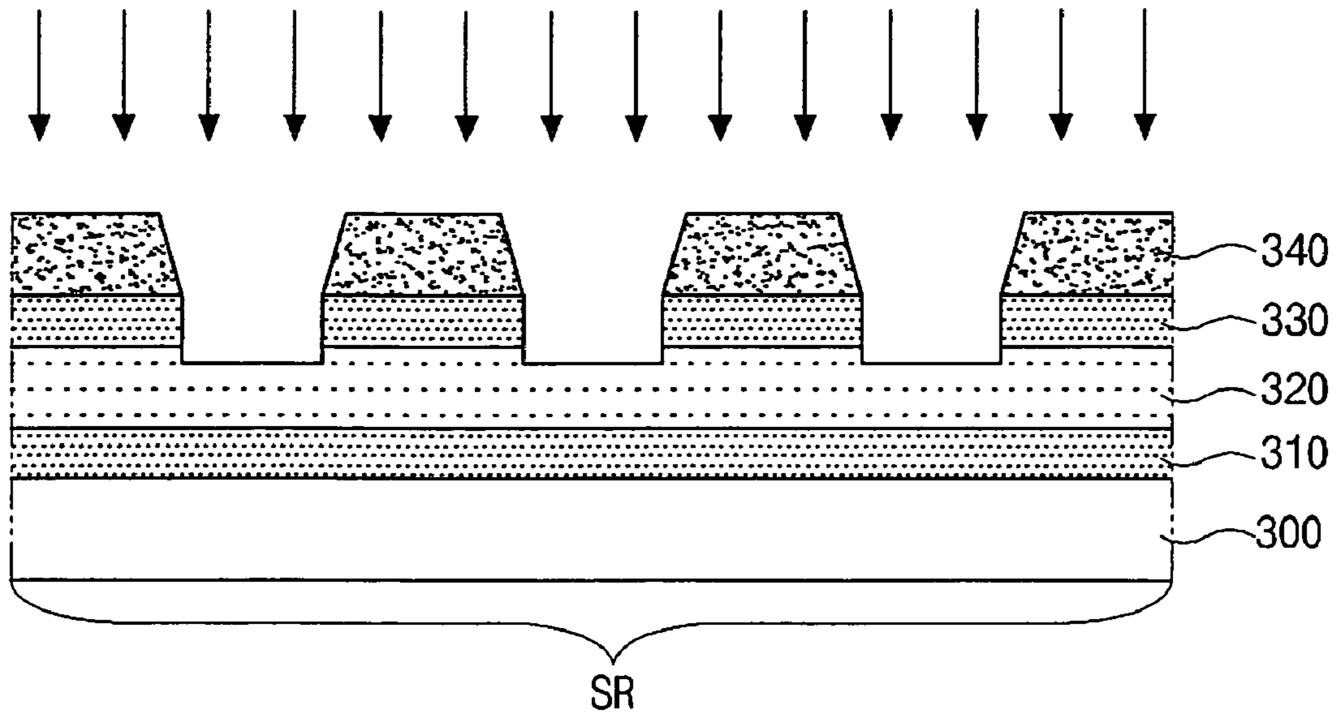
FIG. 11B
