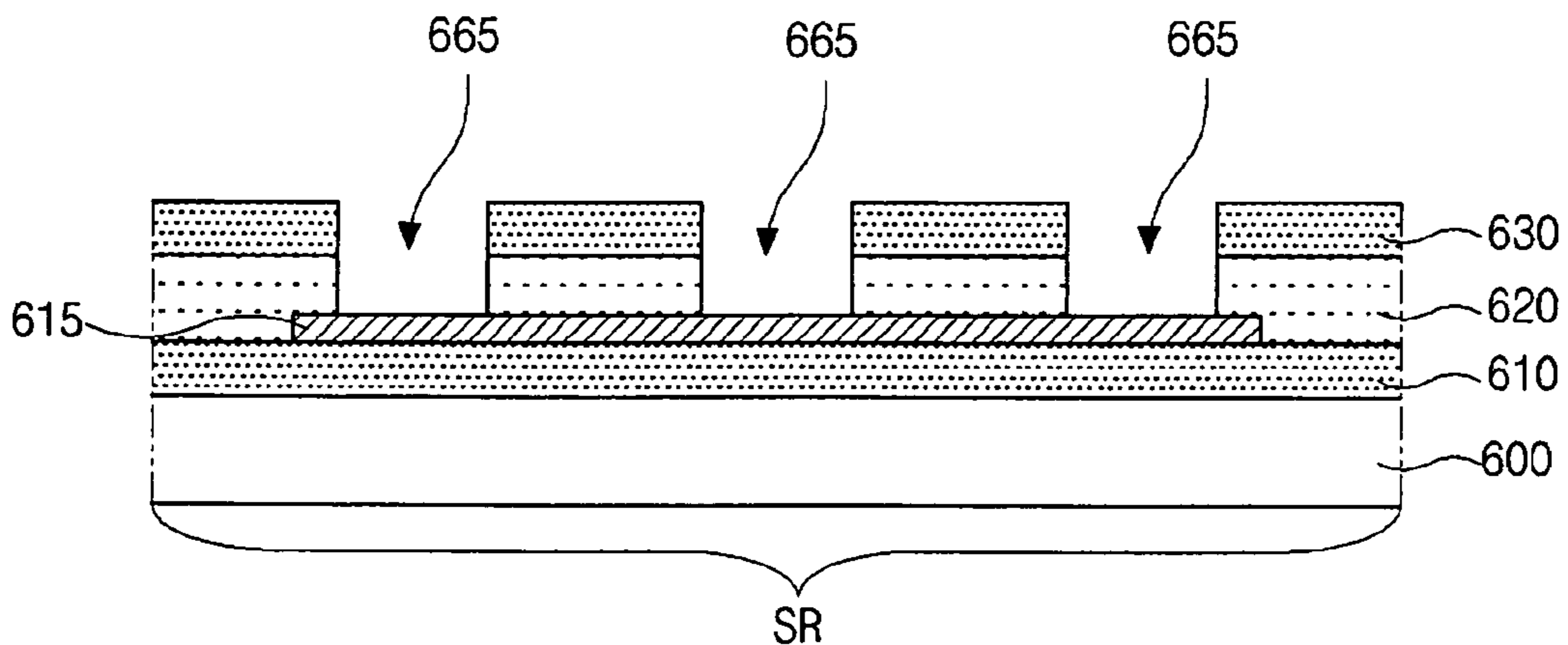
FIG. 14B
