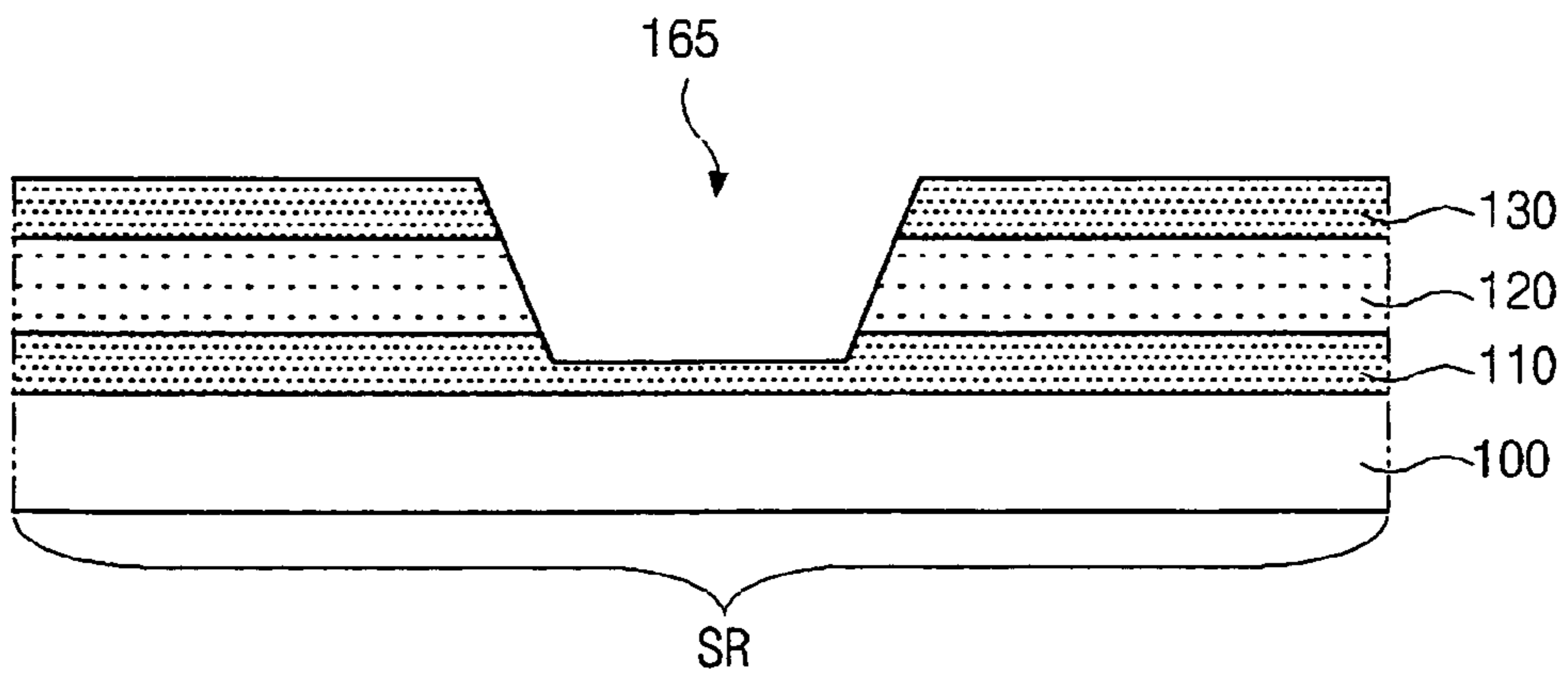
FIG. 9D
