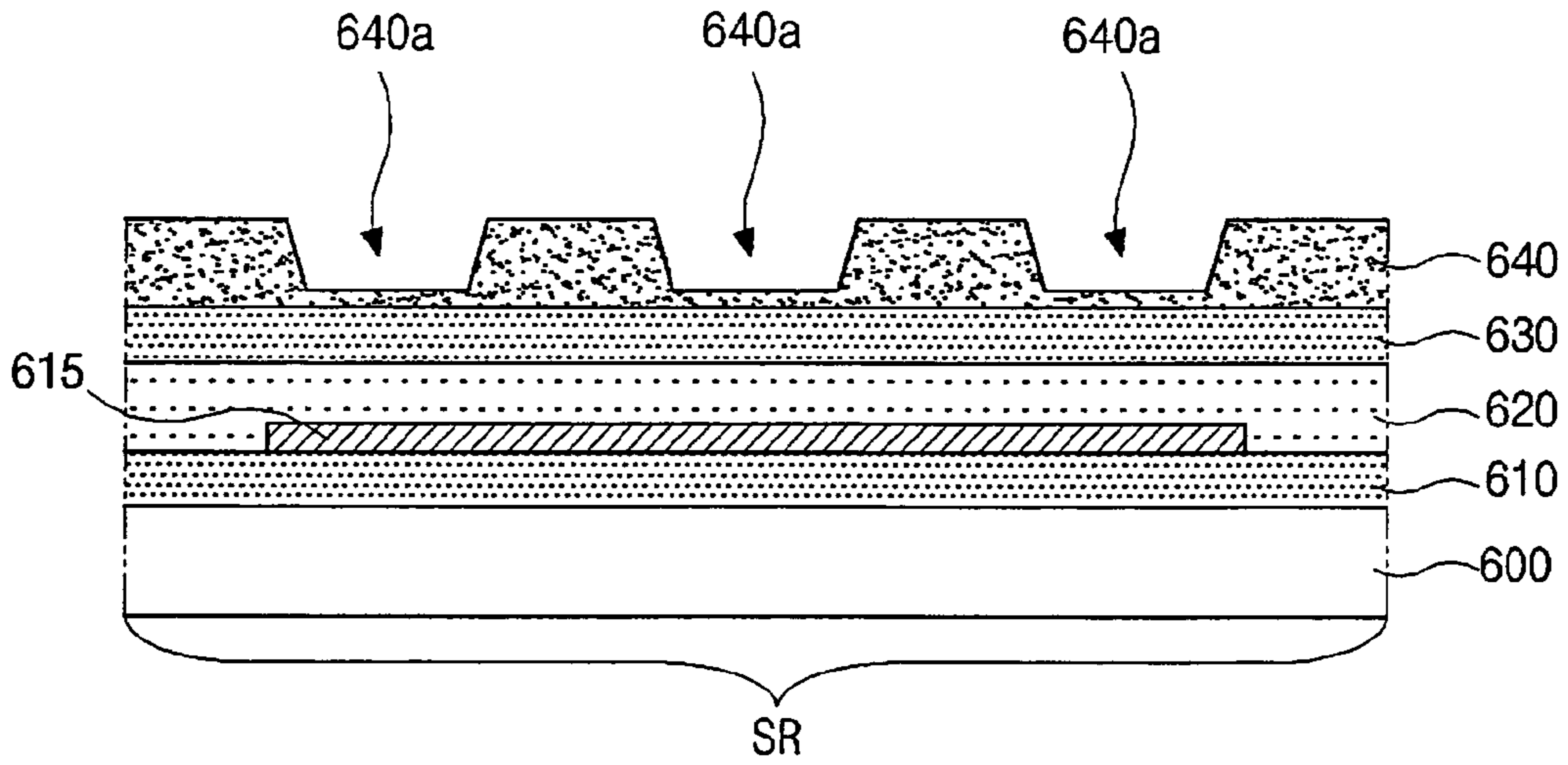
FIG. 14A
