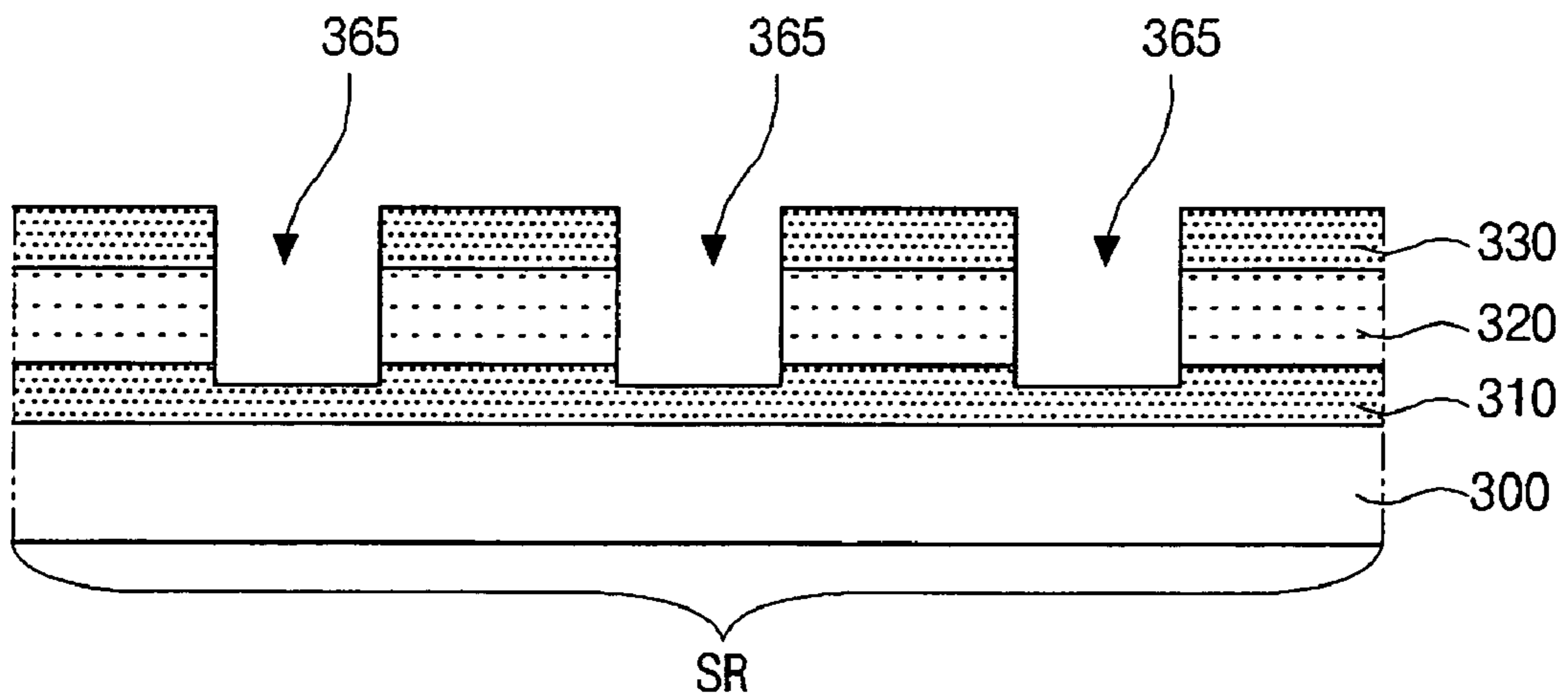
FIG. 11C
