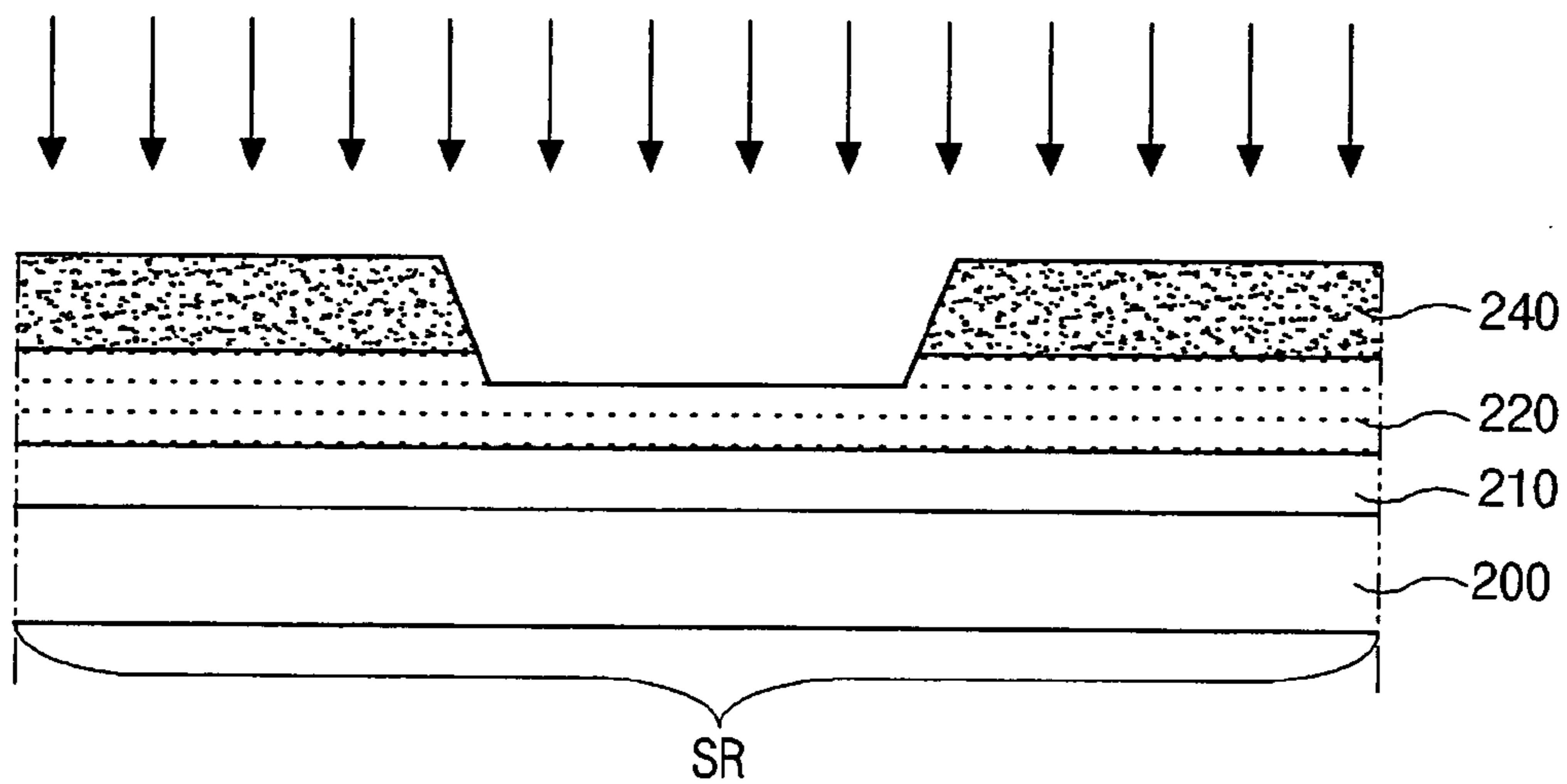
FIG. 10C
