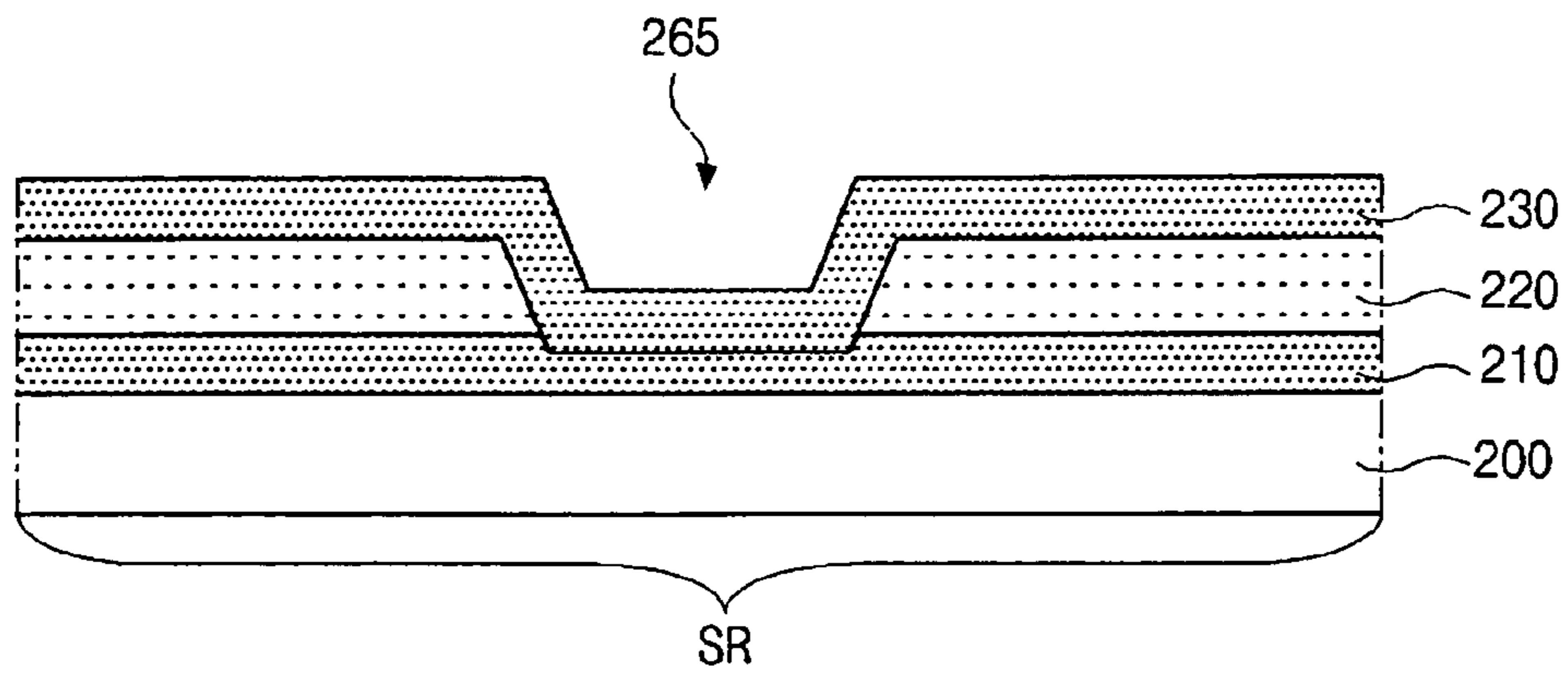
FIG. 10E
