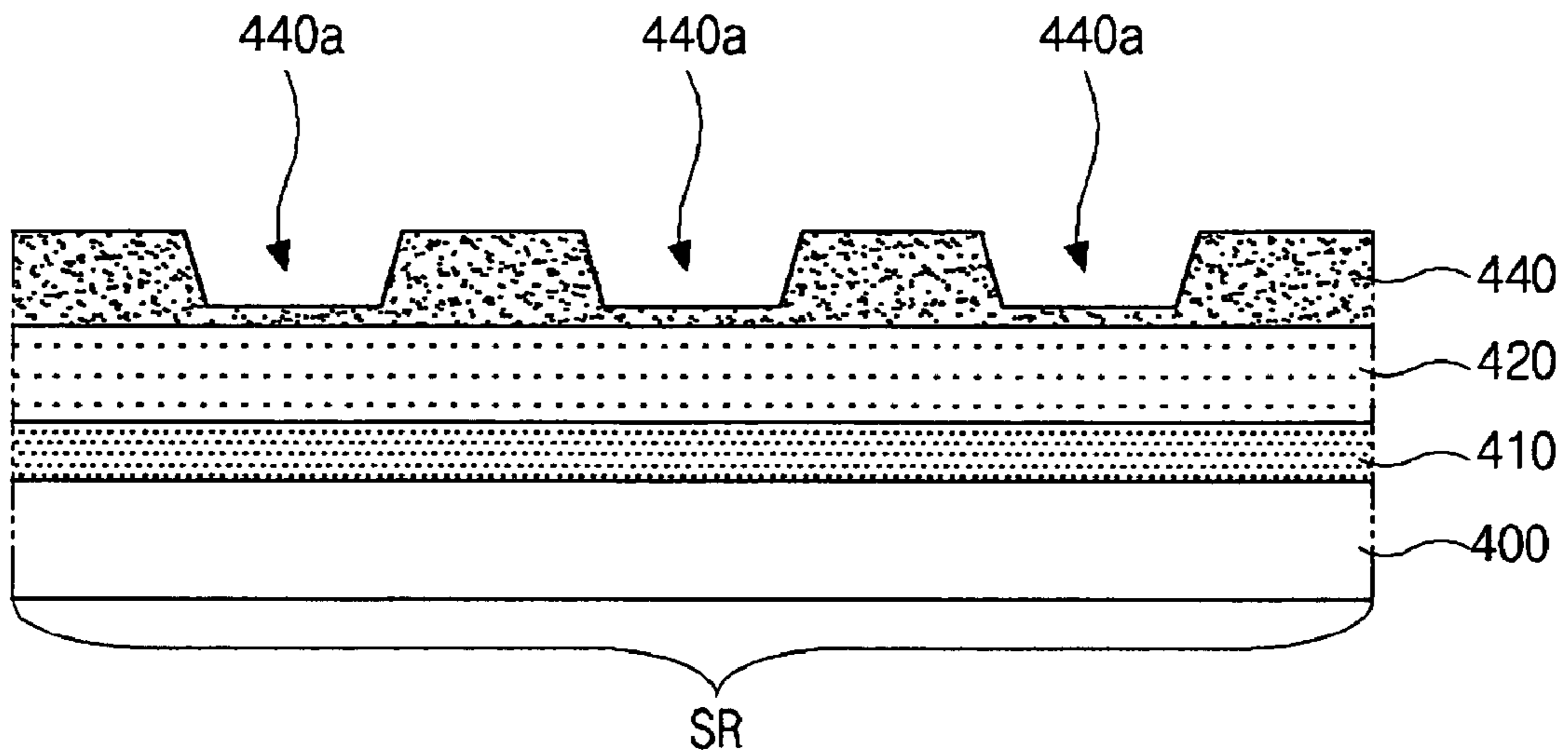
FIG. 12A
