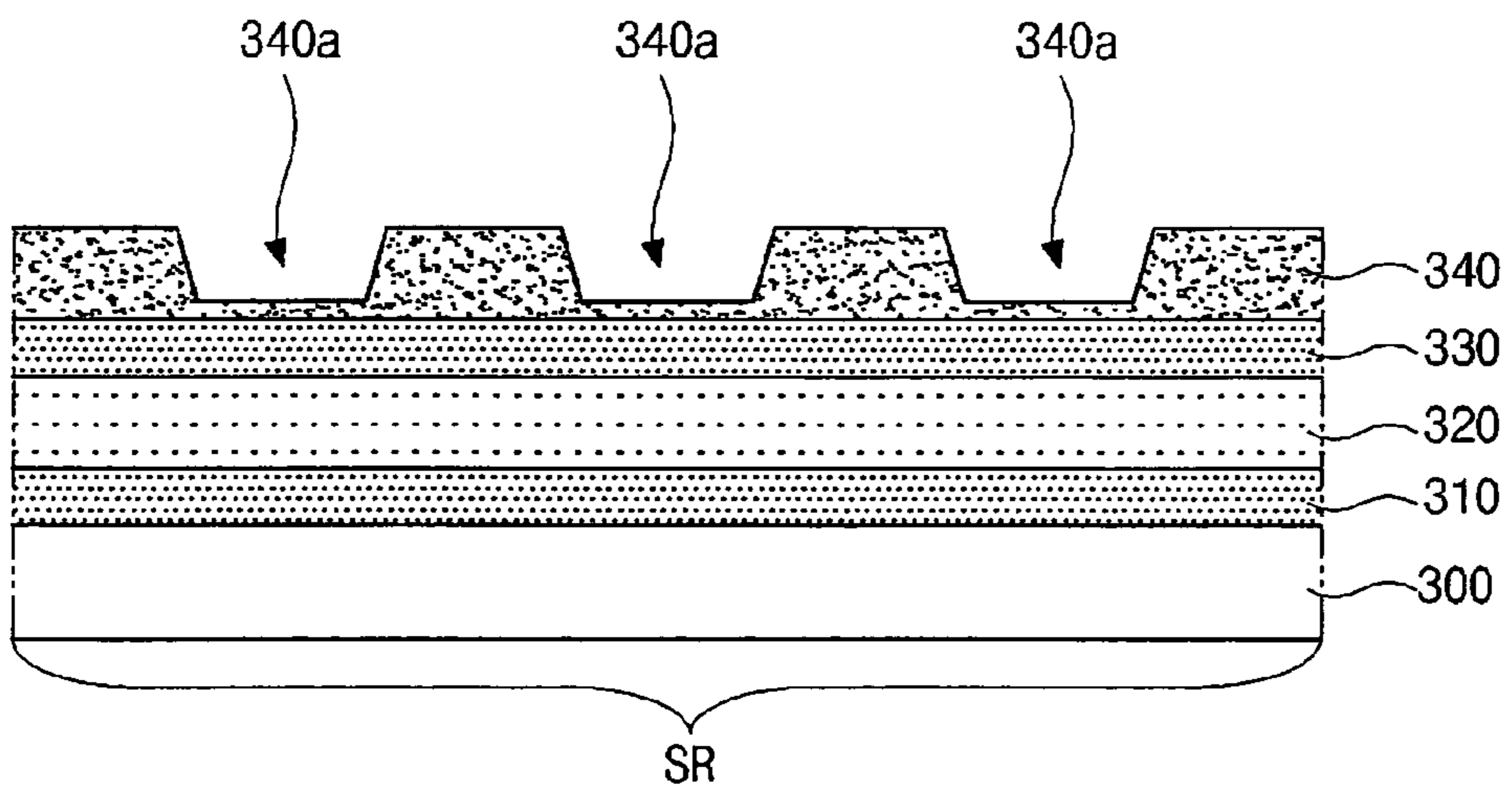
FIG. 11A
