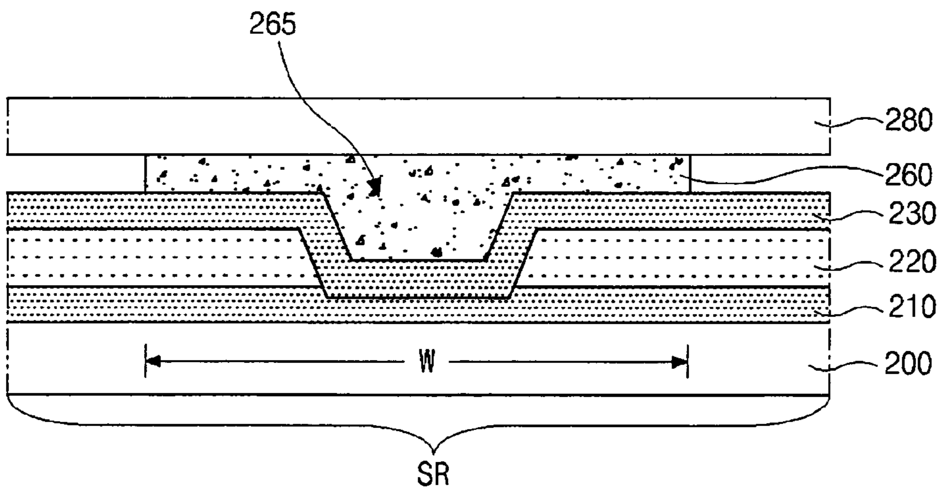
FIG. 10F
