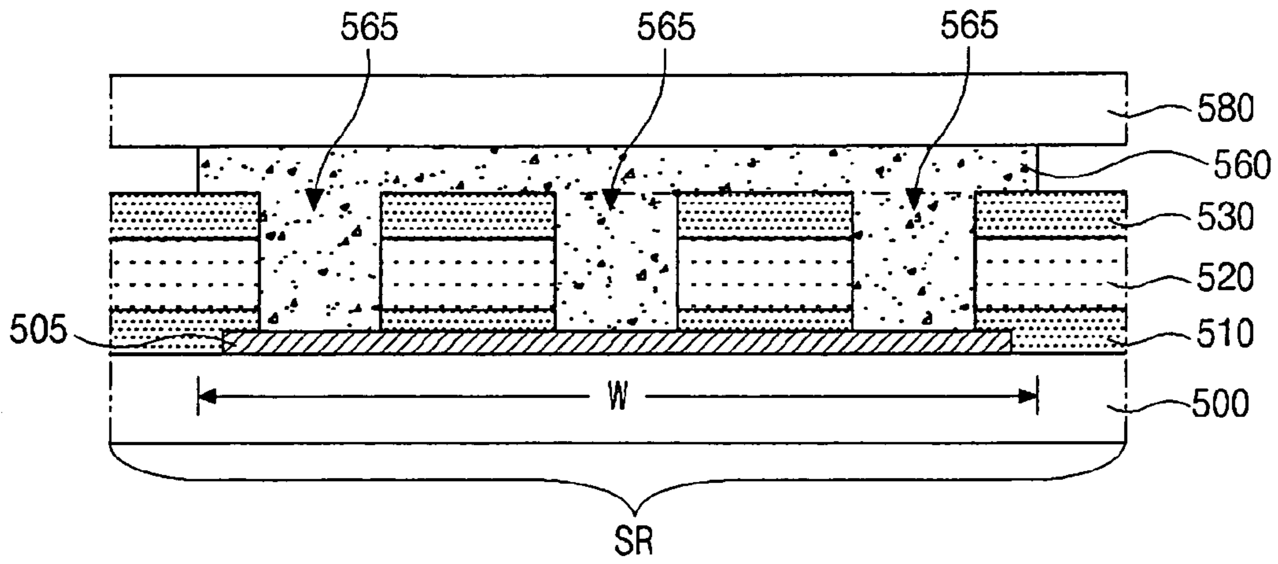
FIG. 13C
