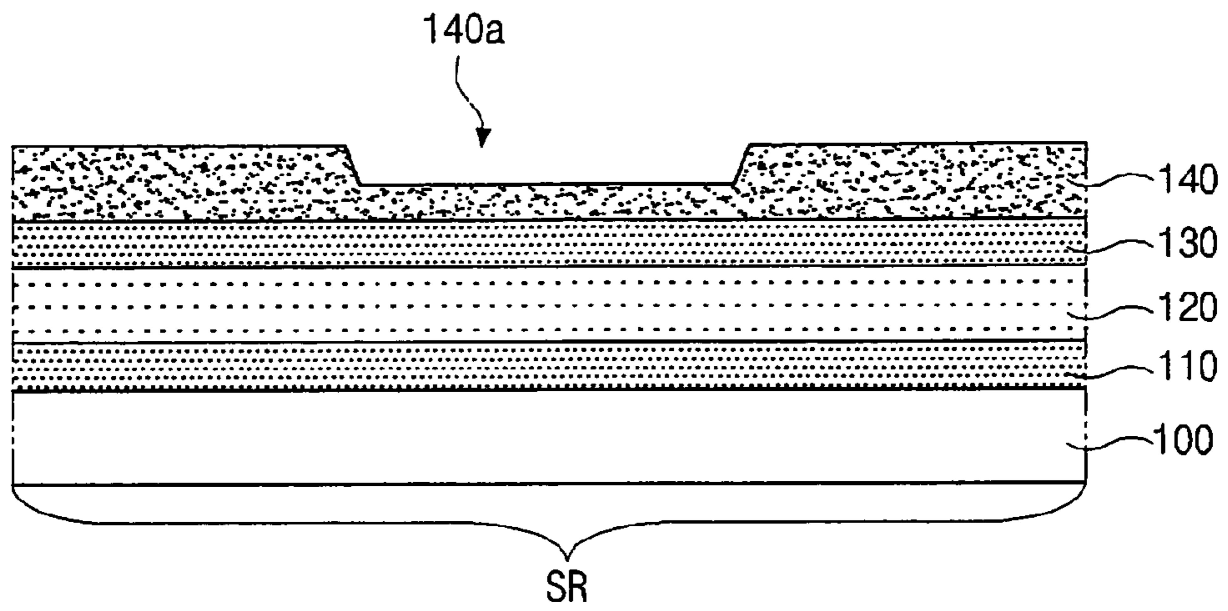
FIG. 9B
