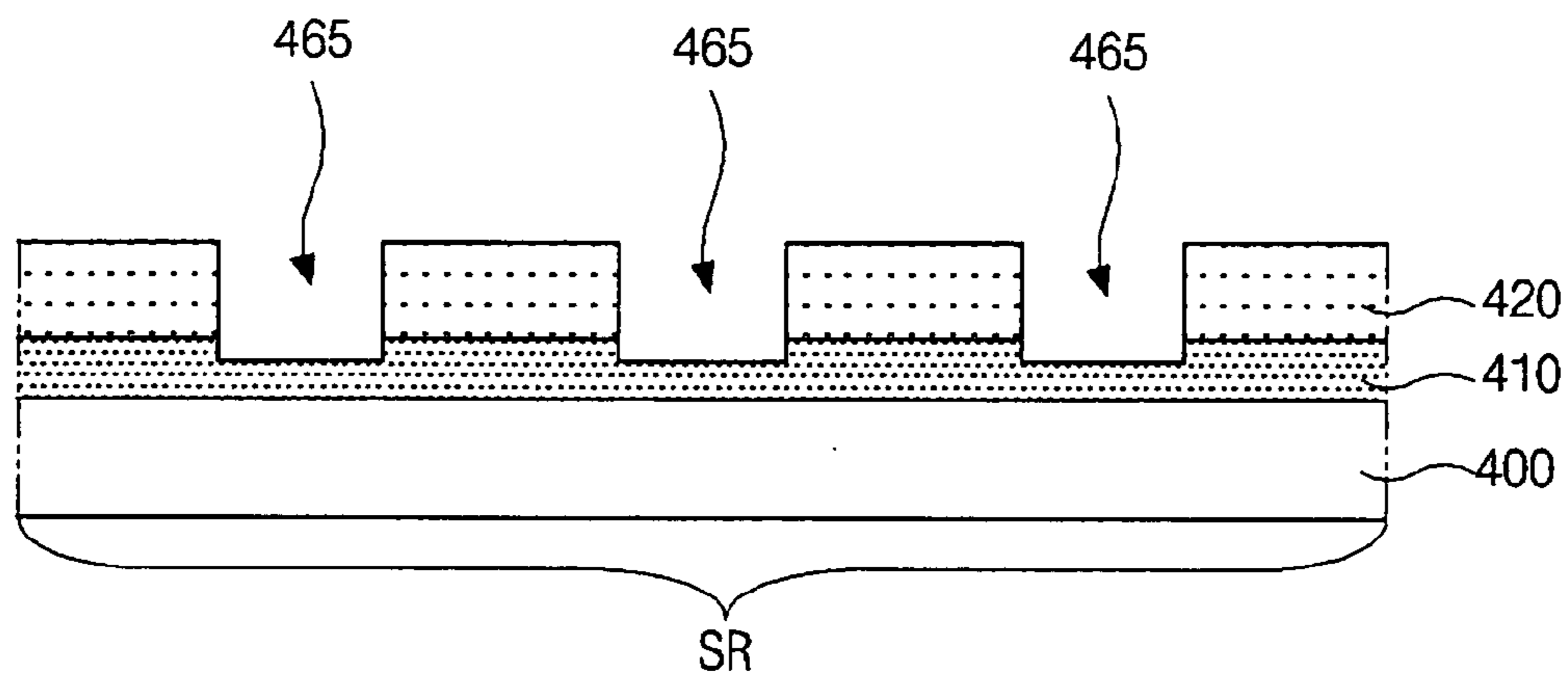
FIG. 12C
