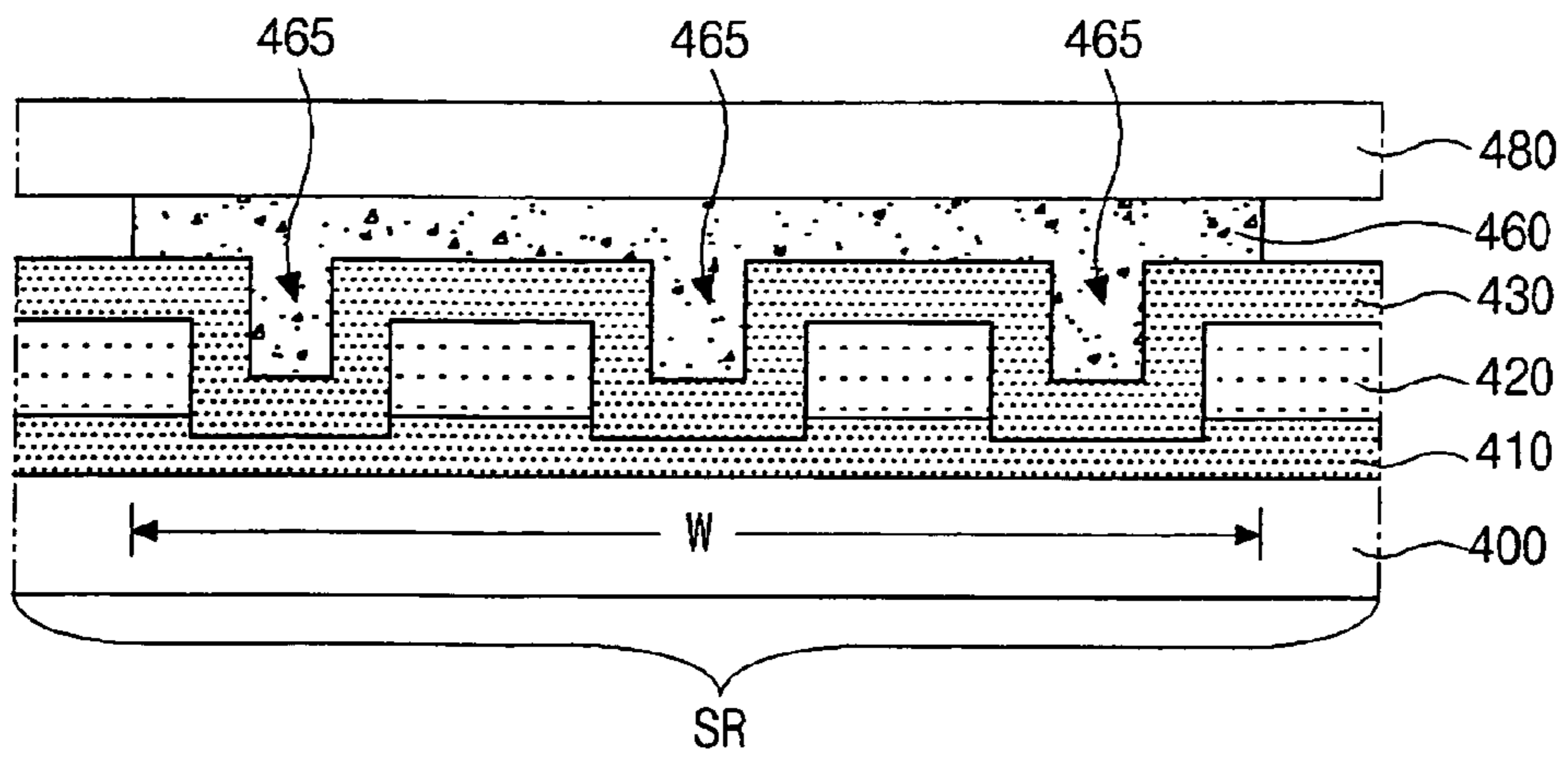
FIG. 12E
