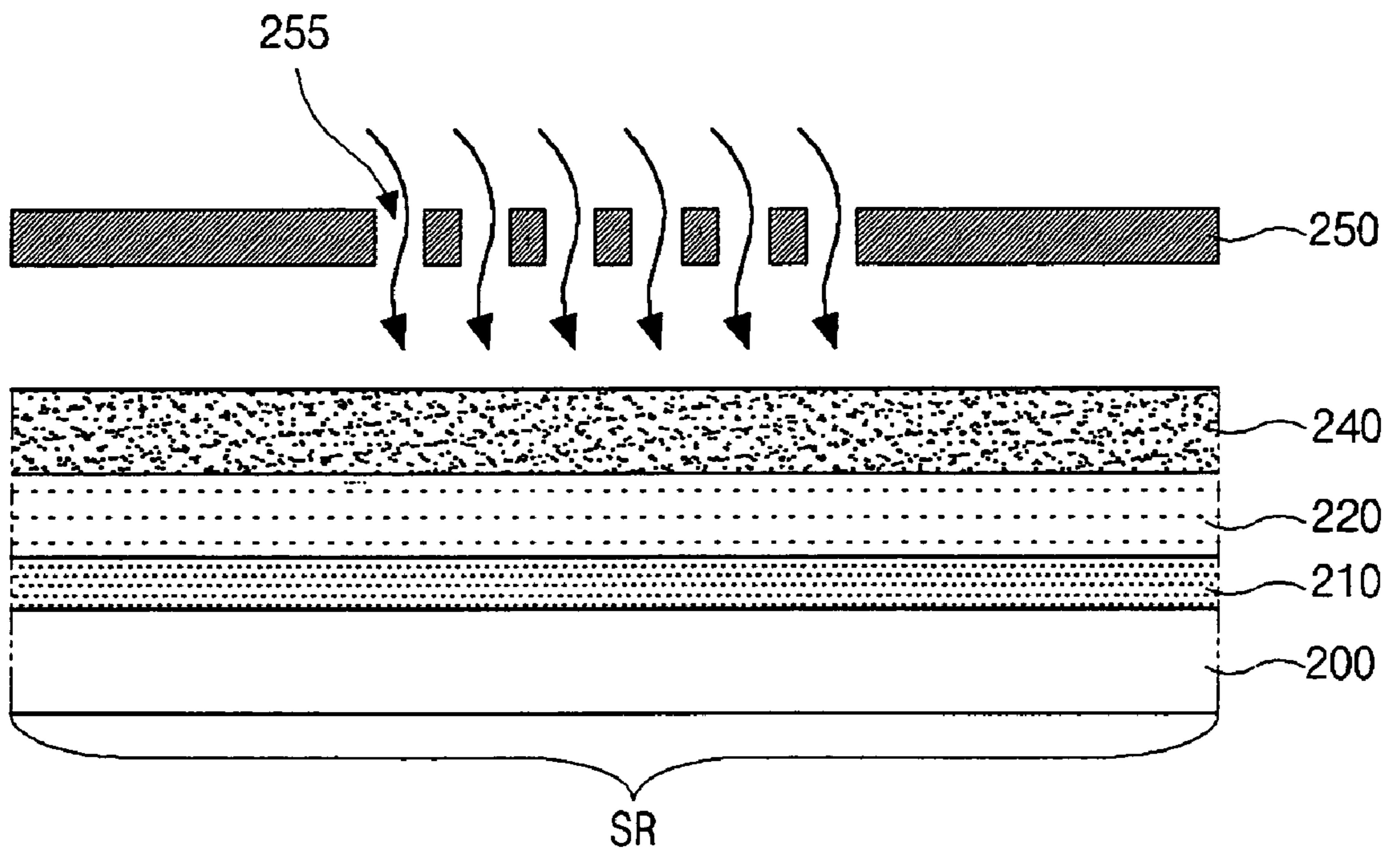
FIG. 10A
