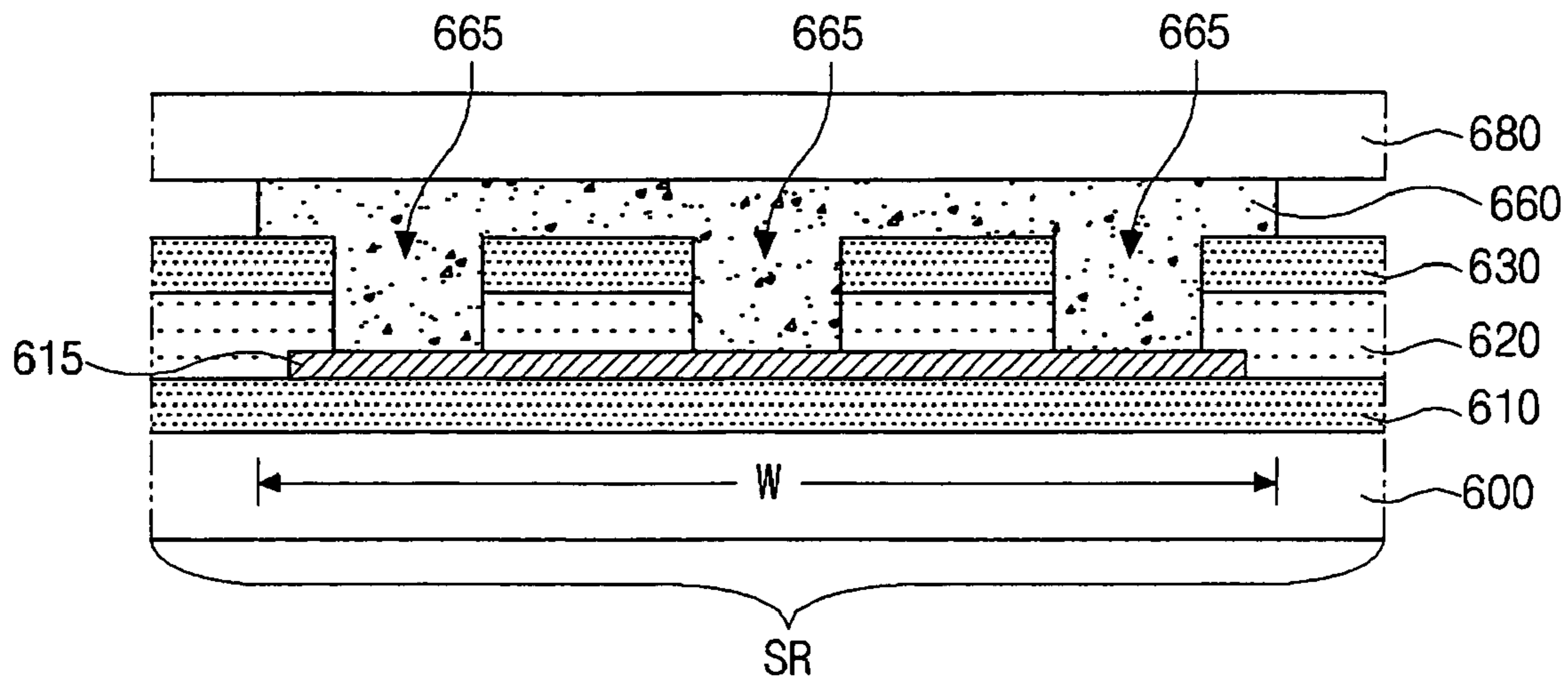
FIG. 14C
