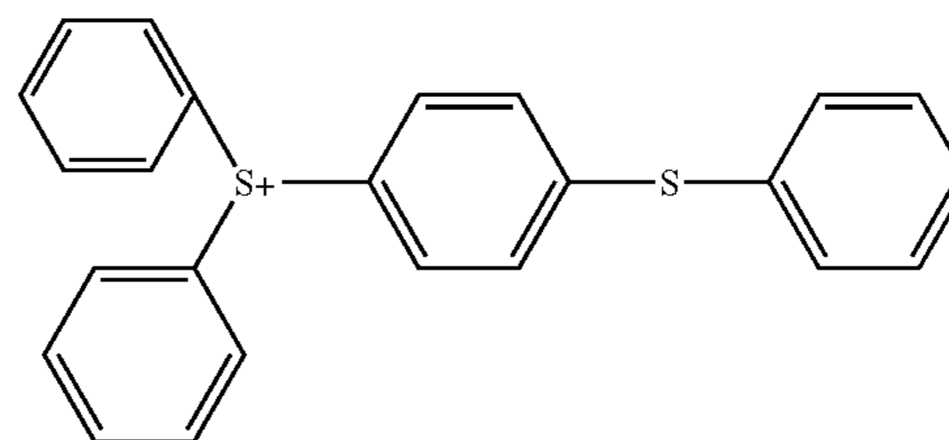
PF6-
