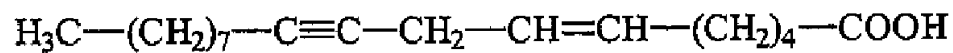
6,9-Octadecenynoic acid
