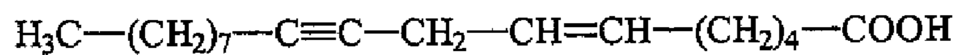
6,9-Octadecenynoic acid
