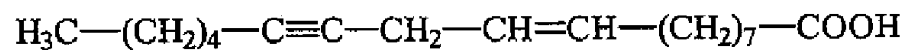
Crepenynic acid
