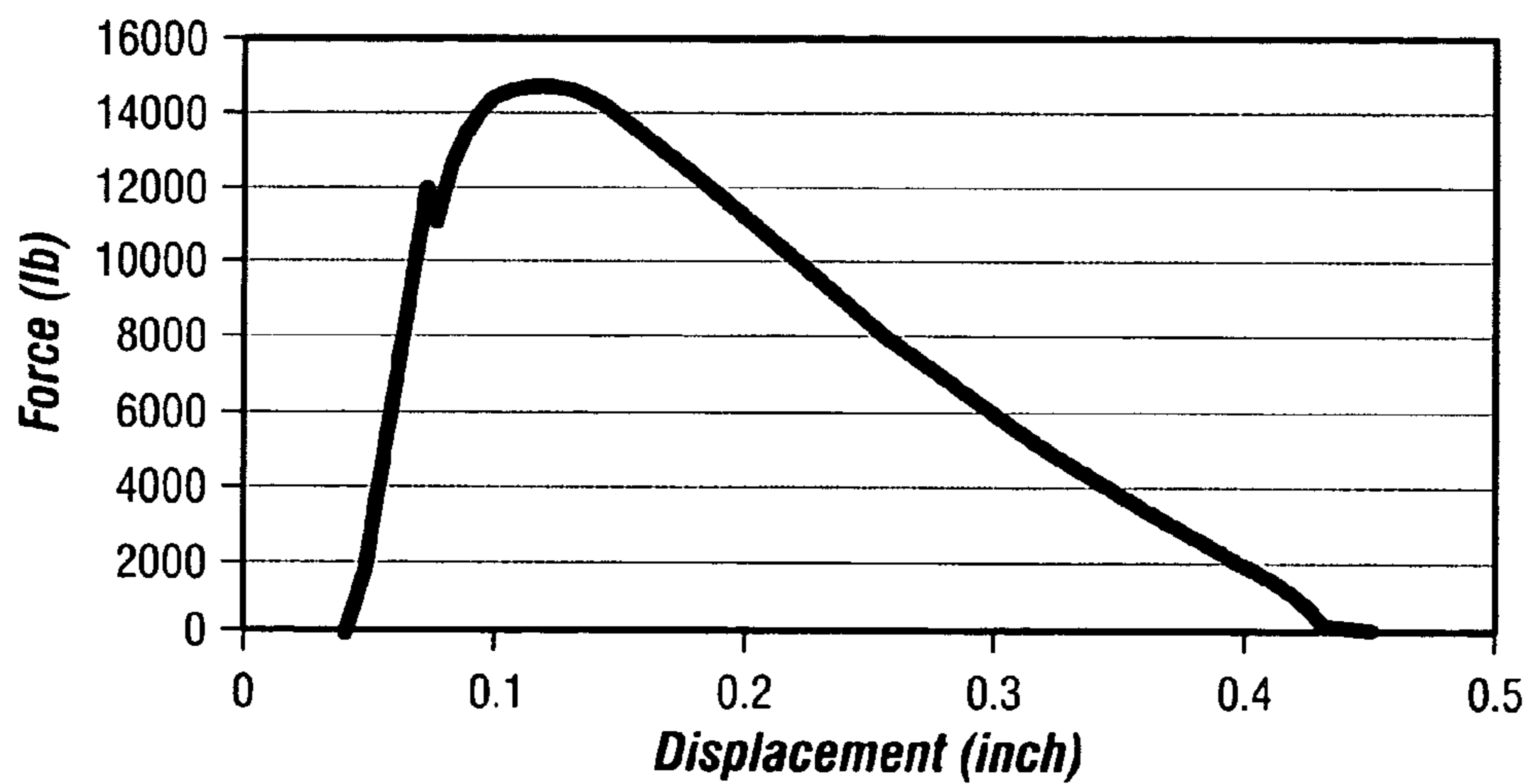
FIG. 11
