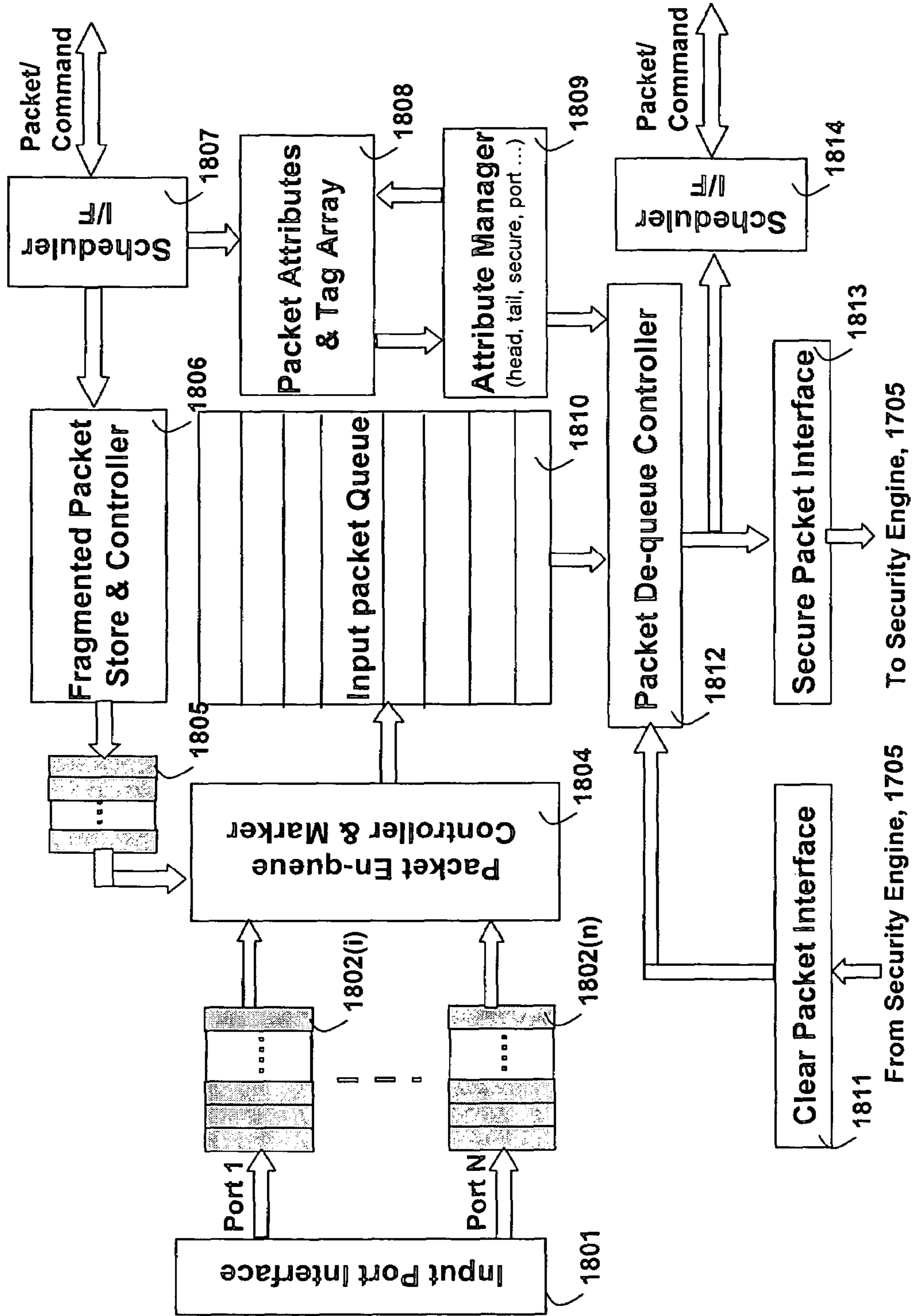
Fig. 18 Input Queue & Controller
