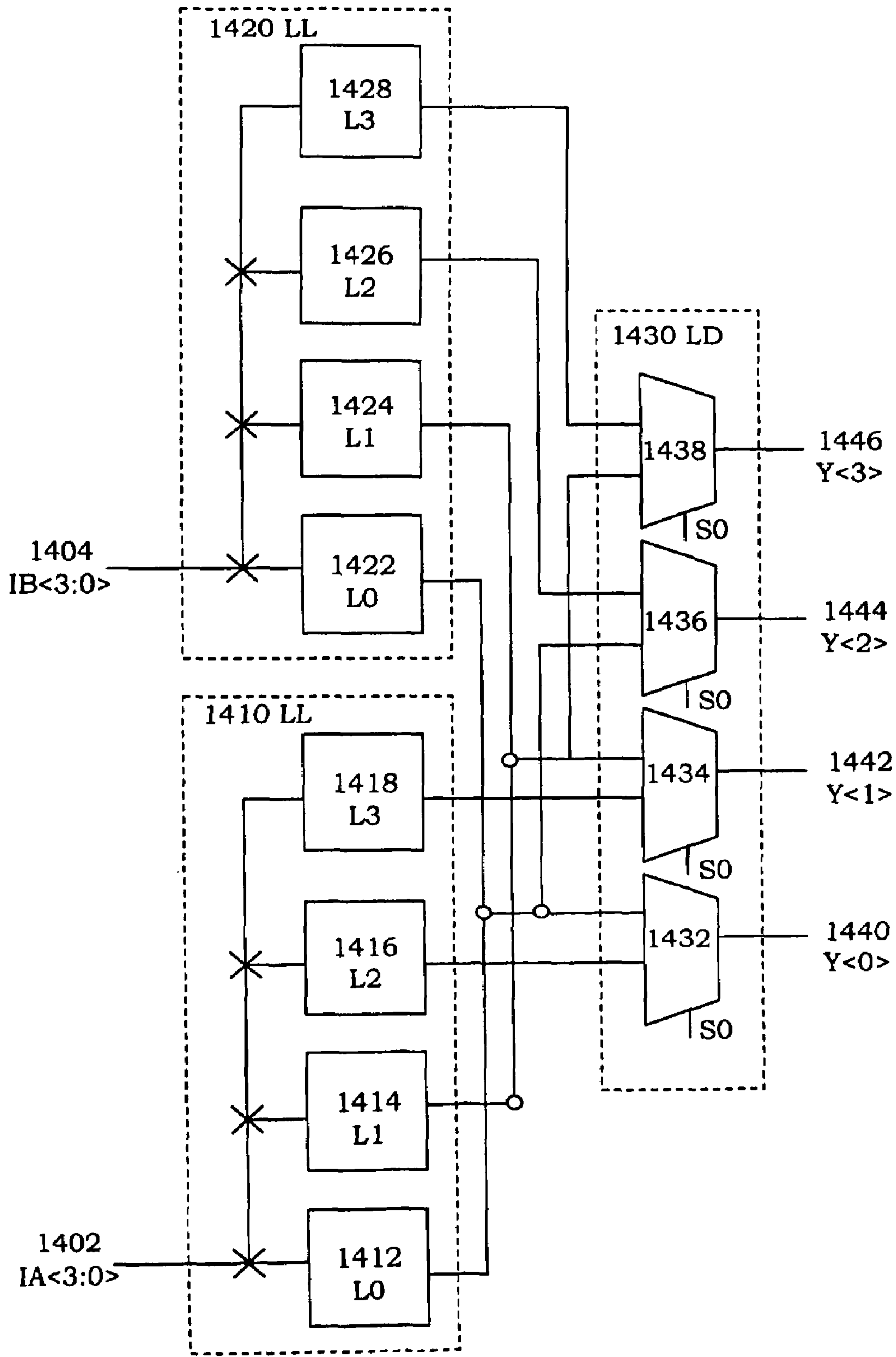
1400 4 2:1 multiplexer FIG. 14
