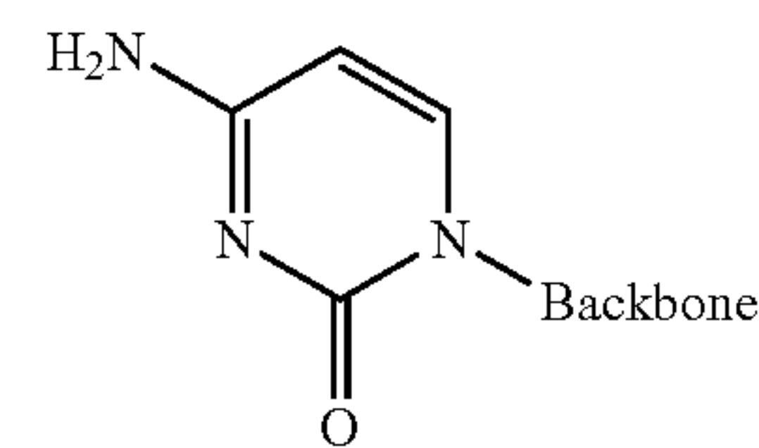
Cytosine
