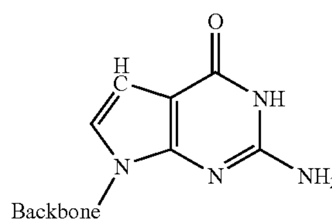
7-deaza guanine
