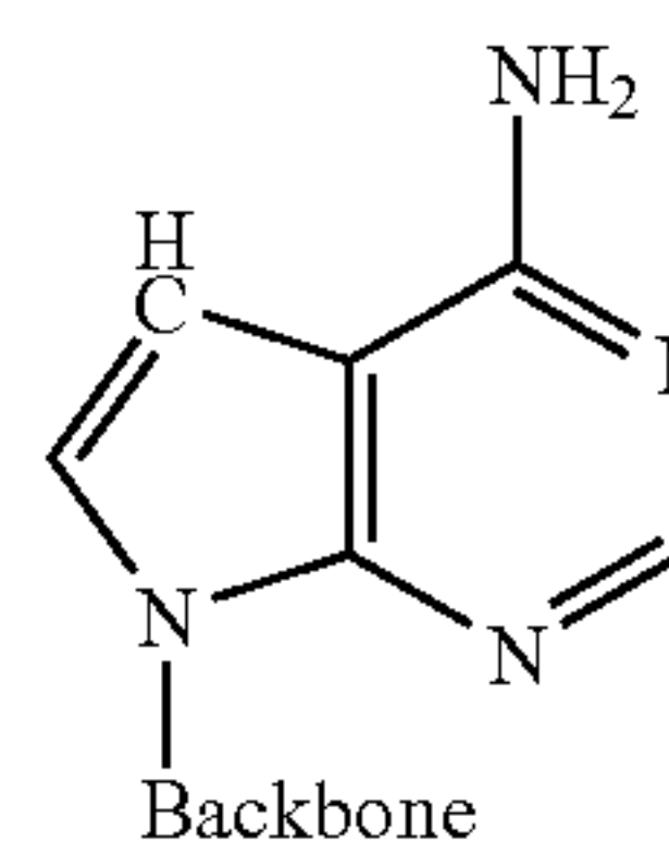
7-deaza adenine
