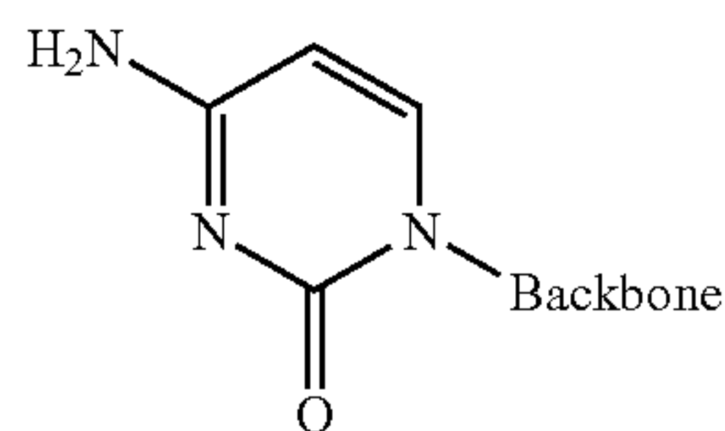
Cytosine
