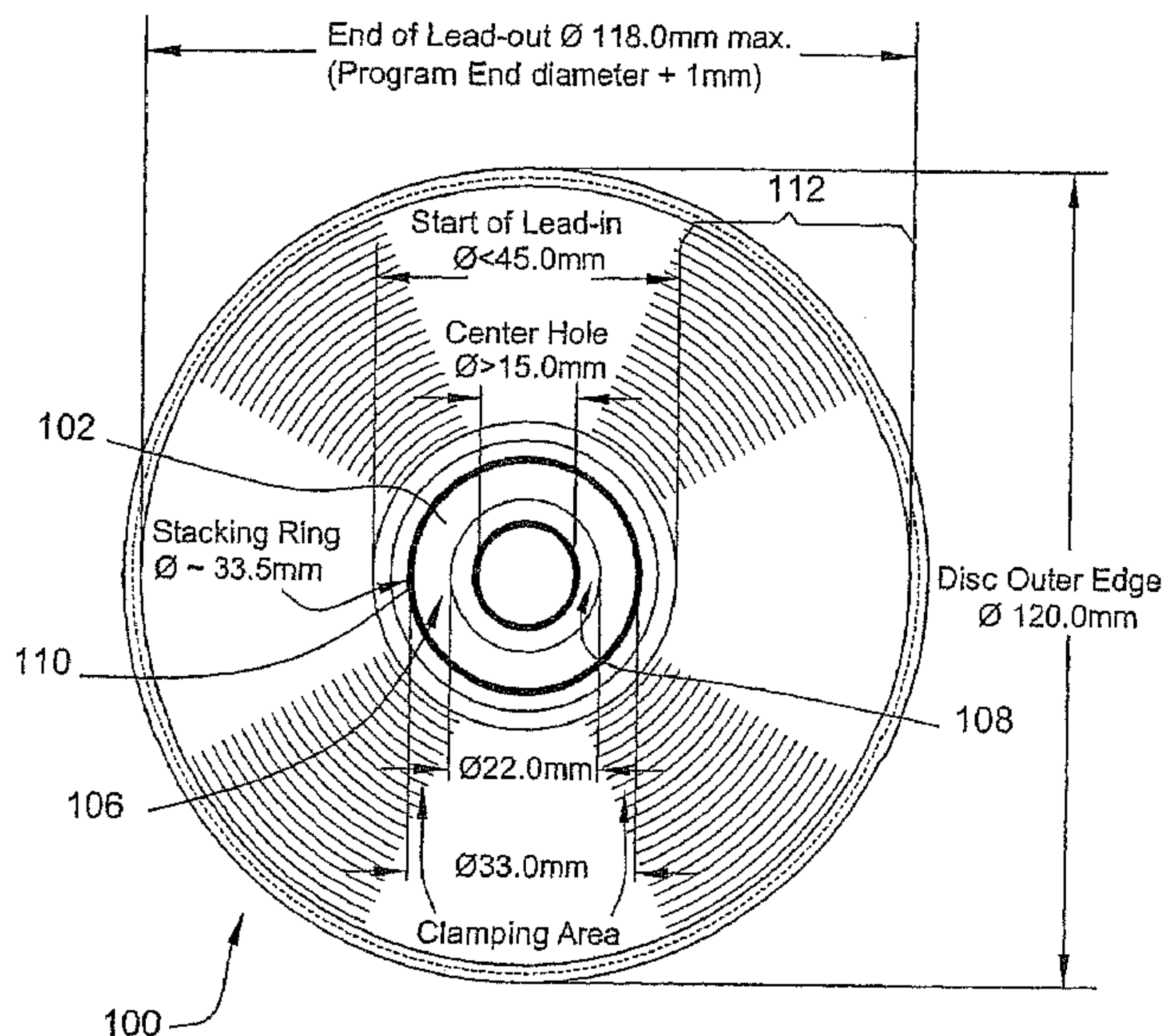
DVD DIMENSIONS
