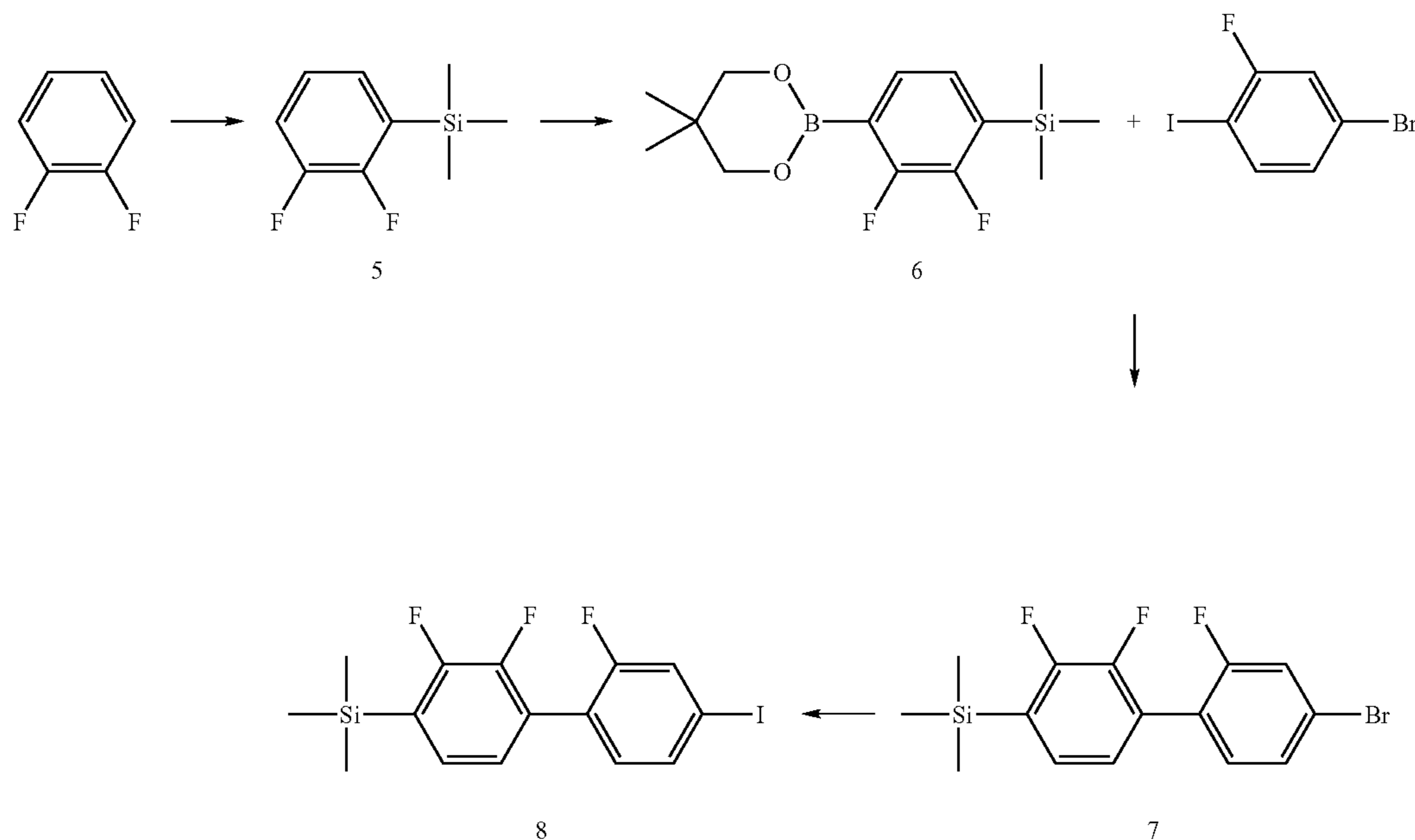
1,2-Difluoro-3-trimethylsilylbenzene (5)
