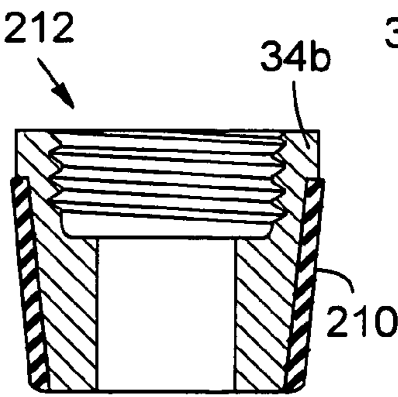
FIG. 14
