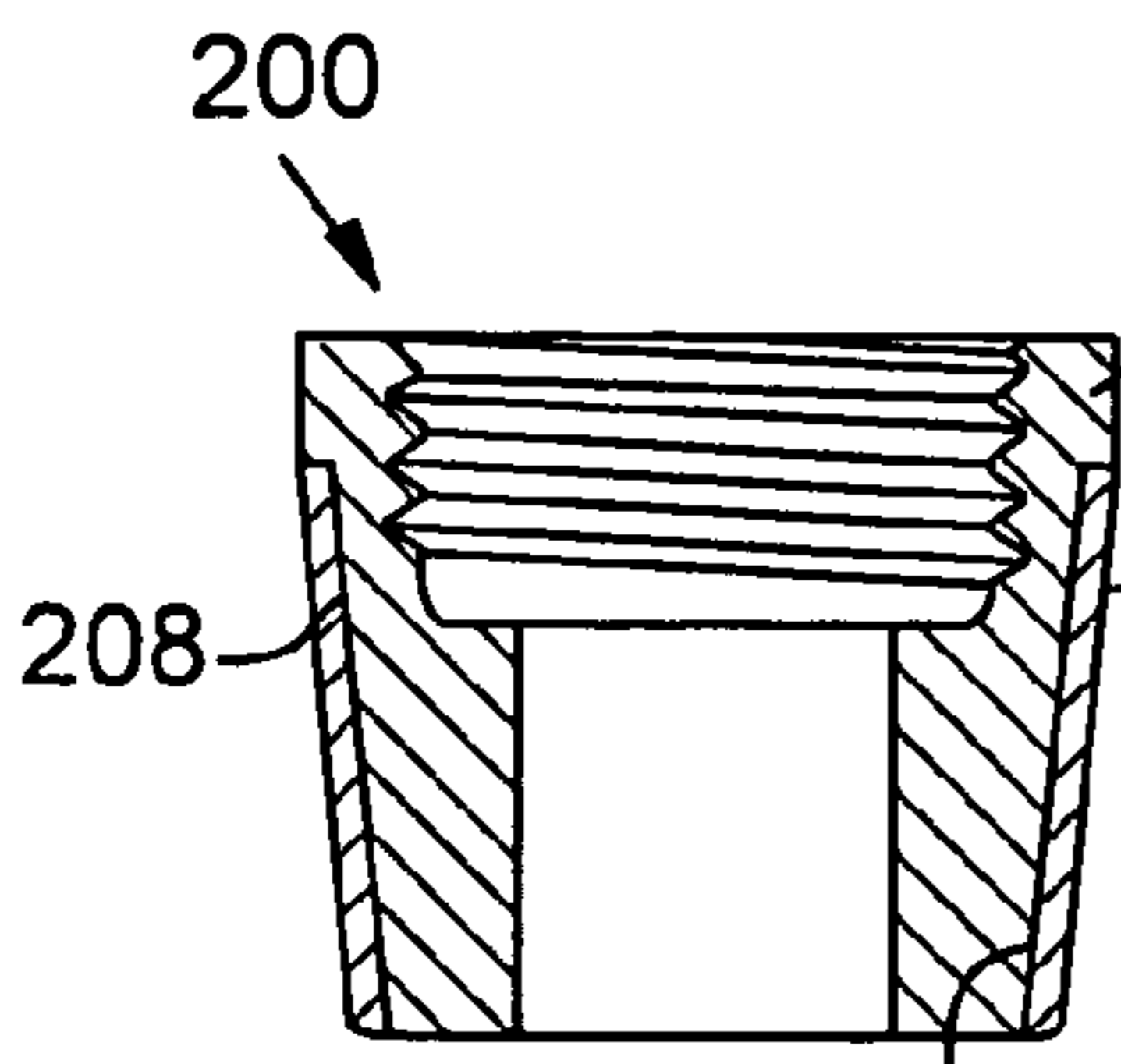
FIG. 13
