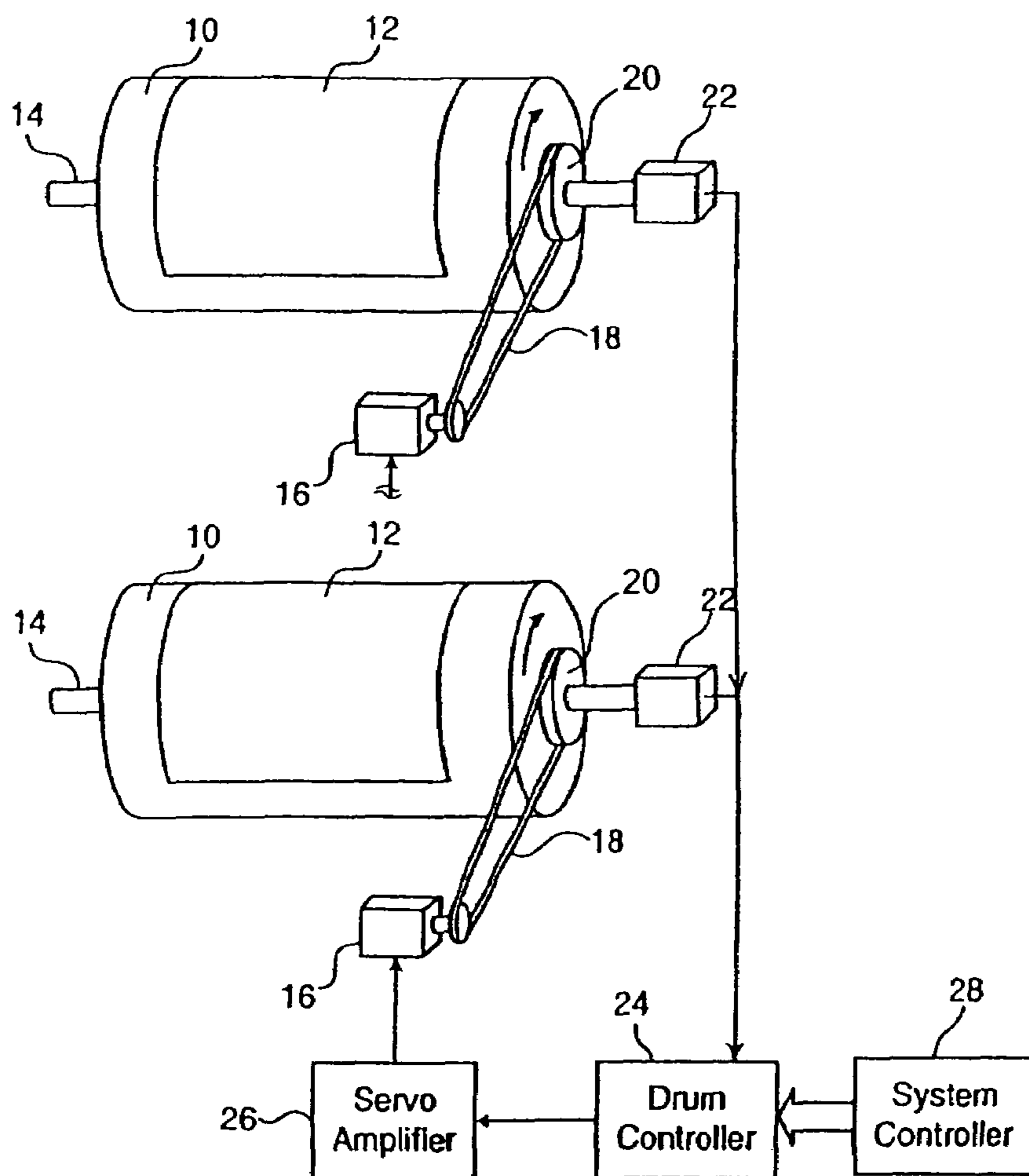
FIG. 1-A PRIOR ART
