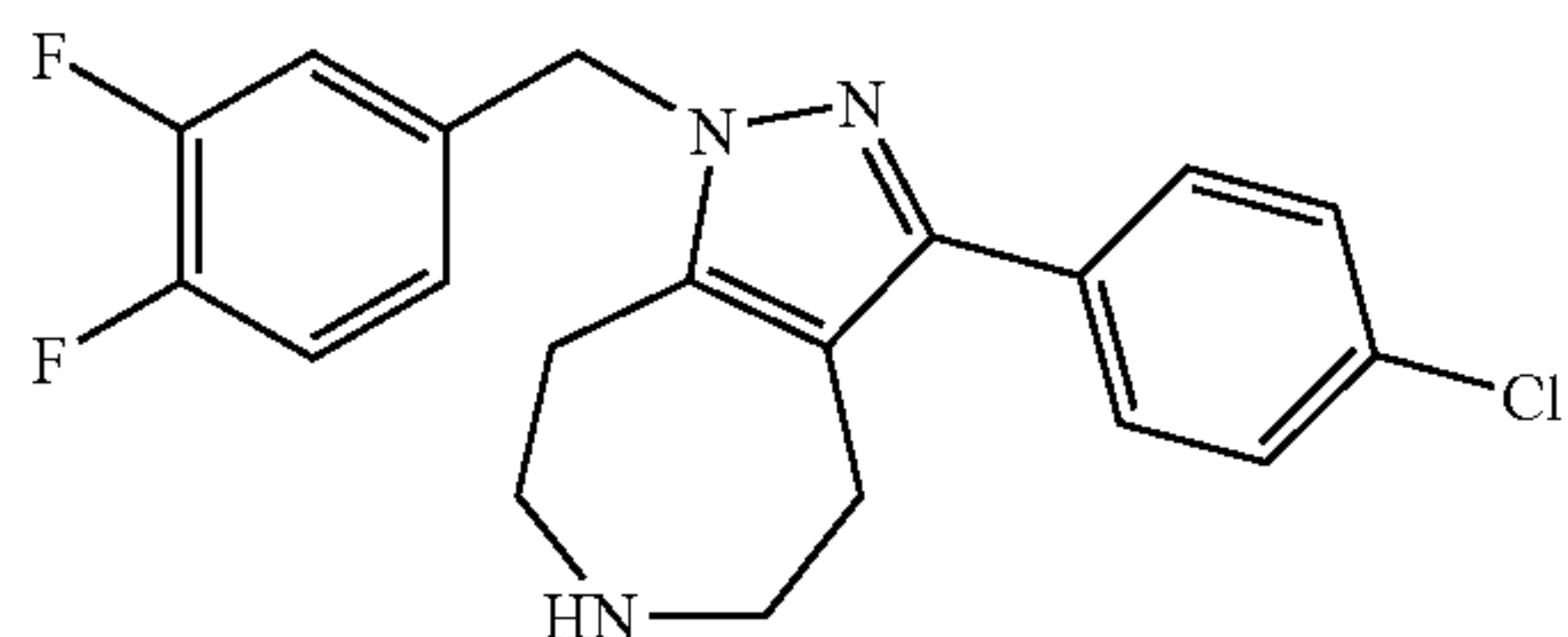
3-(4-Chloro-phenyl)-1-(3,4-difluoro-benzyl)-1,4,5,6, 7,8-hexahydro-1,2,6-triaza-azulene
