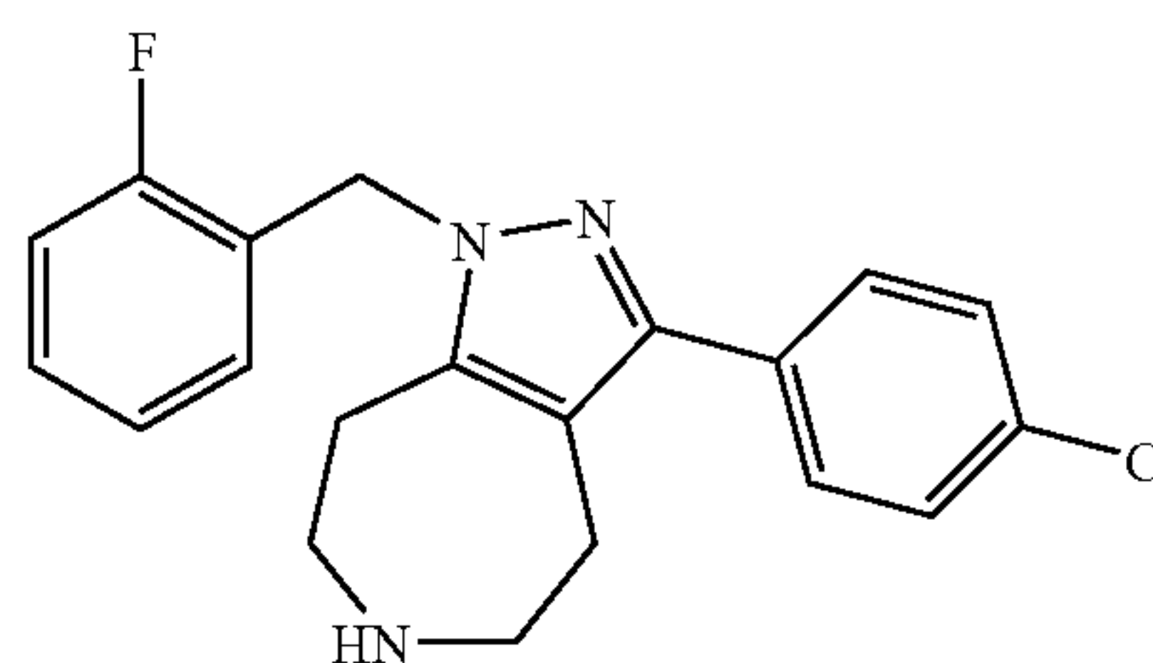
3-(4-Chloro-phenyl)-1-(2-fluoro-benzyl)-1,4,5,6,7,8-hexahydro-1,2,6-triaza-azulene
