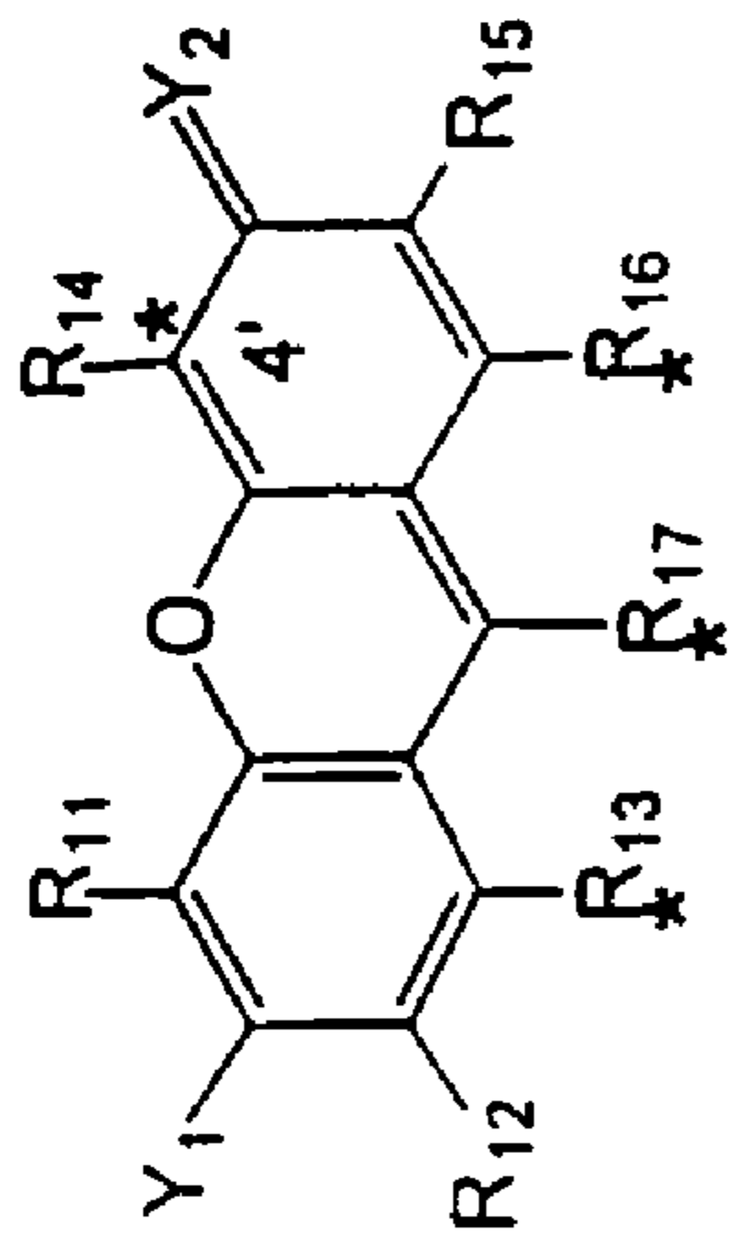
XANTHENE
