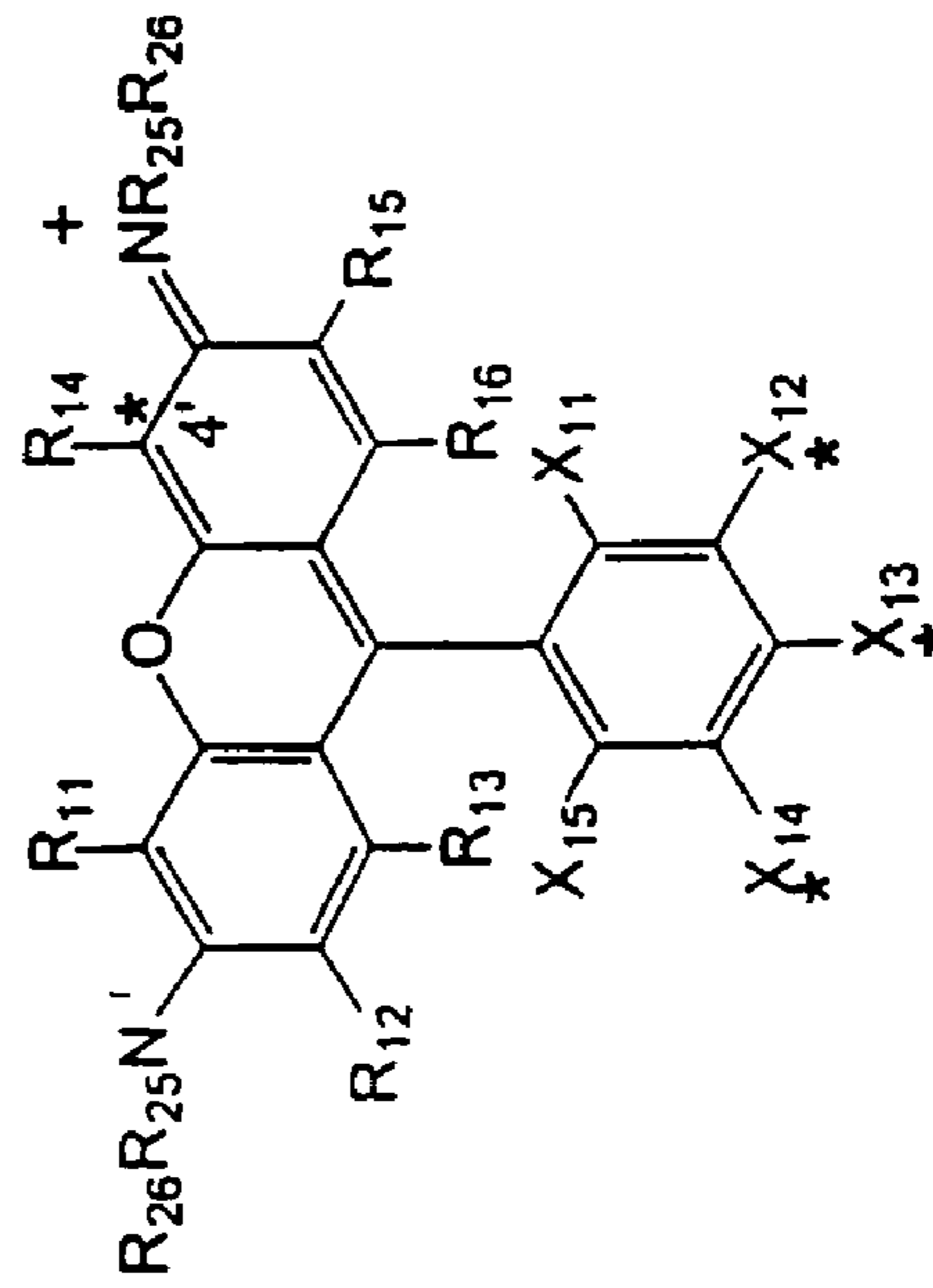
RHODAMINE
