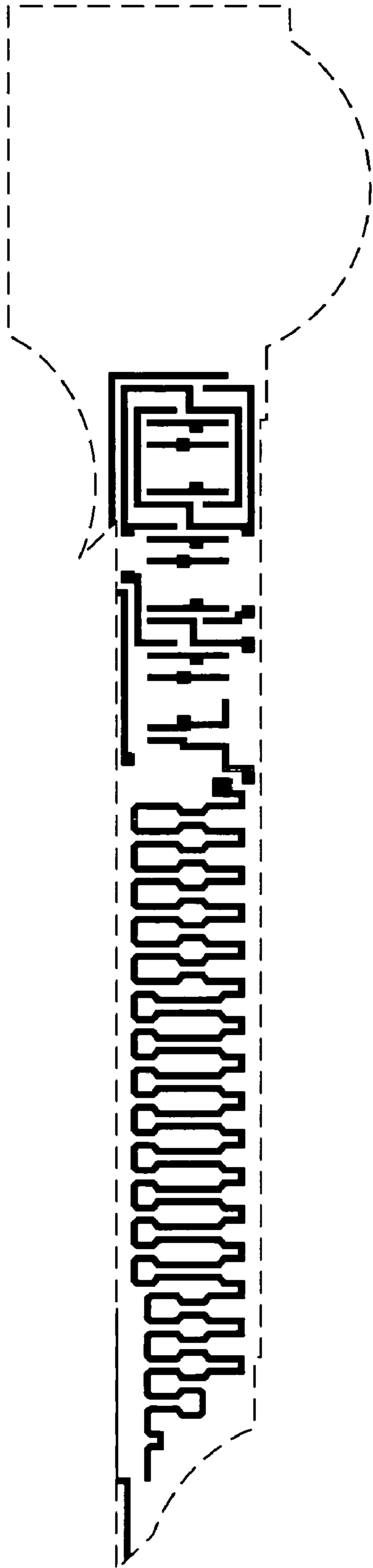
Poly mask
