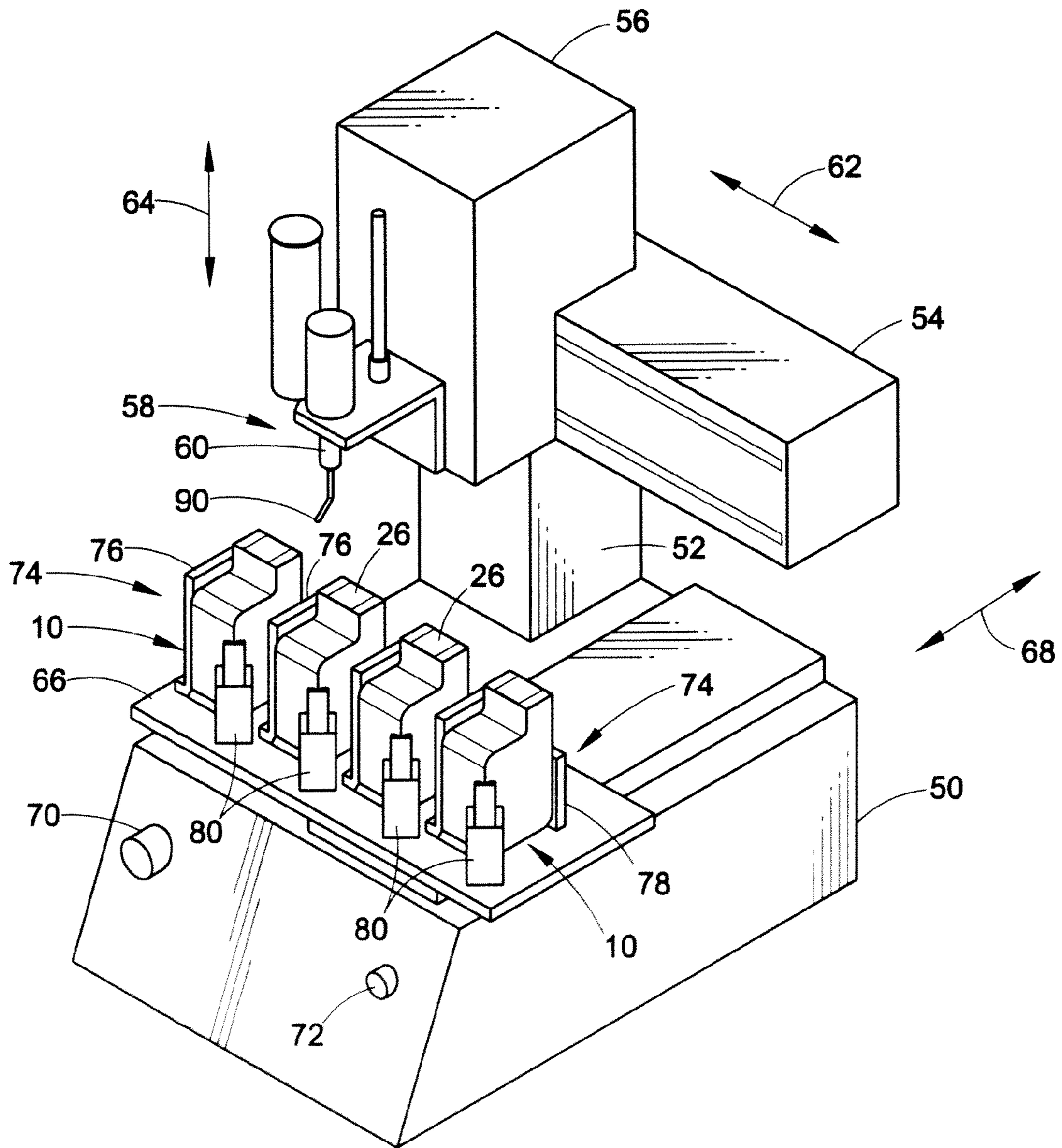
FIG. 14
