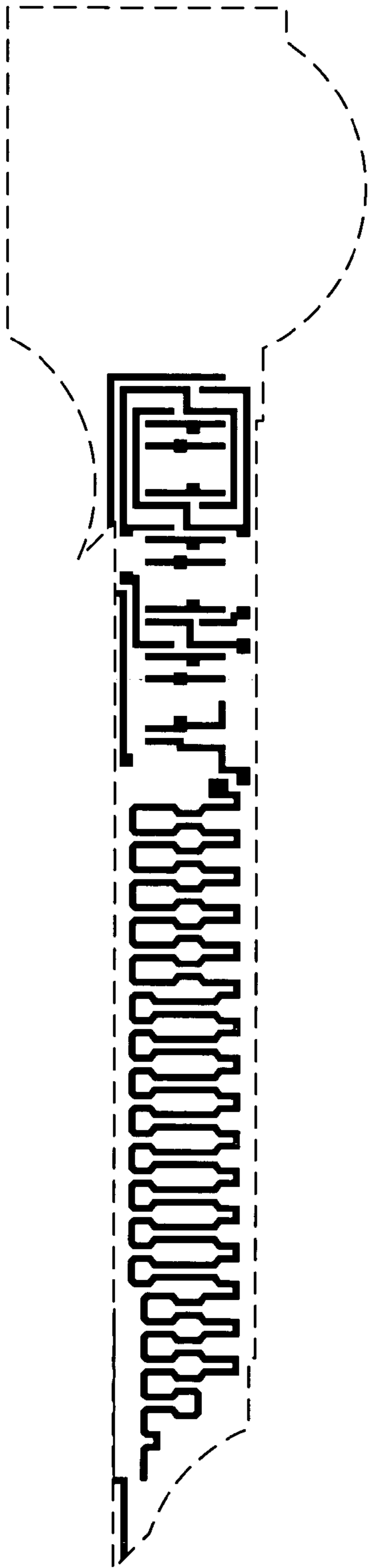
Poly mask
