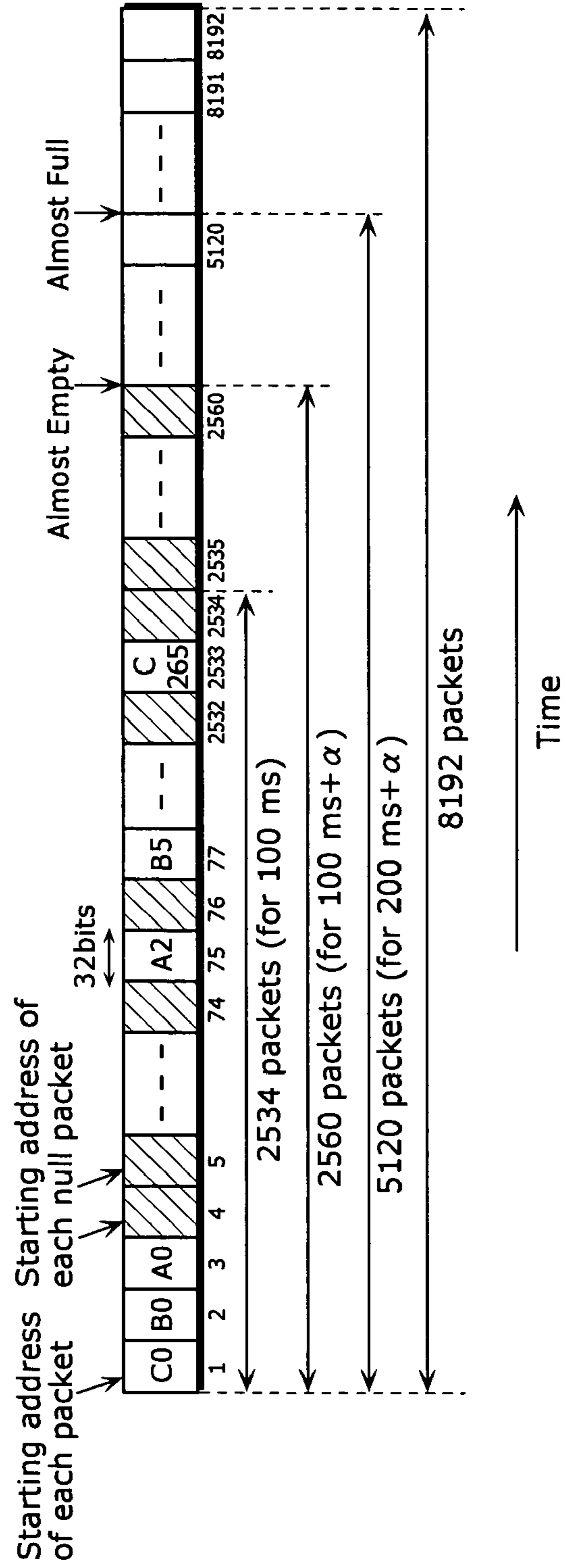
FIG. 9B
