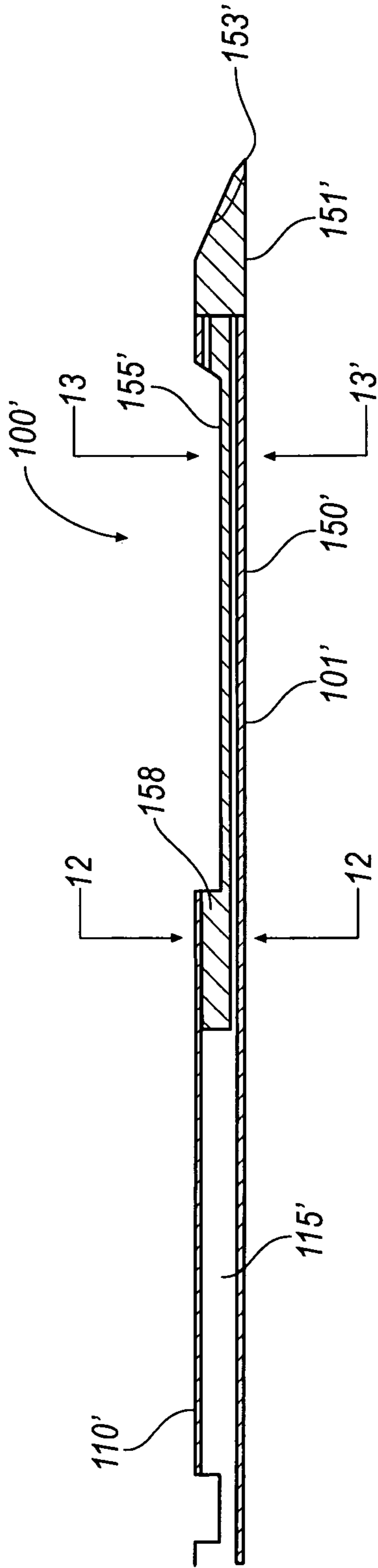
FIG. 11
