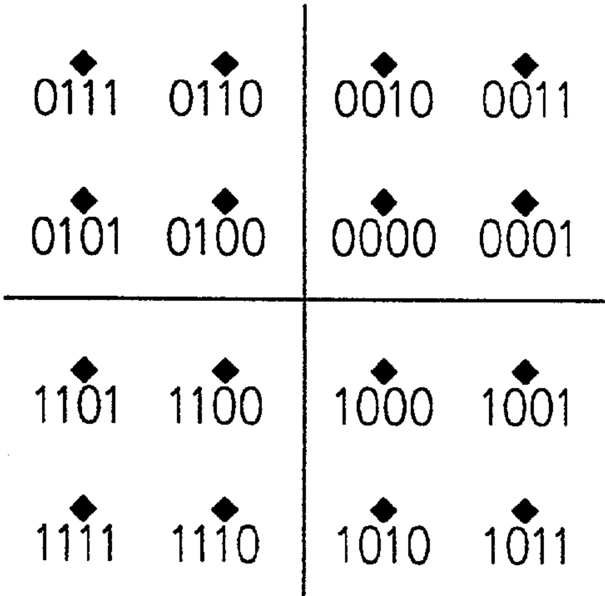
FIG. 12c 4 BITS PER BAUD
