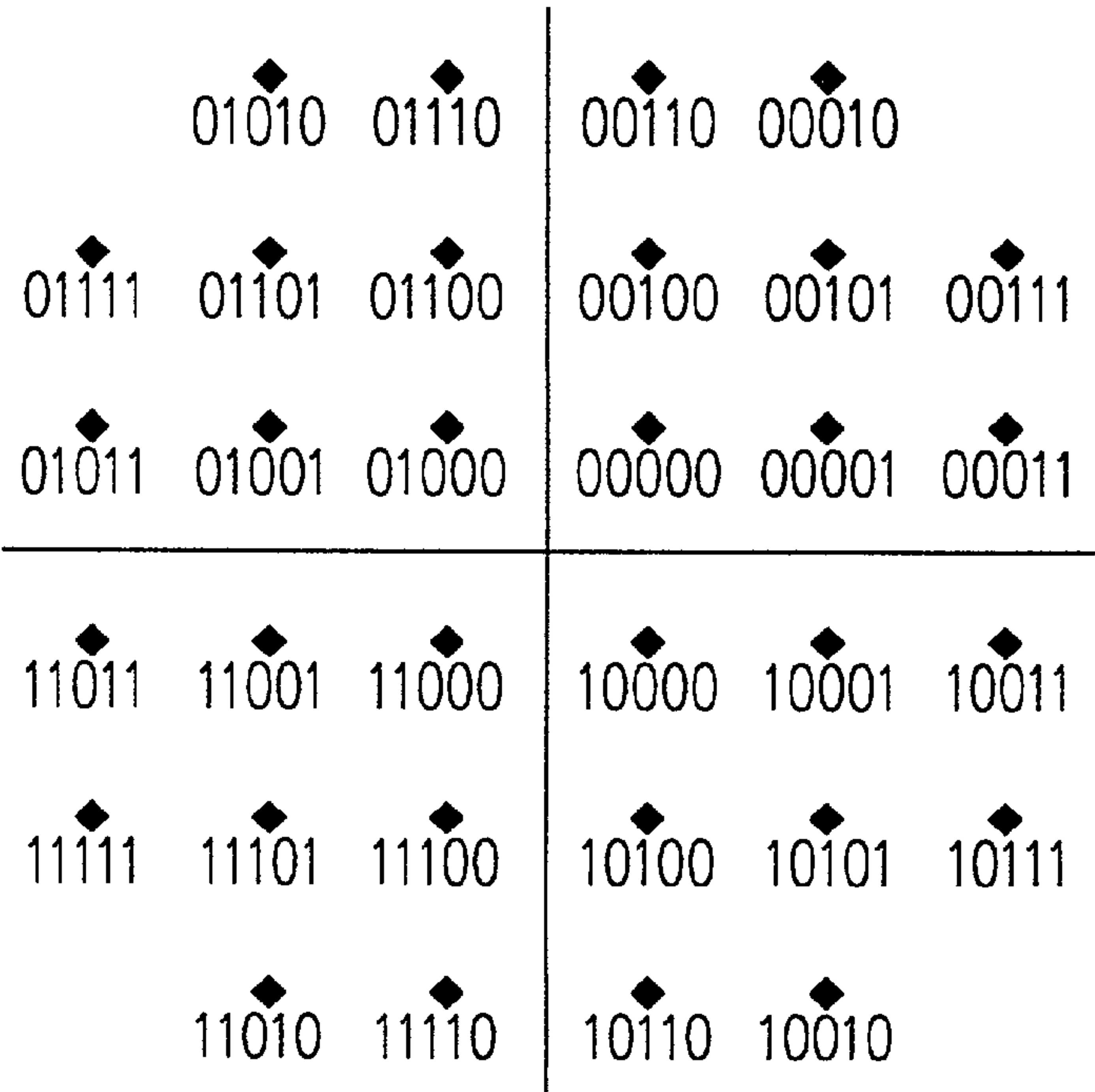
FIG. 12d 5 BITS PER BAUD
