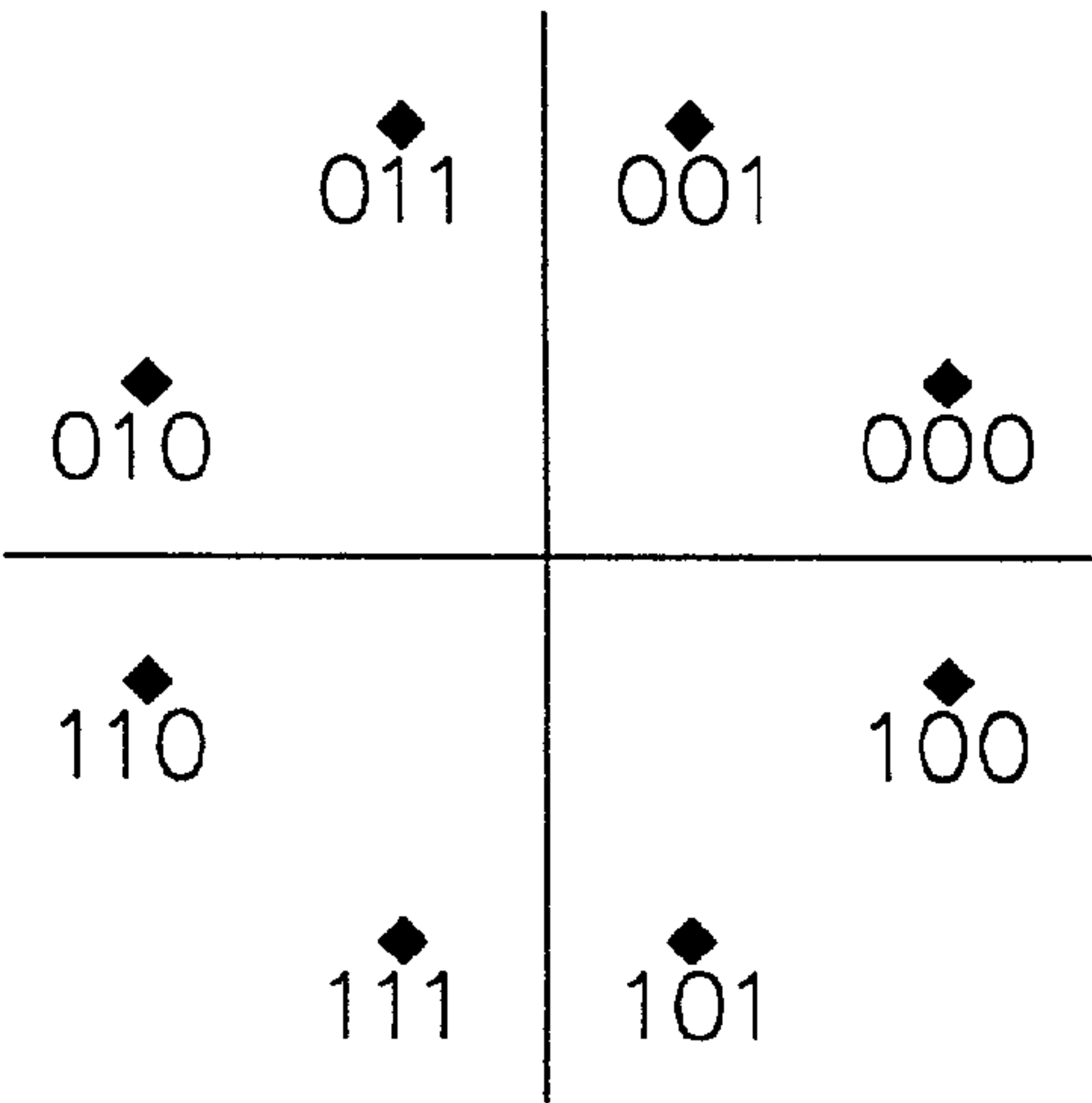
FIG. 12b 3 BITS PER BAUD
