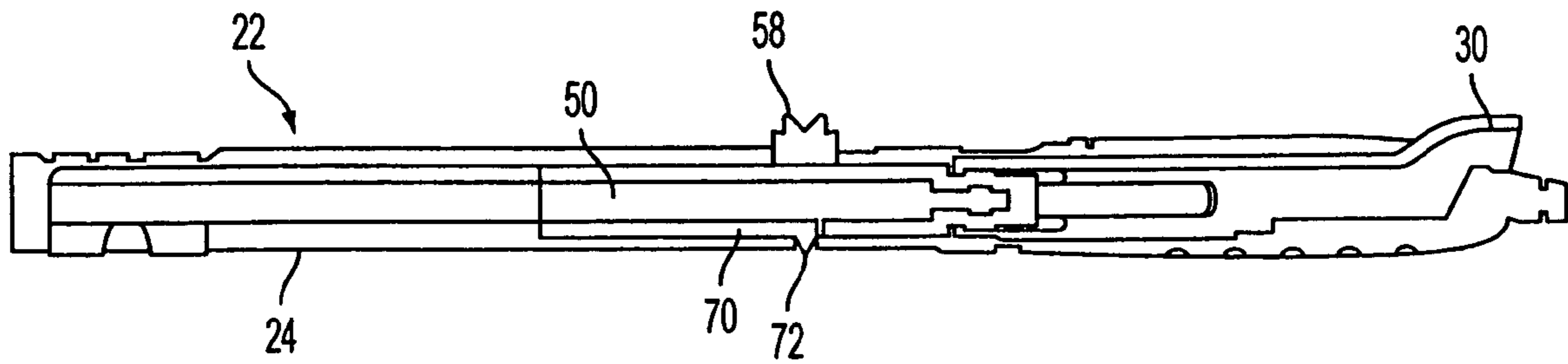
FIG. 8A
