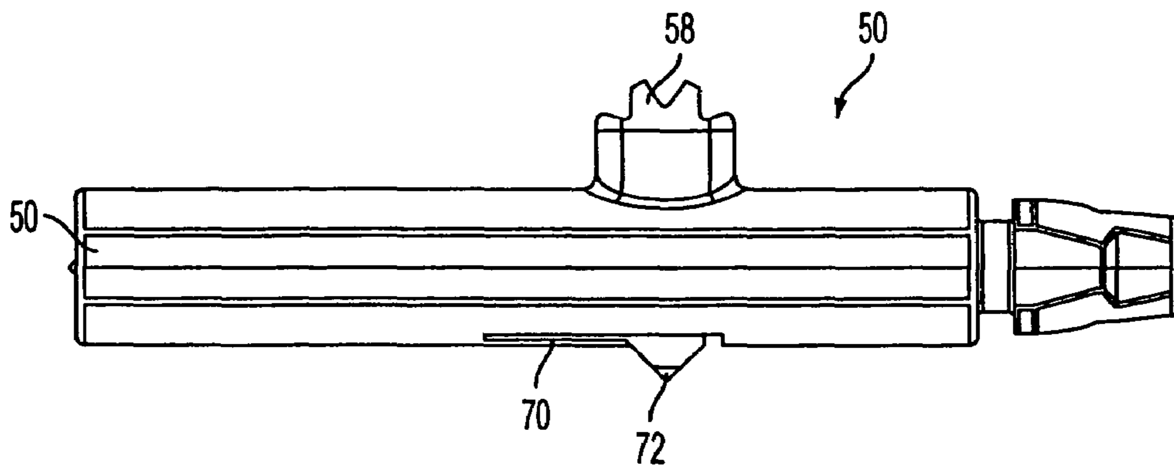
FIG. 8D
