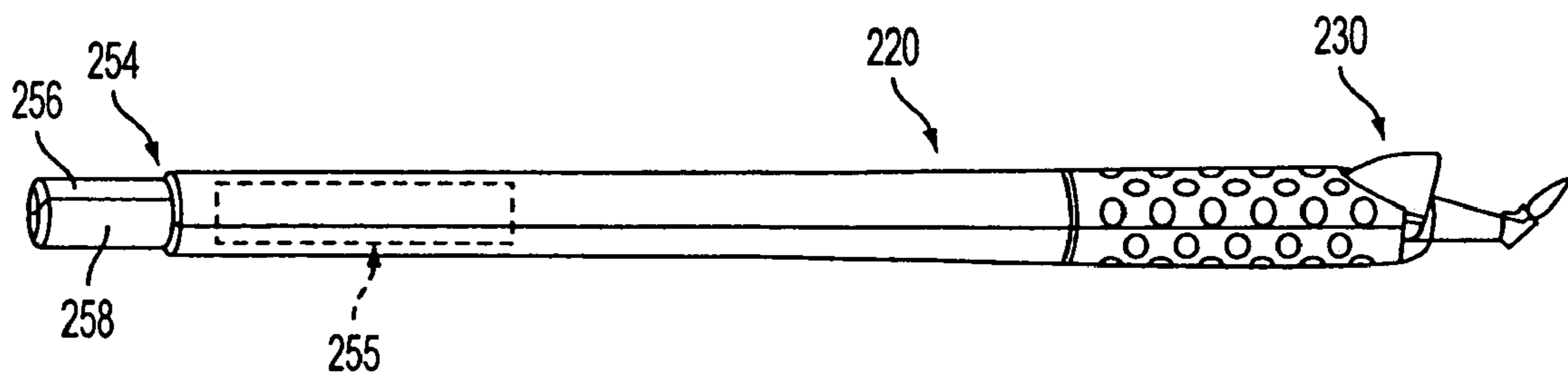
FIG. 12C
