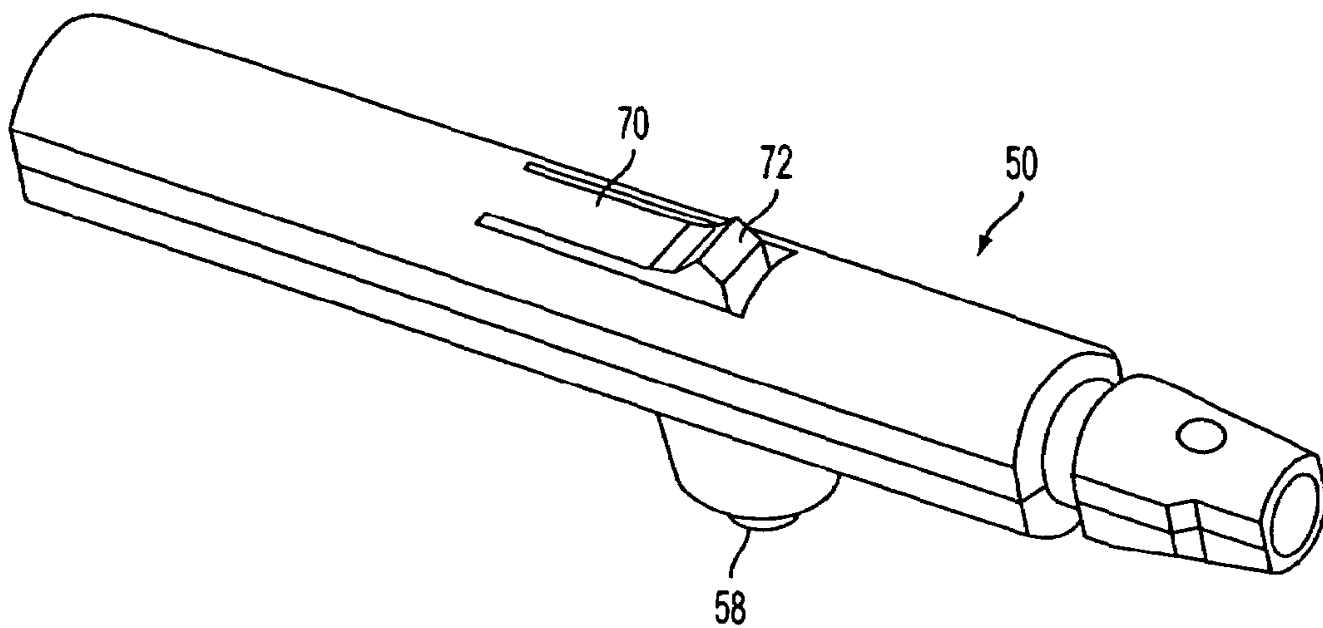
FIG. 8F
