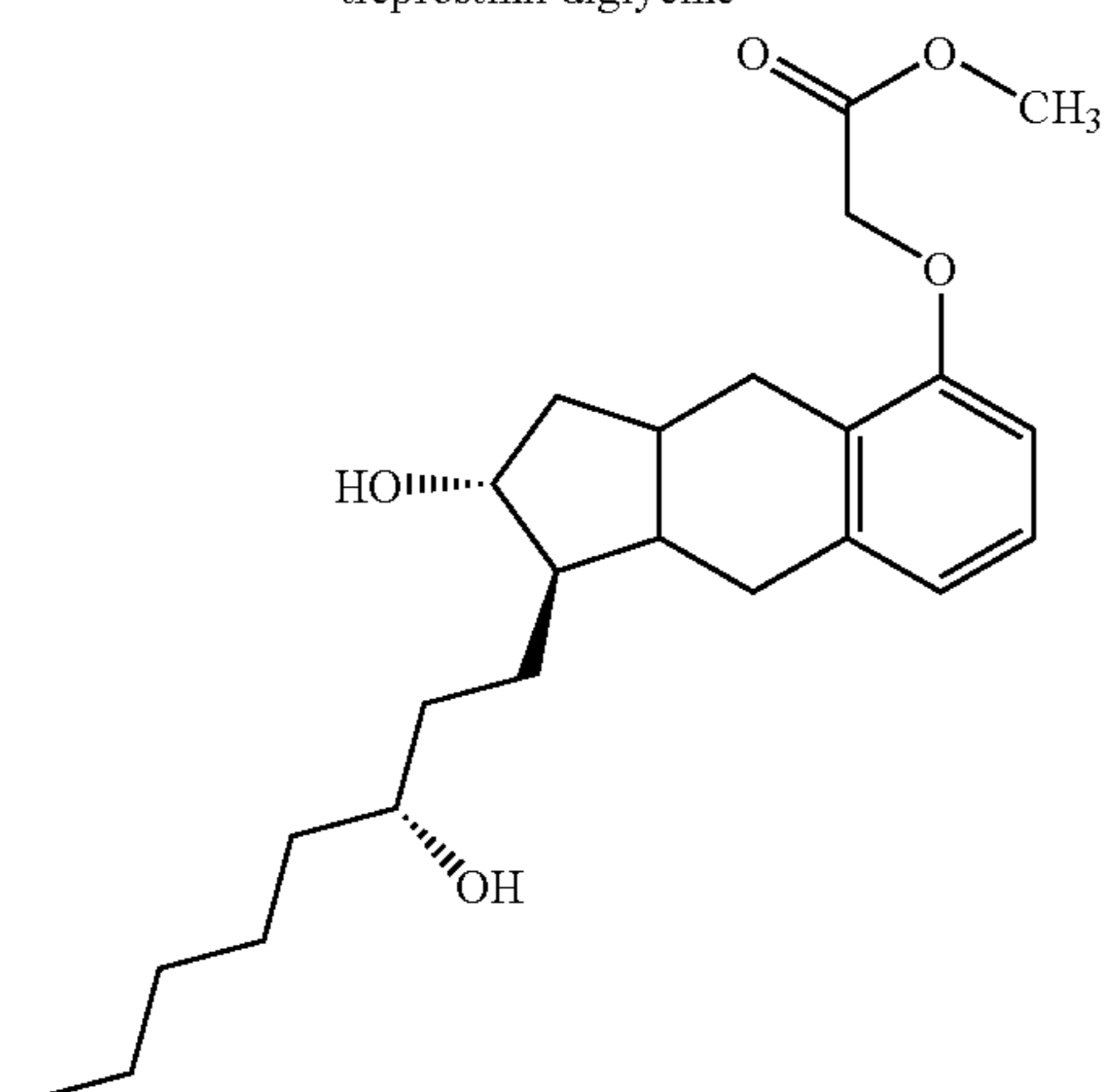
treprostnil methyl ester
