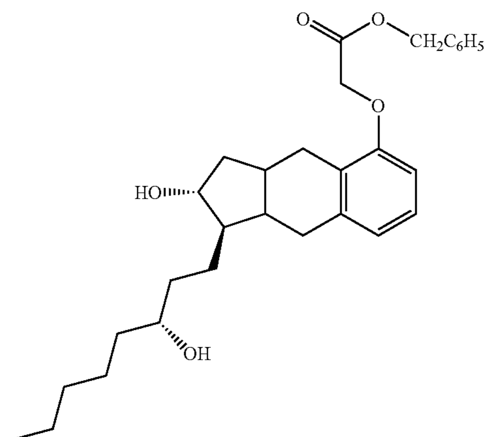
treprostnil benzyl ester
