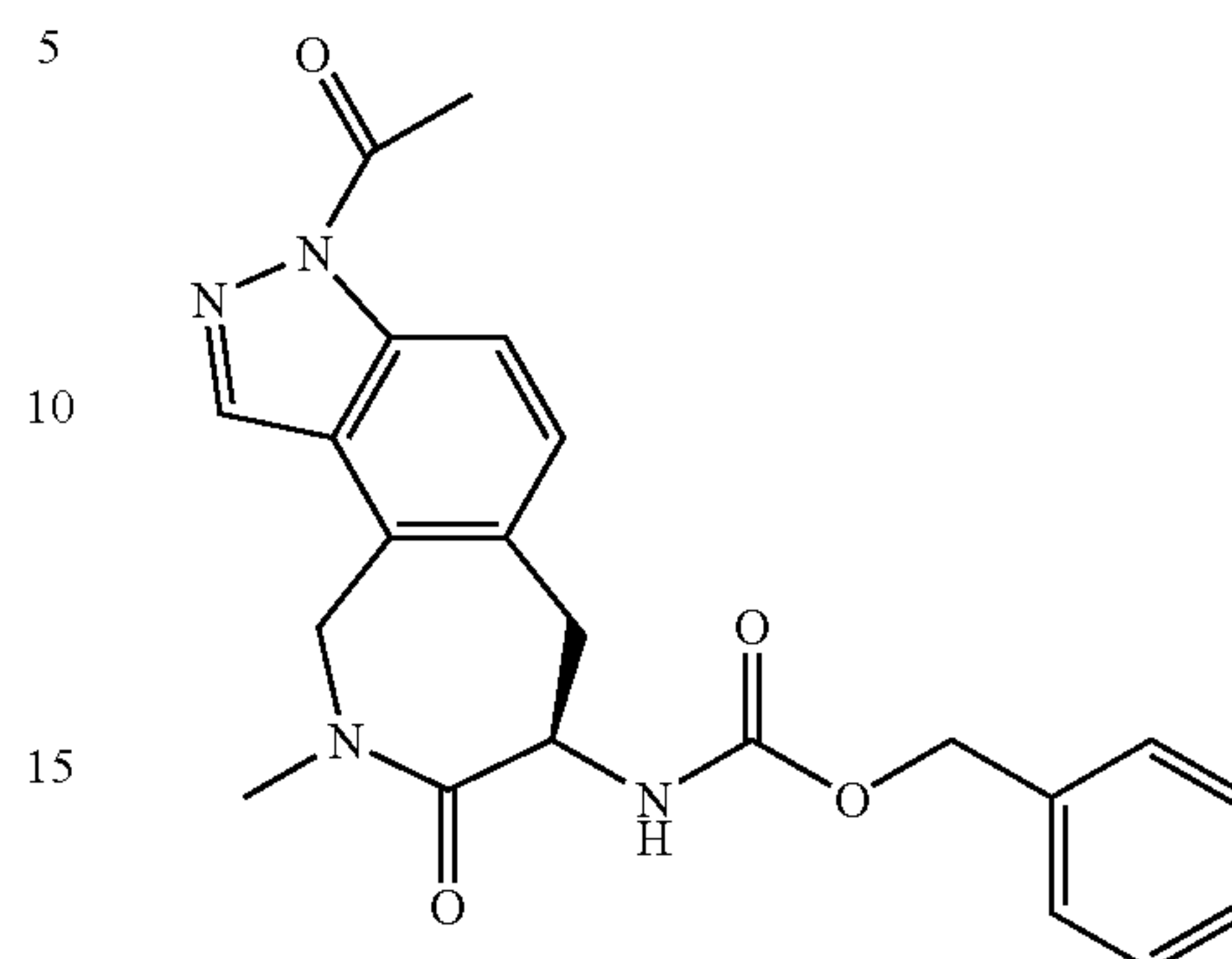
20
