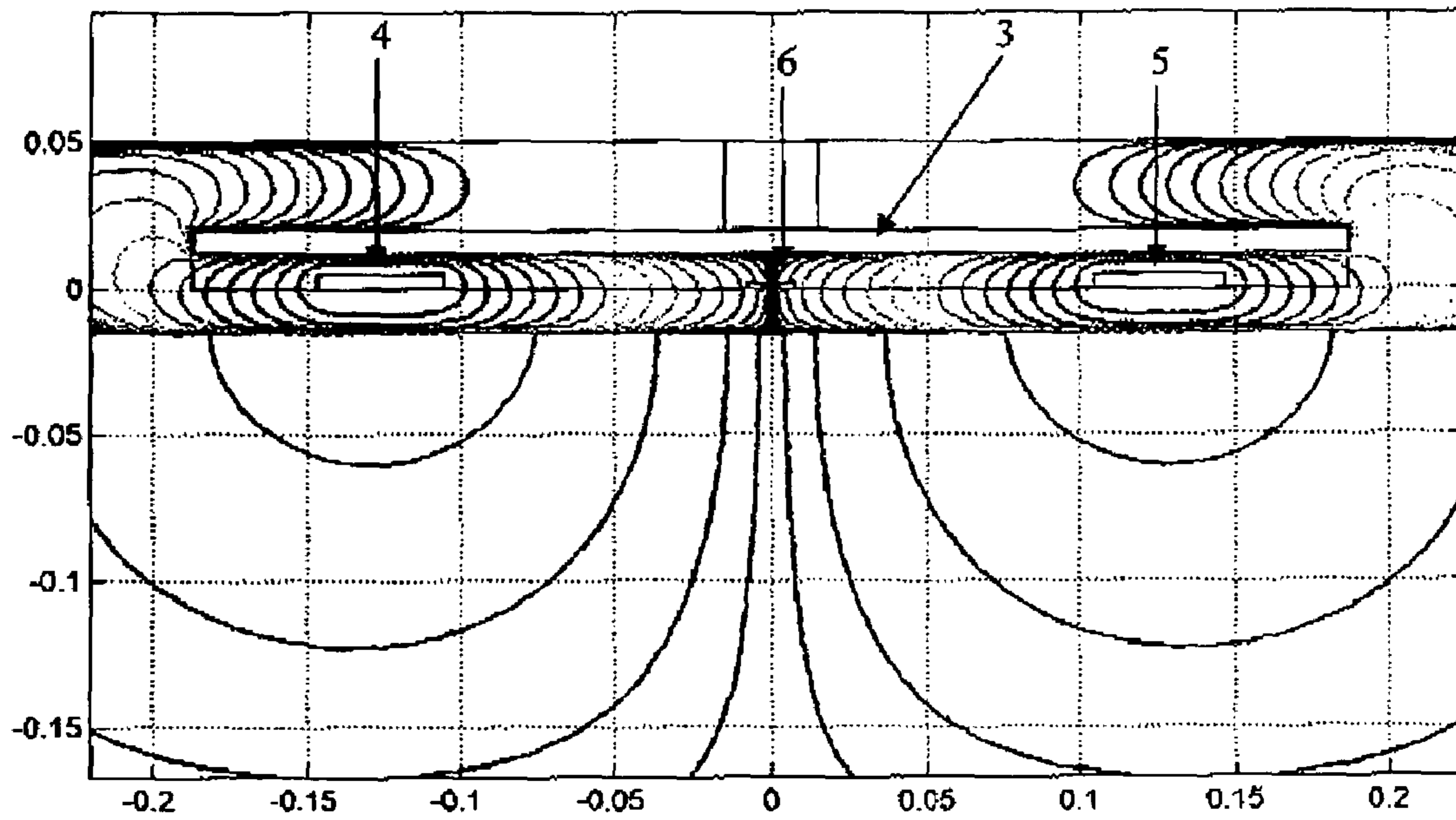
--Prior Art--
