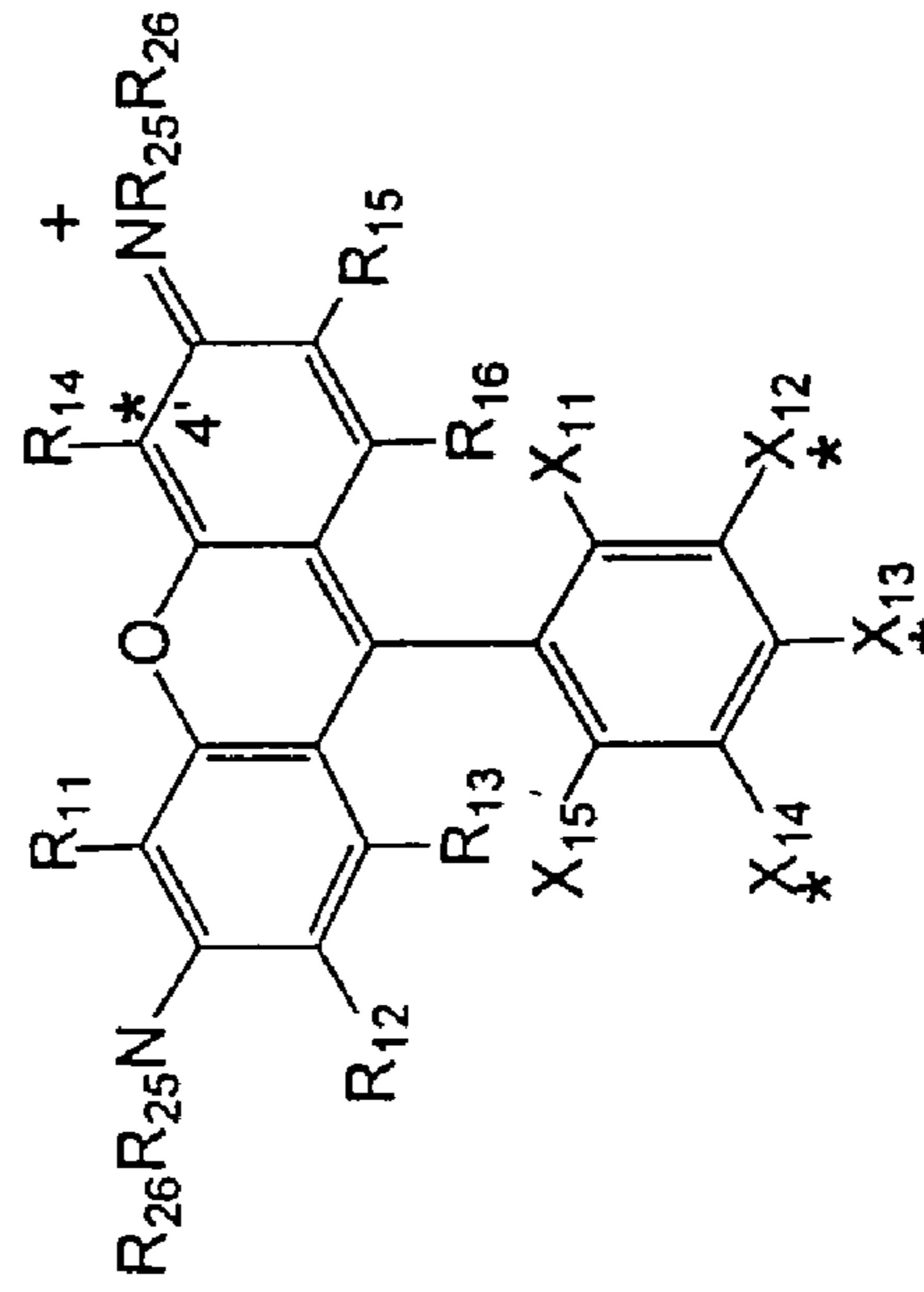
RHODAMINE
