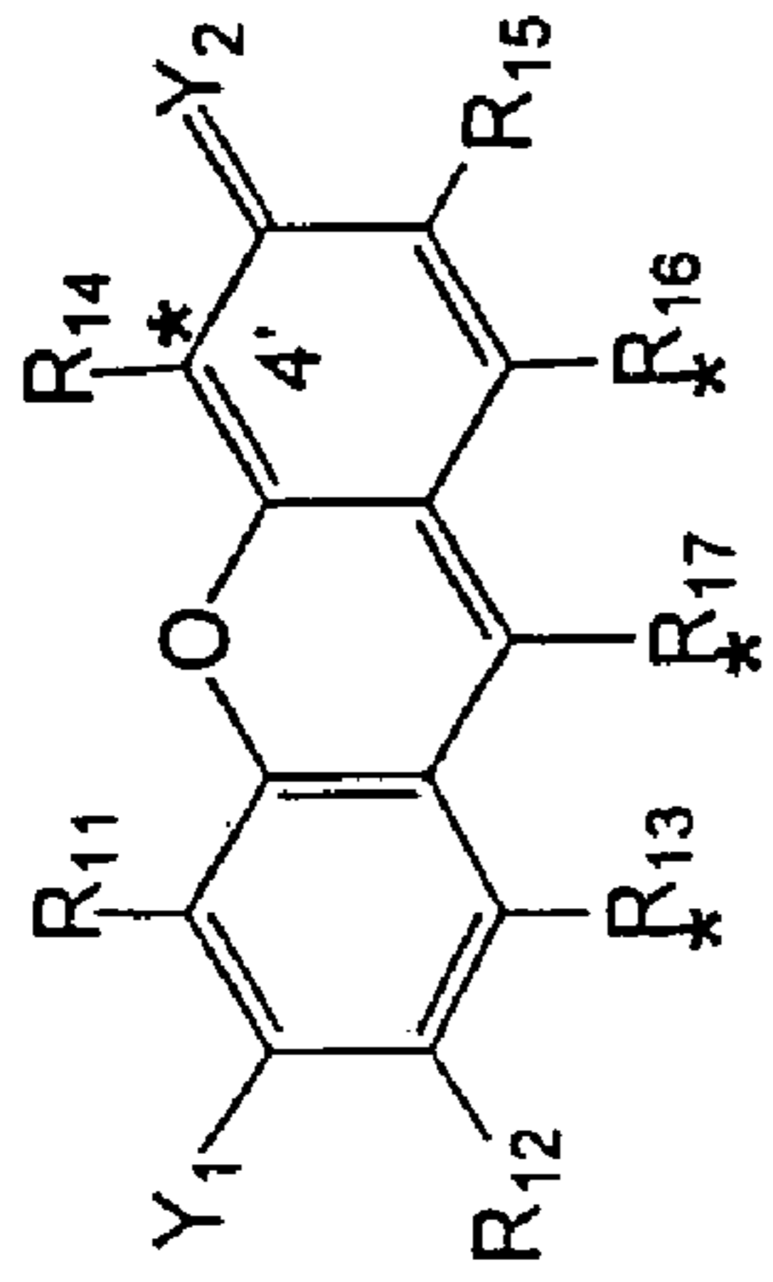
XANTHENE
