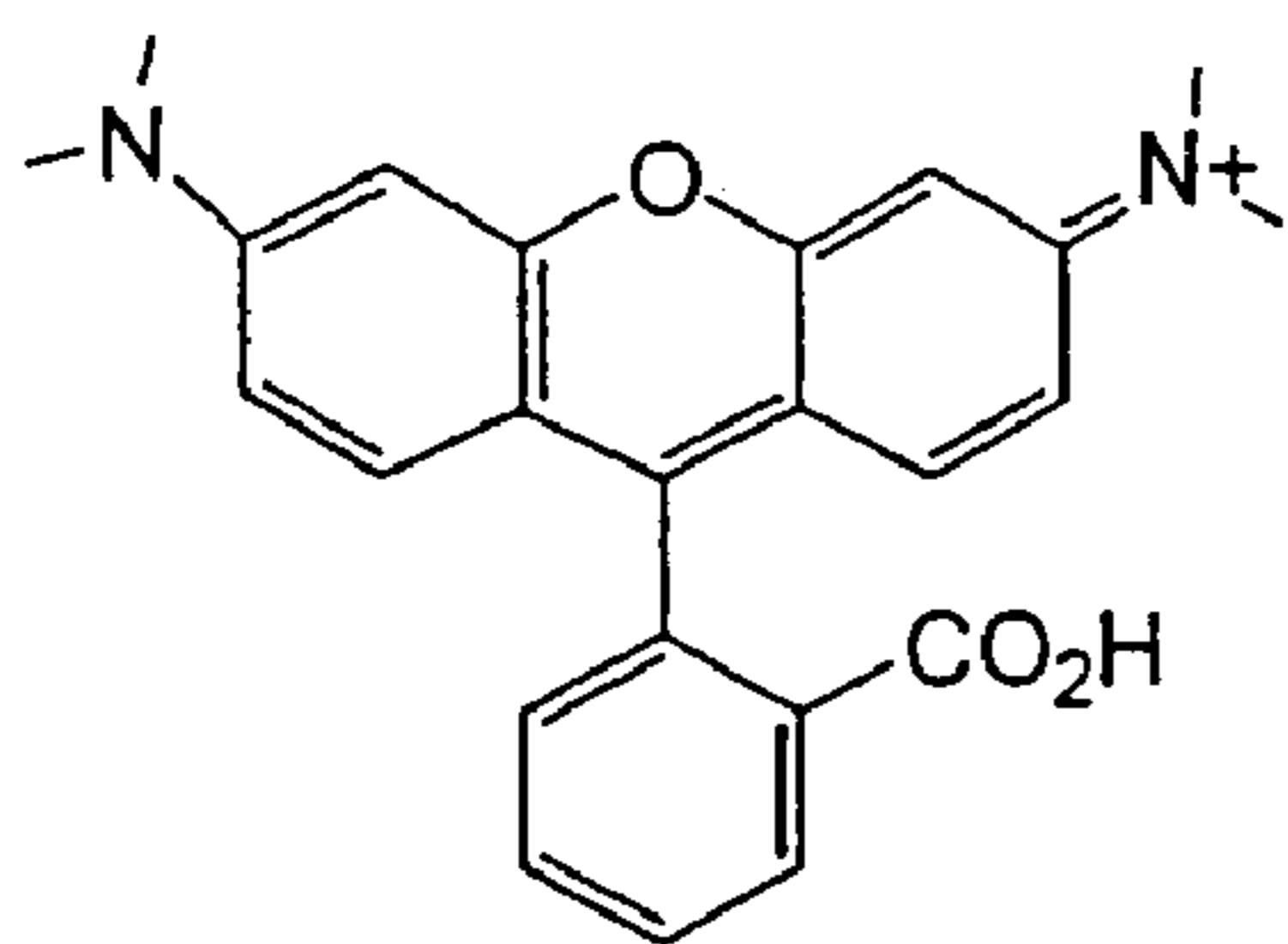
Rhodamine
