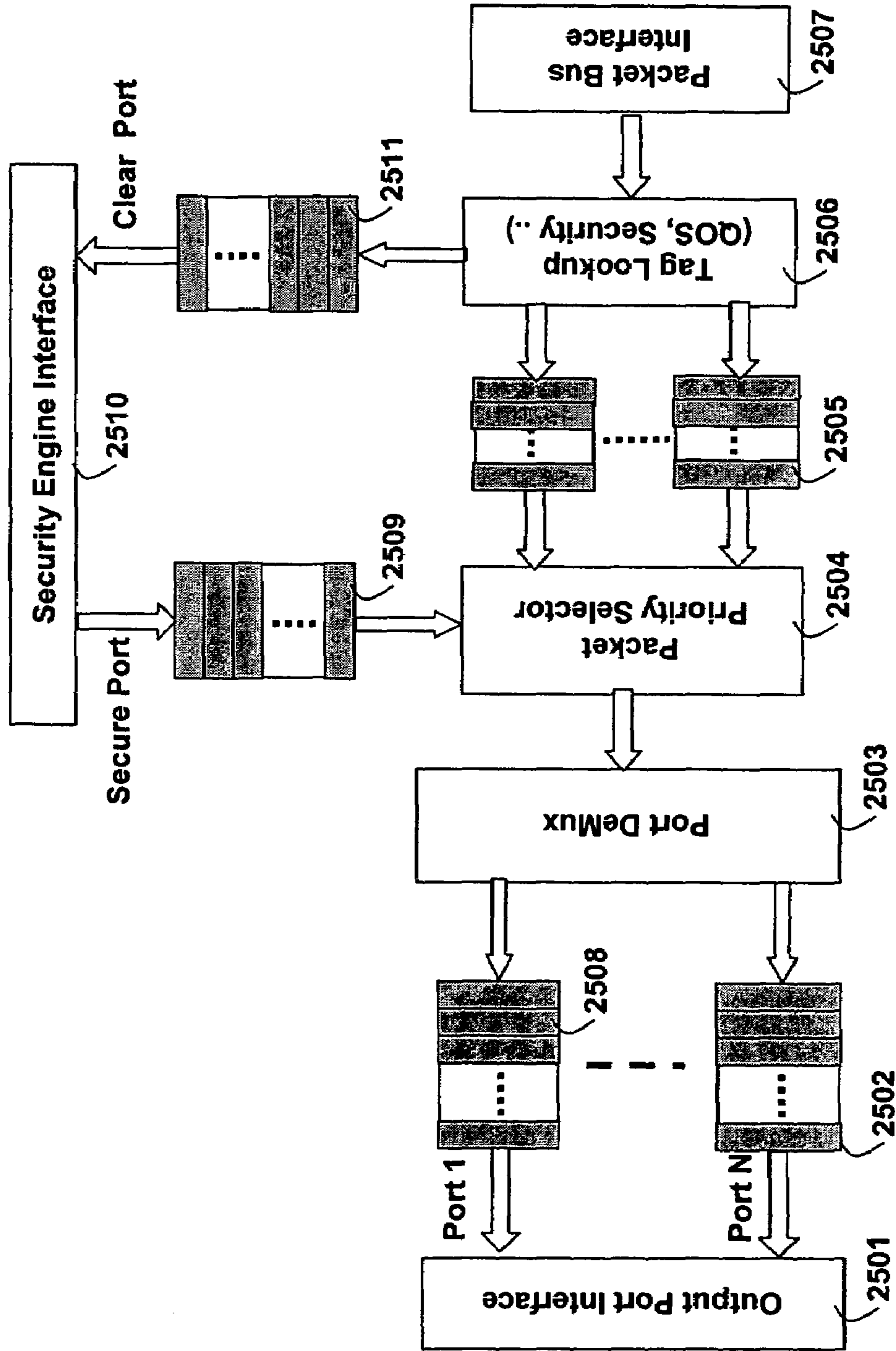
Fig. 25 Output Queue
