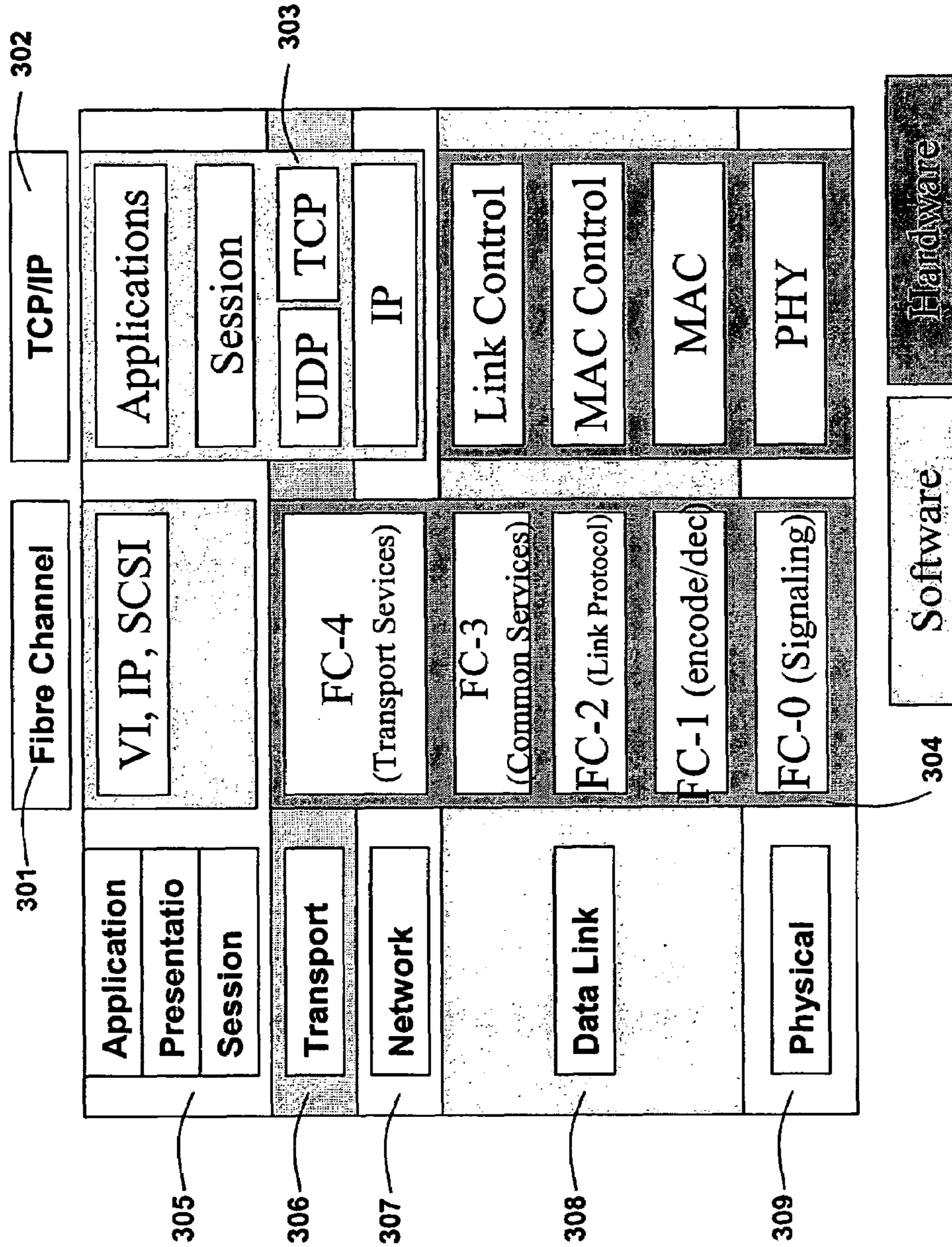
Fig. 3 OSI Stack
