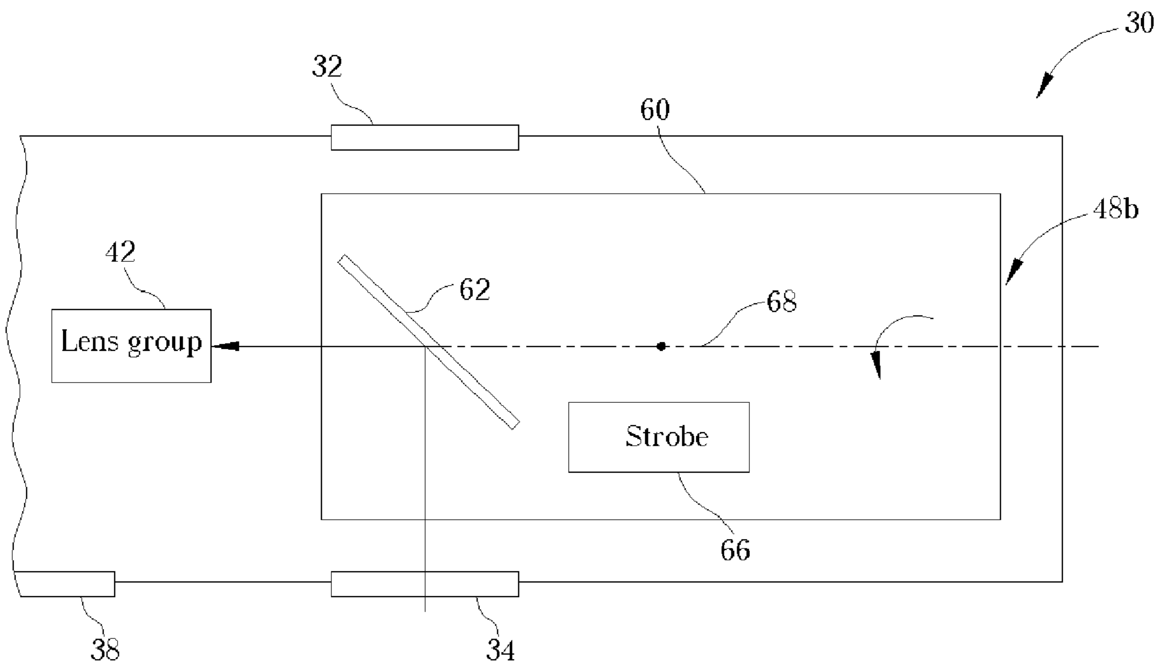
Fig. 10
