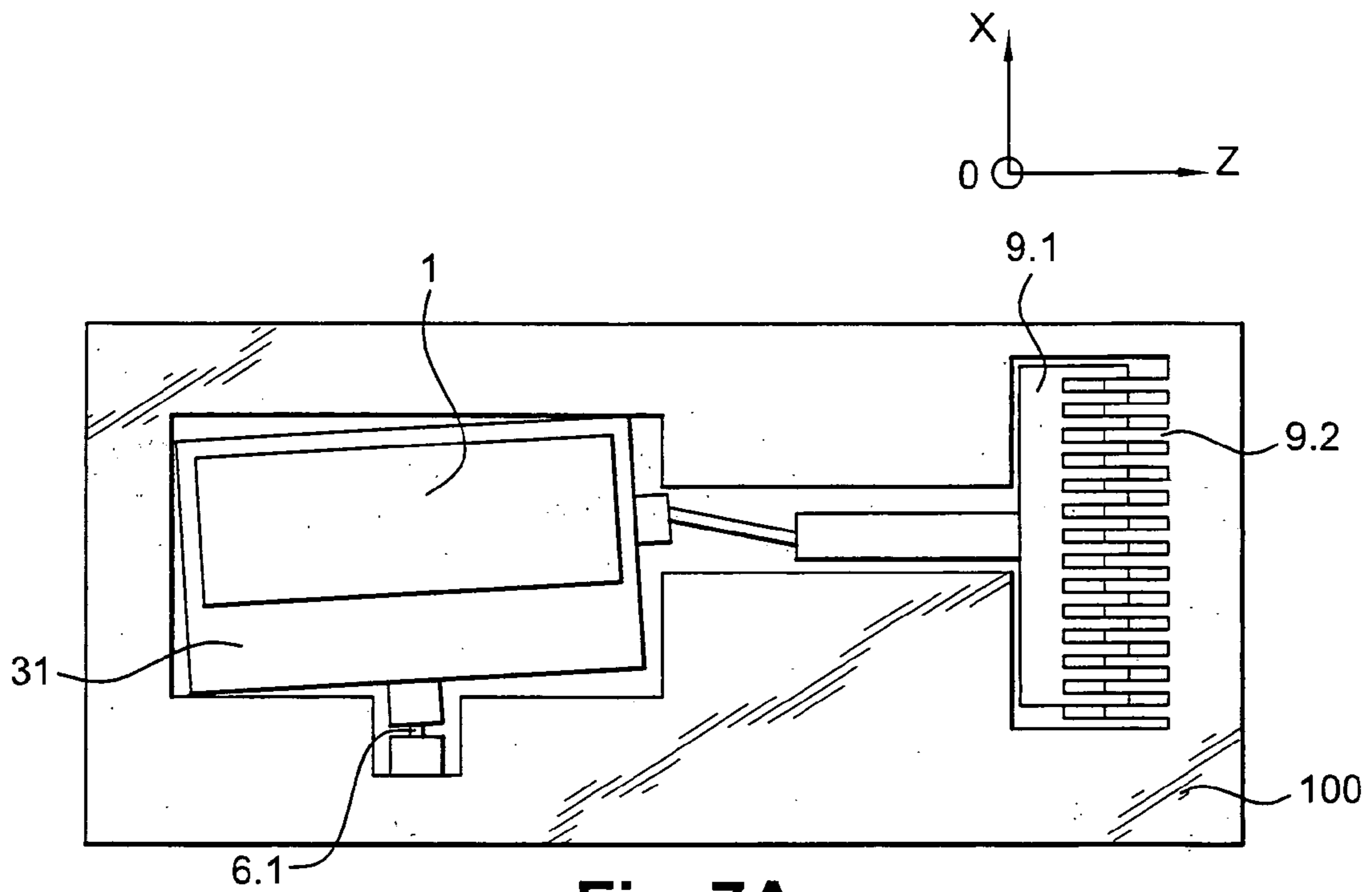
Fig. 7A
