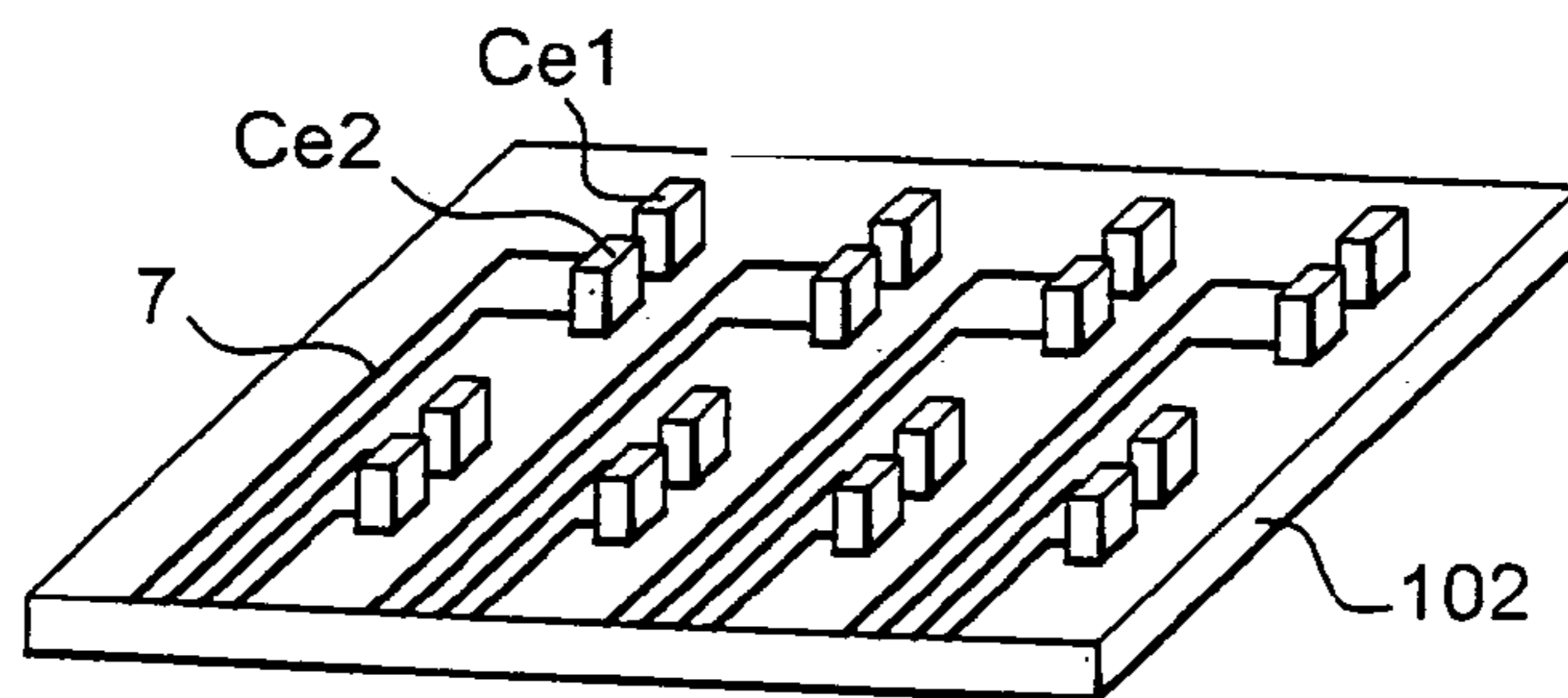
Fig. 4B
