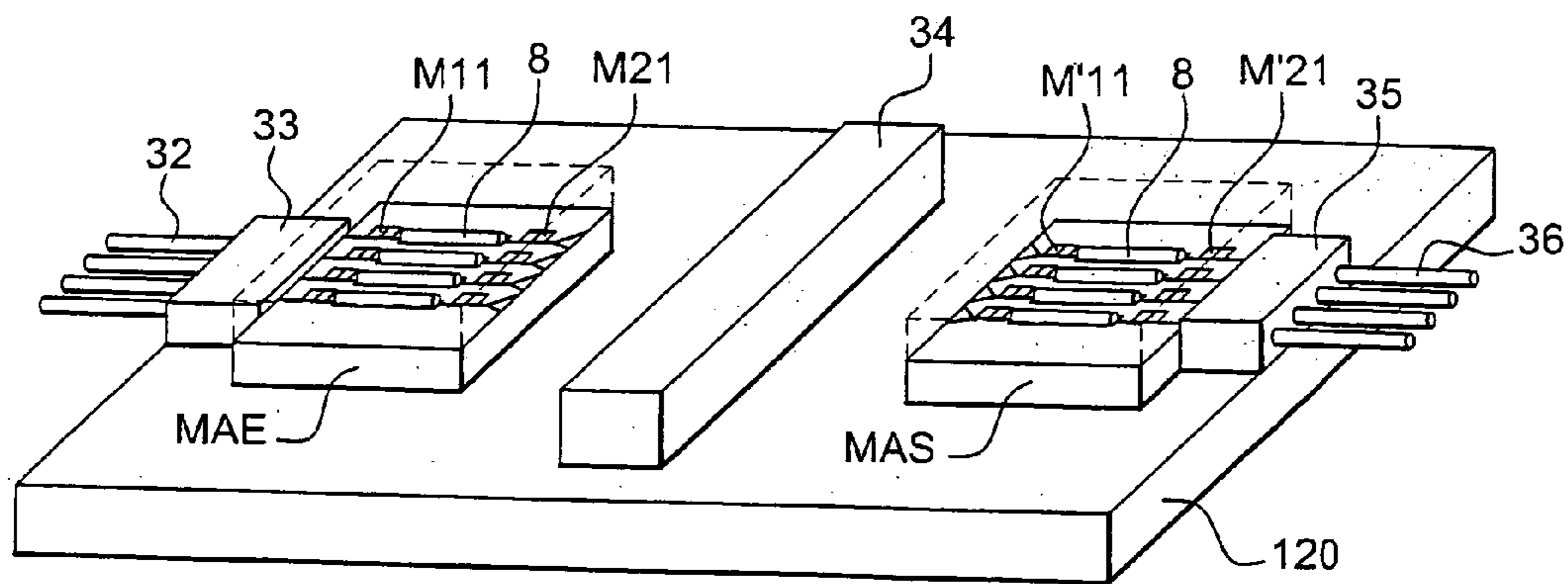
Fig. 3C
