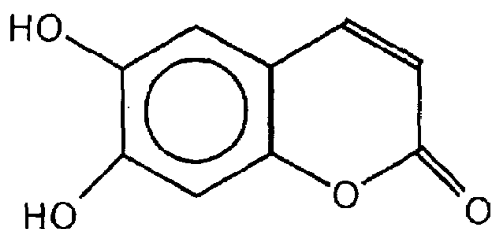
Esculetin
