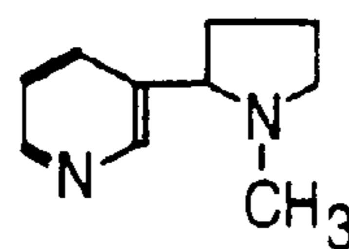
Nicotine
