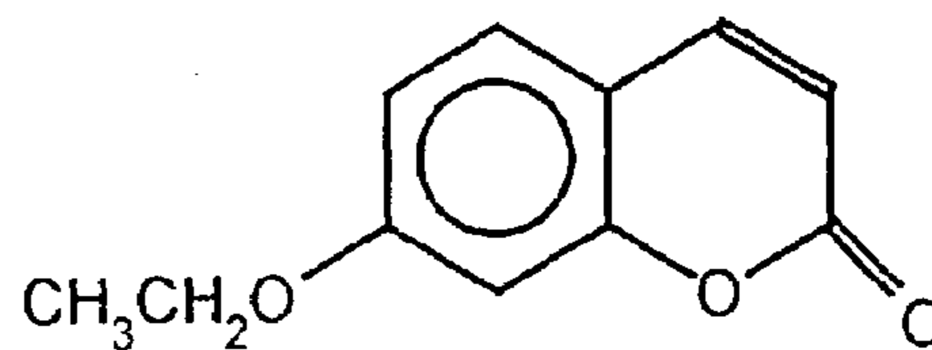
7-Ethoxycoumarin
