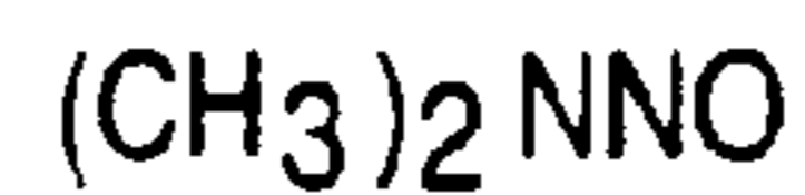
N-Nitrosodimethylamine
