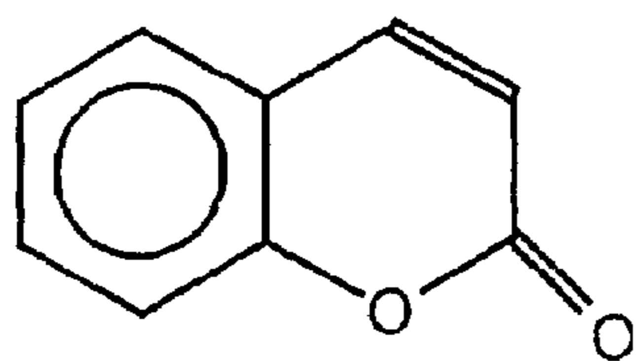
Coumarin
