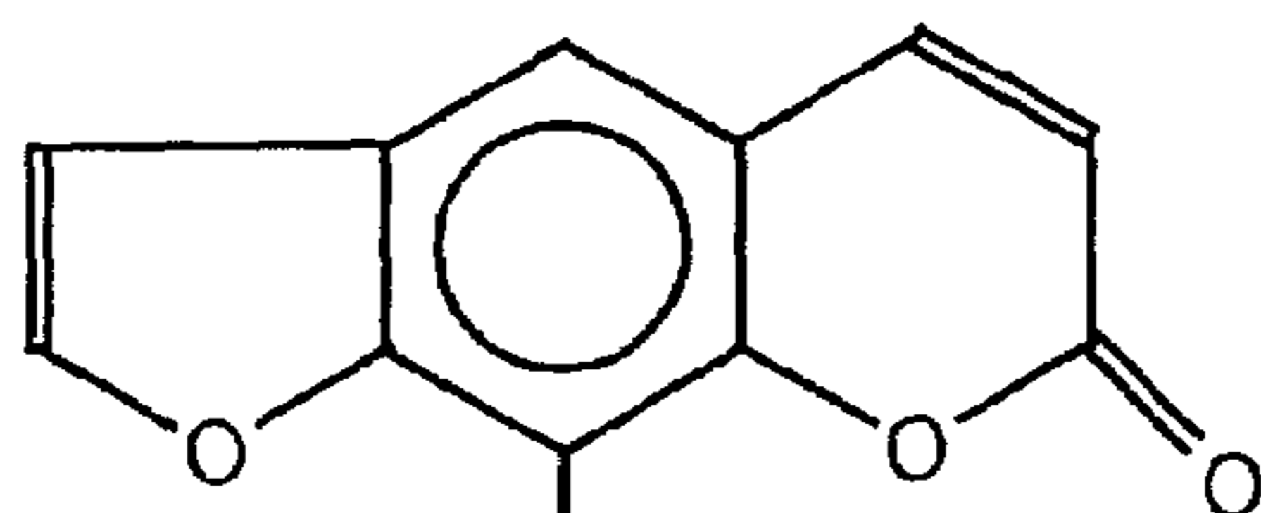
Esculetin
