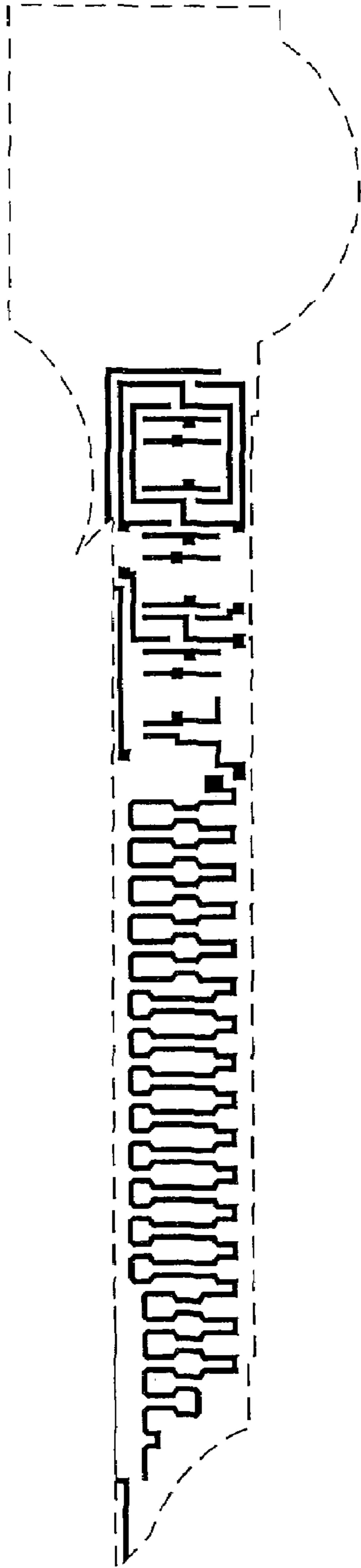
Poly mask
