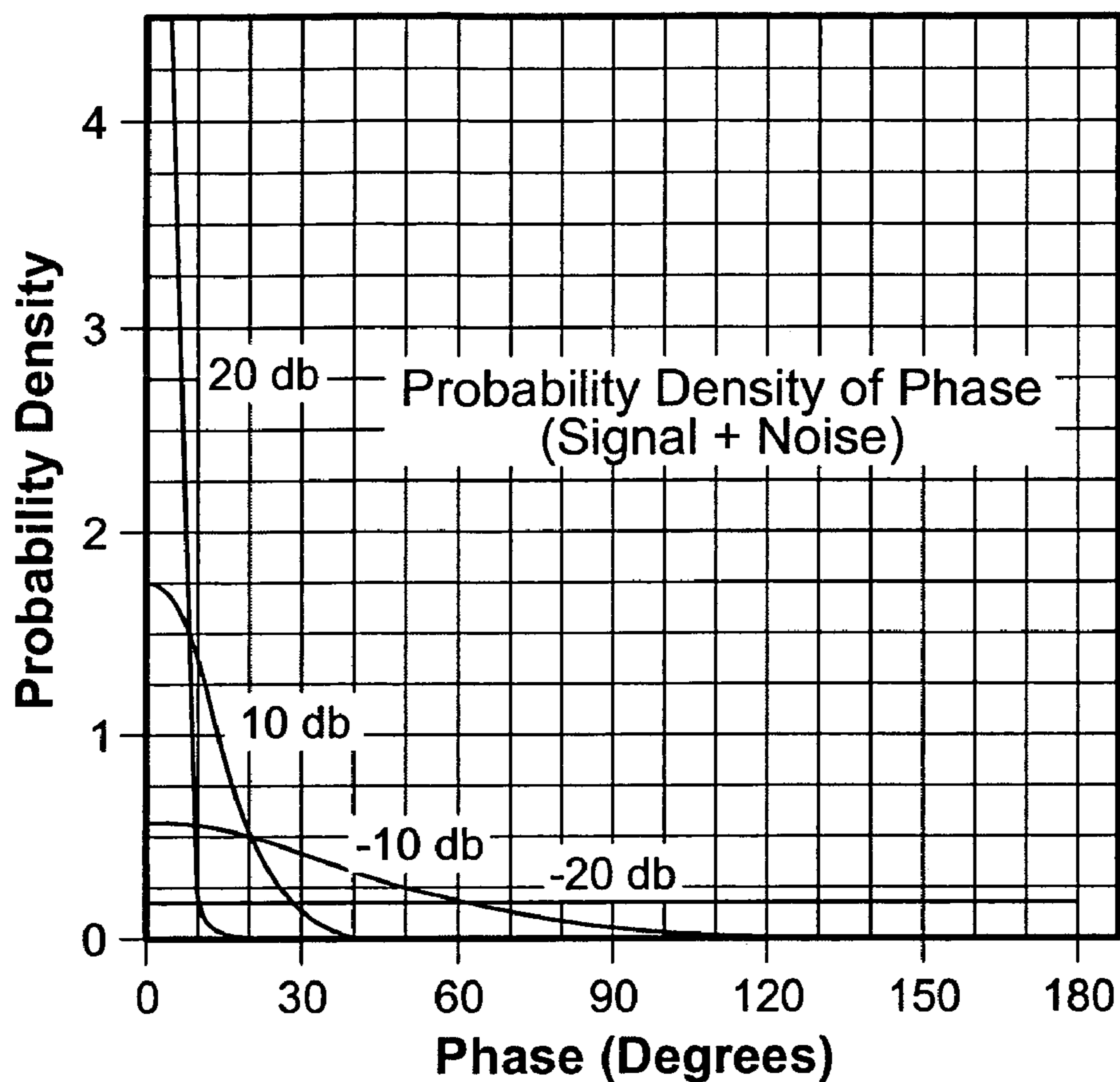
FIG. 9B
