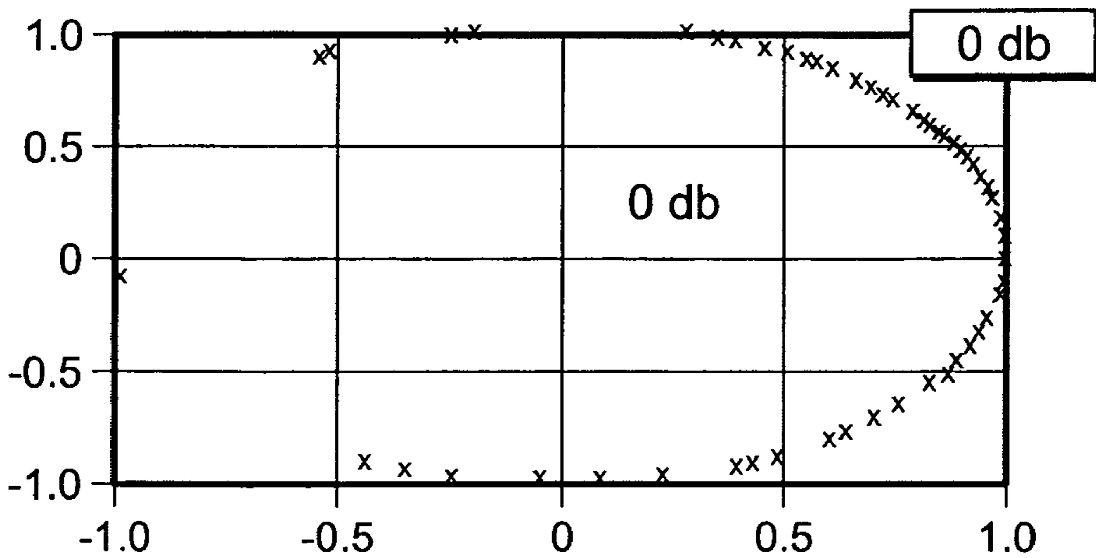
FIG. 9A-2
