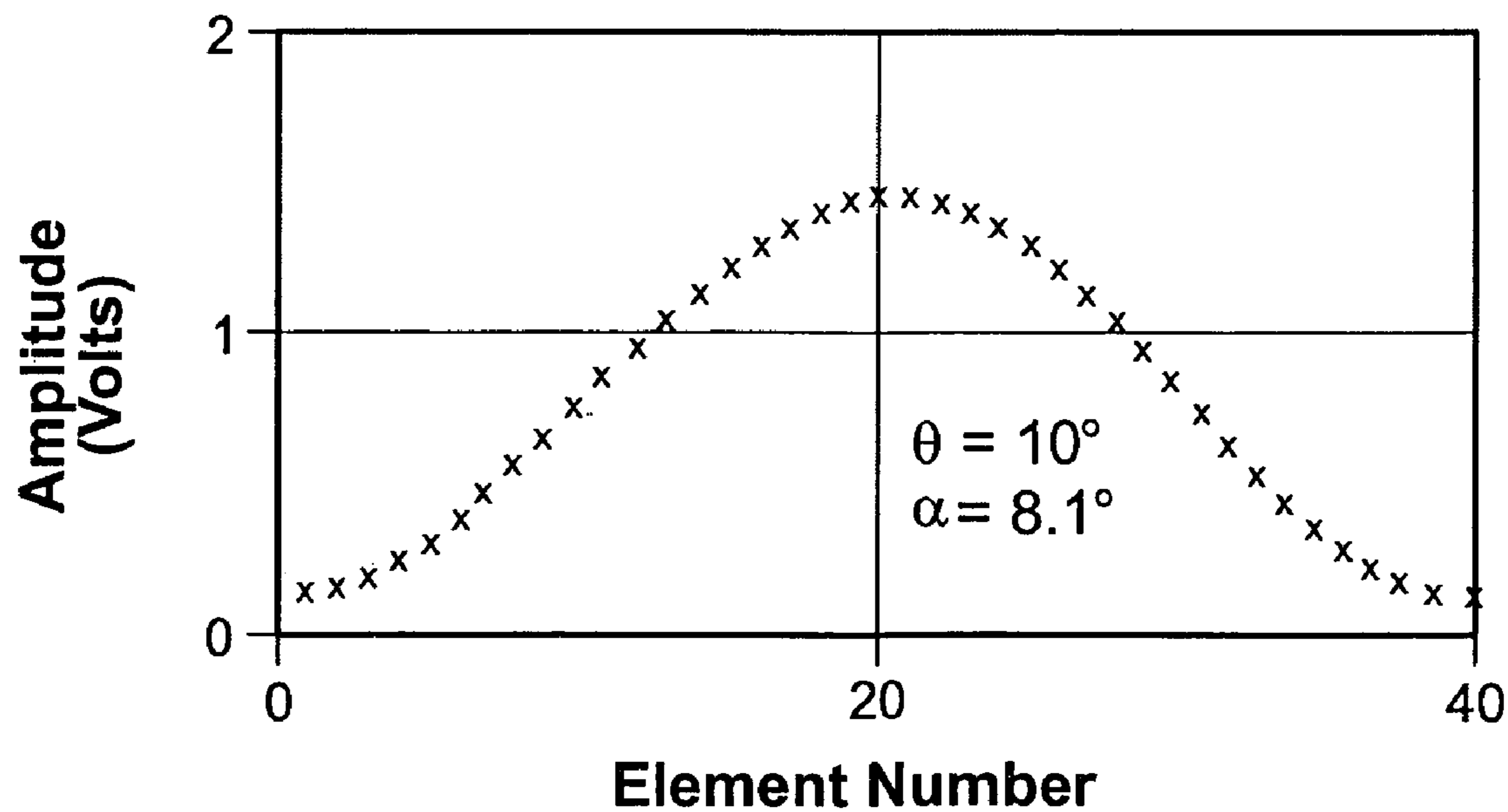
FIG. 7B
