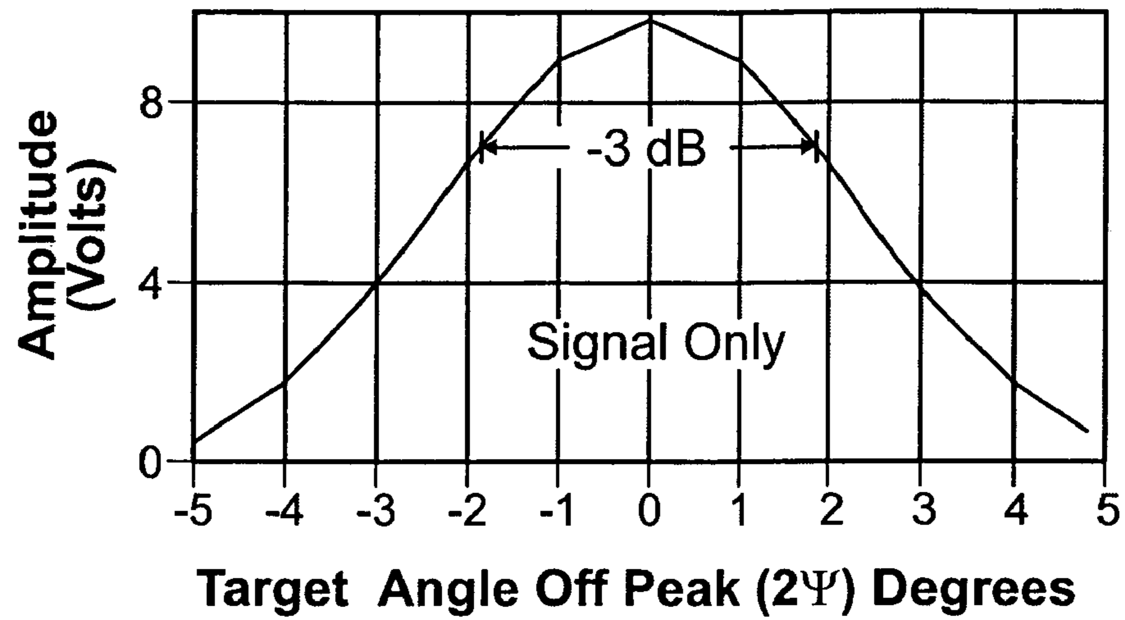
FIG. 2B
