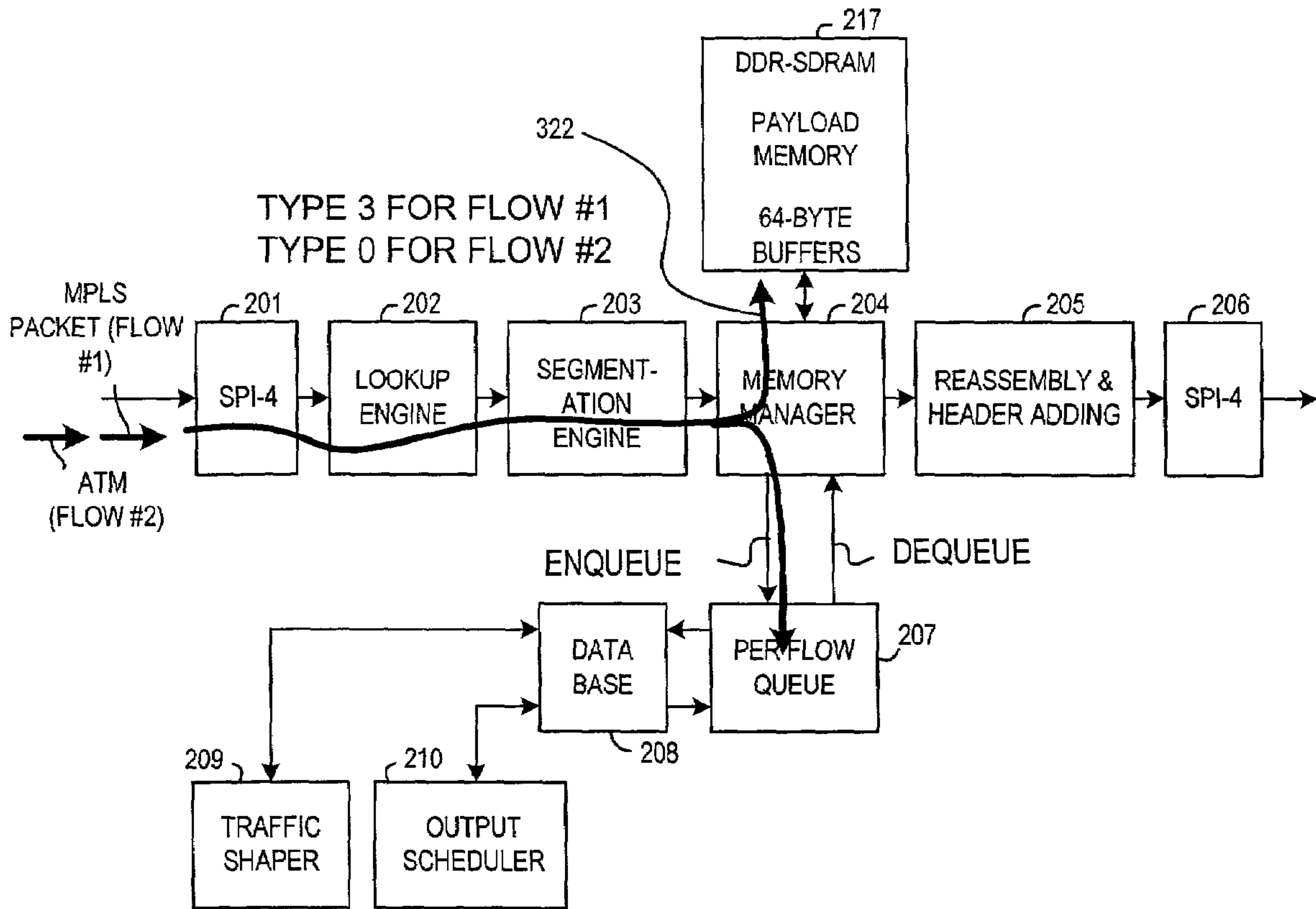
INGRESS MODE
