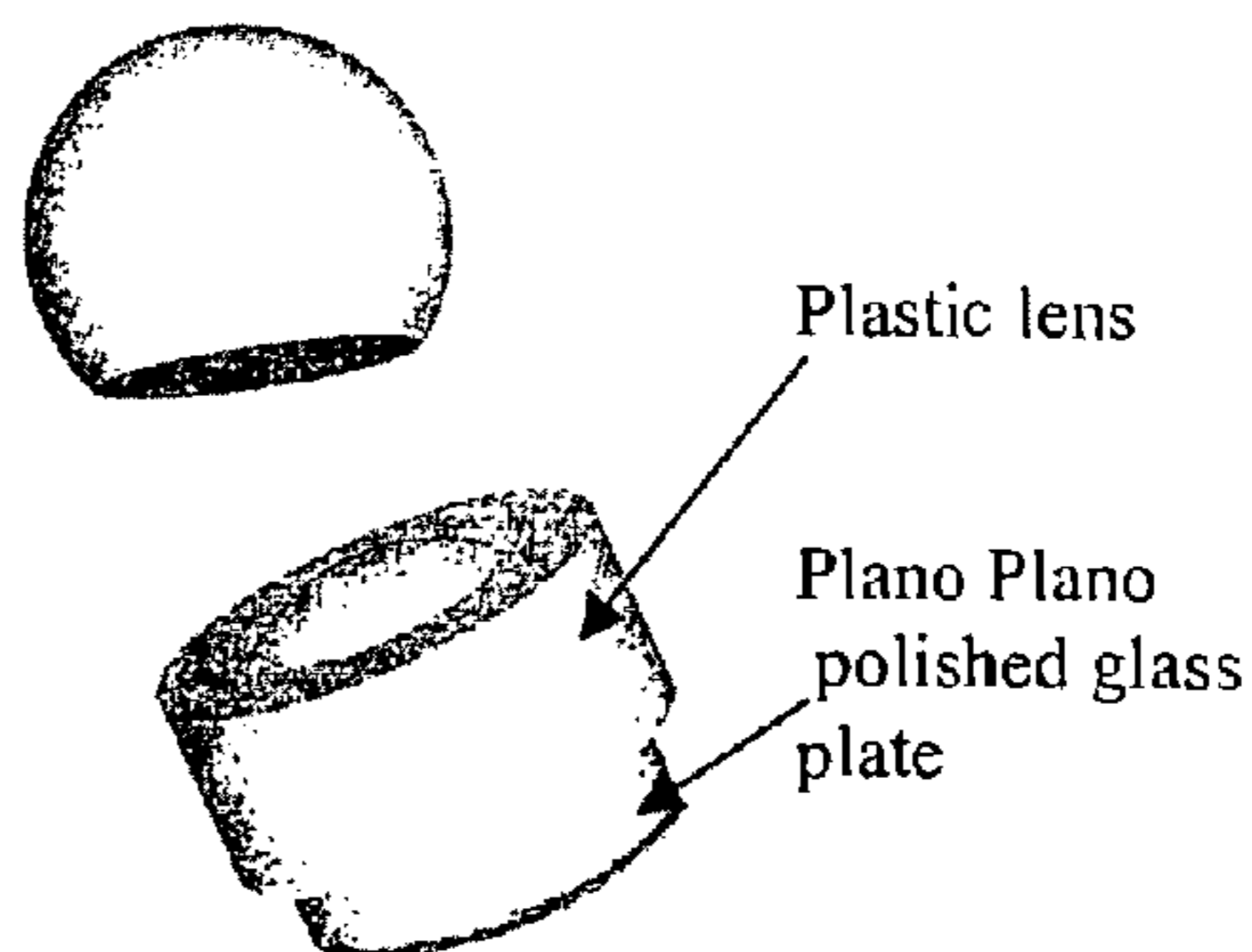
(d) Perspective view of glass holder
