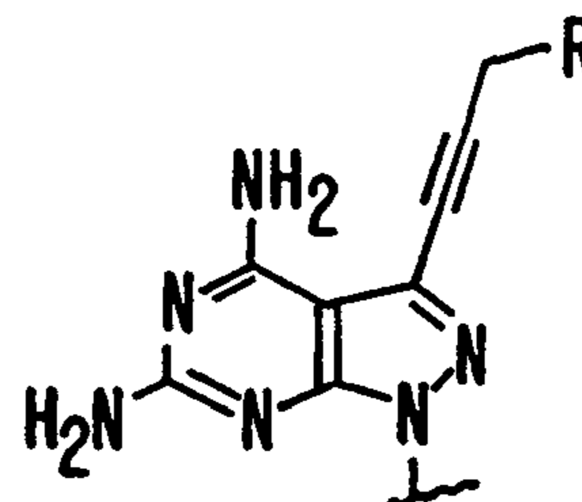
(NH 2 ) 2 PPPAOH R = OH (NH 2 ) 2 PPPA NH 2 R = NH 2
