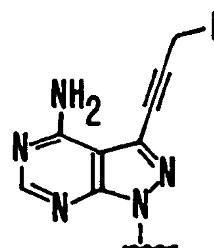
HOPPPA R = OH NH 2 PPPA R = NH 2
