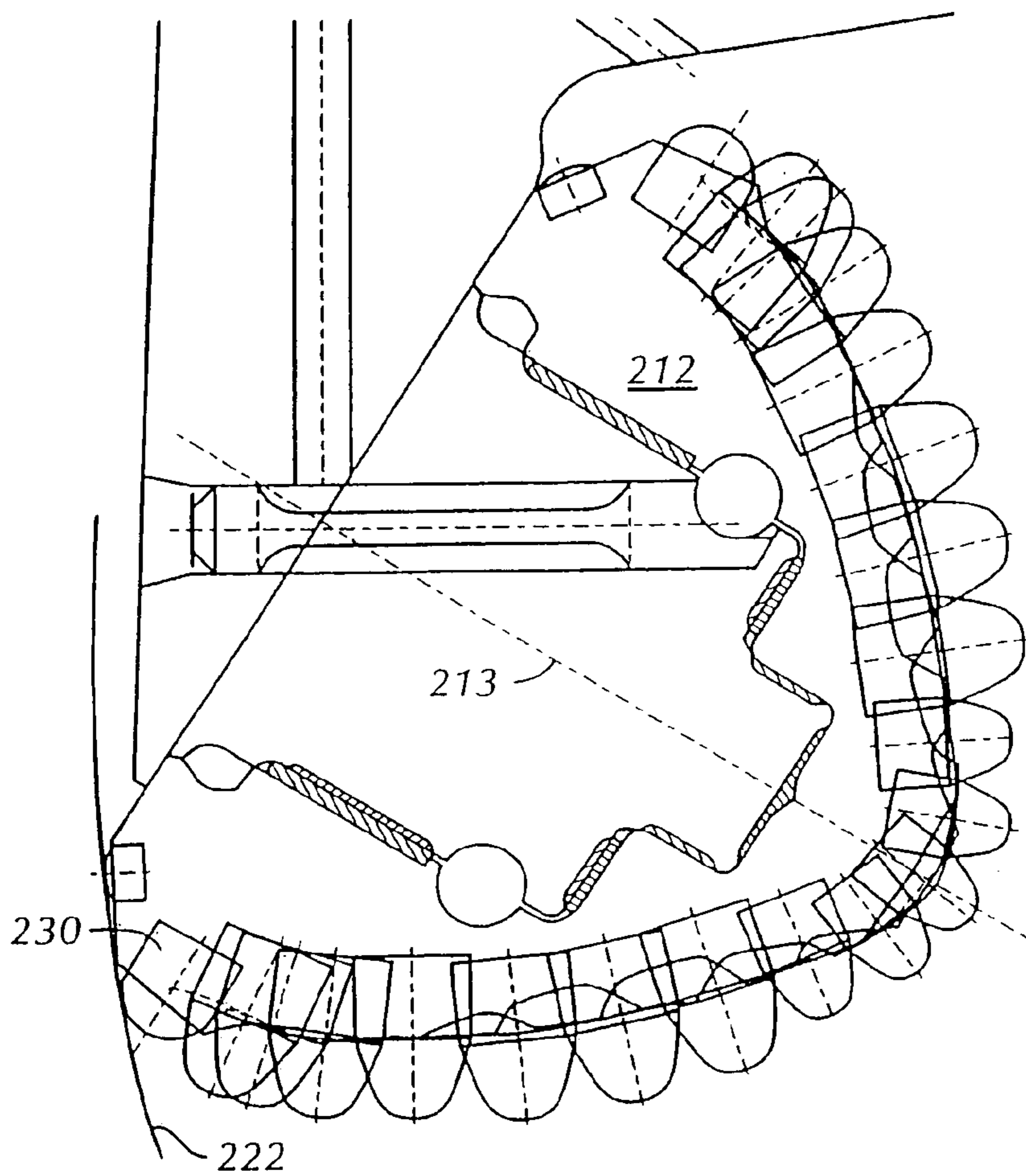
FIG. 20
