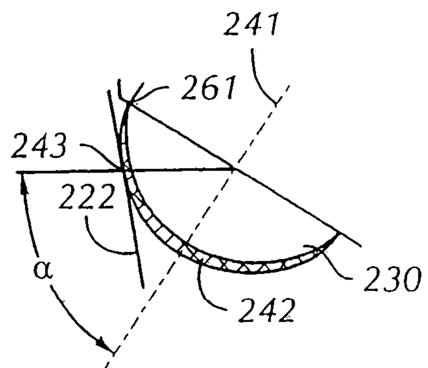
FIG. 15
