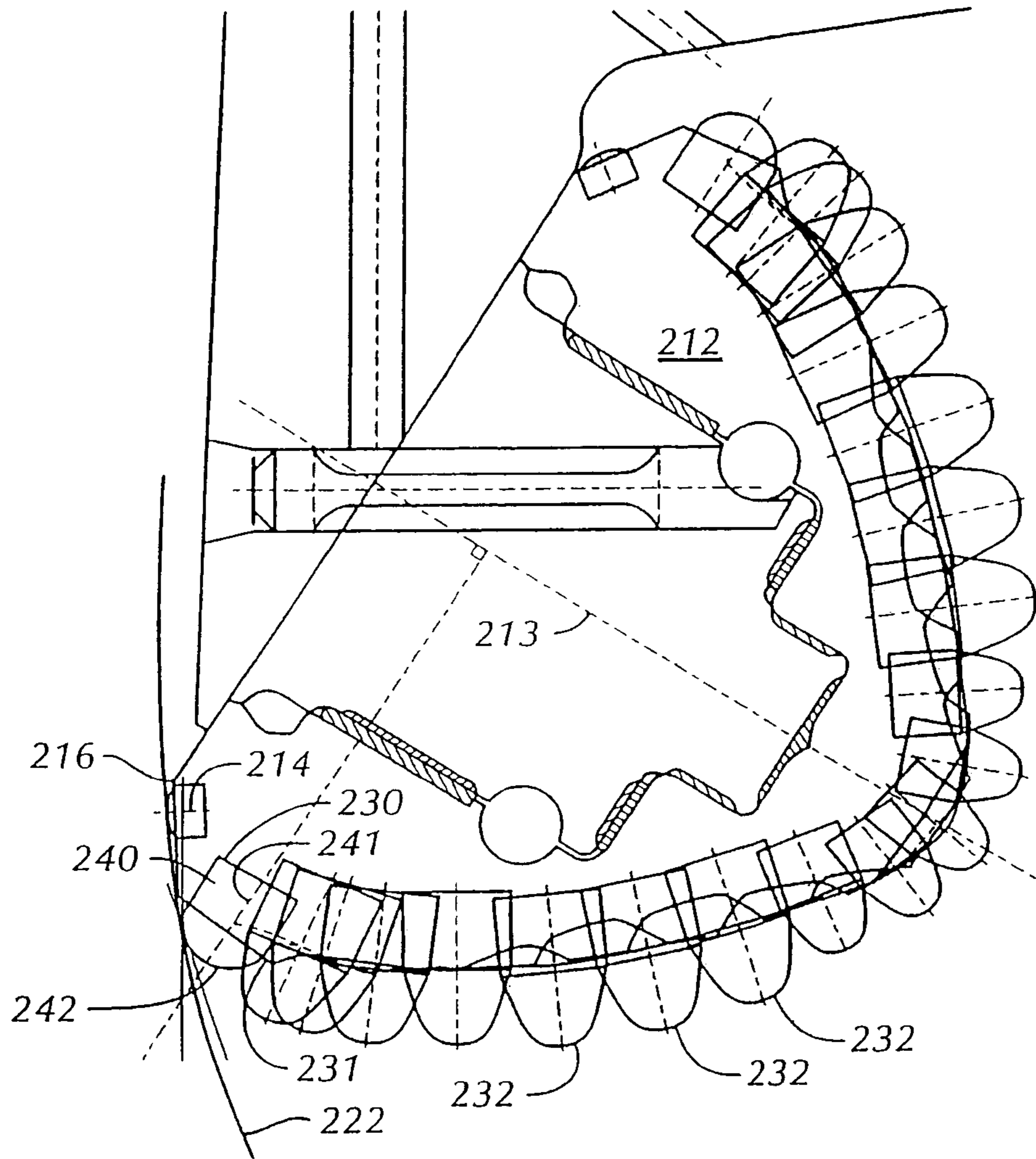
FIG. 14
