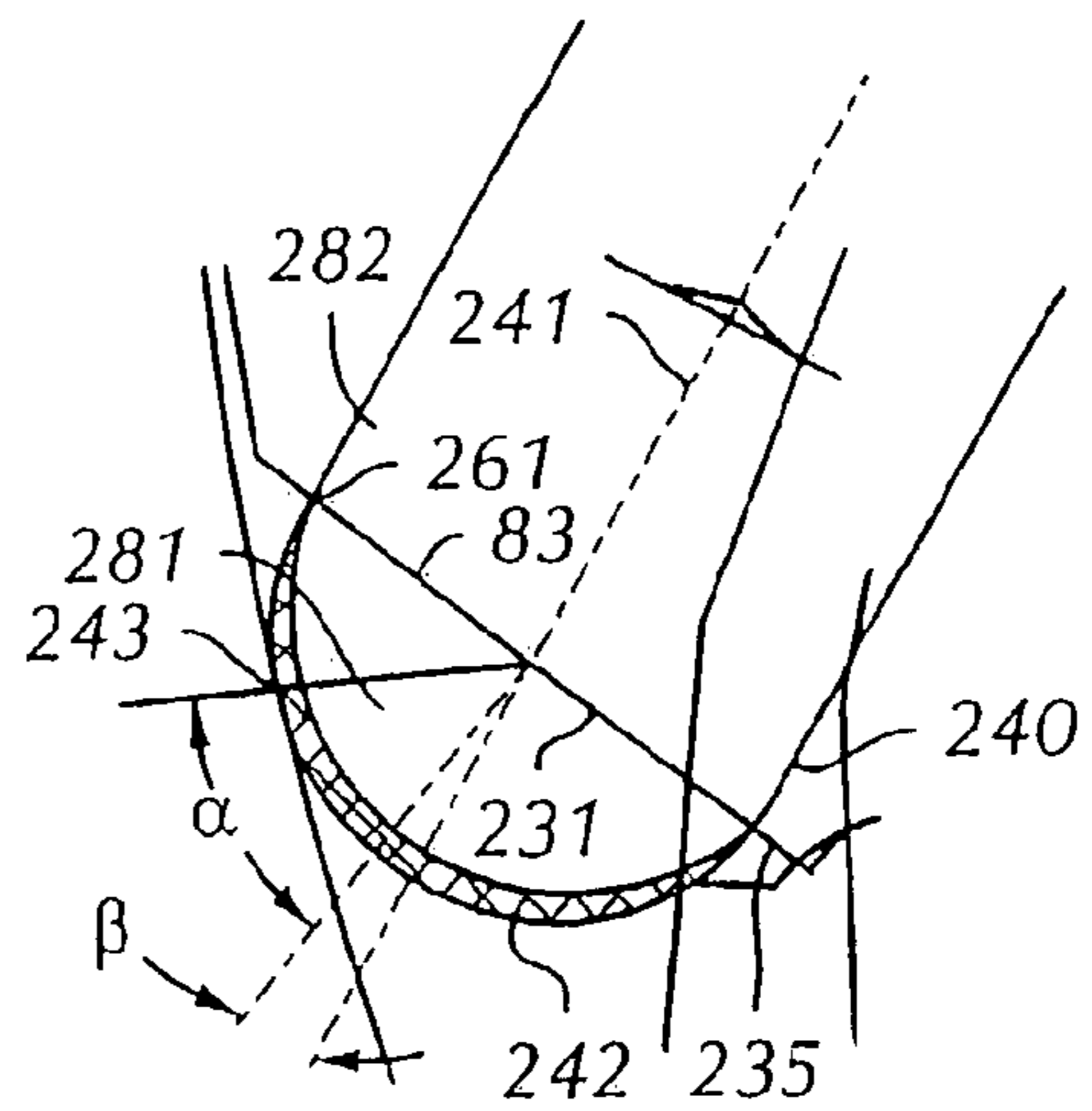
FIG. 21
