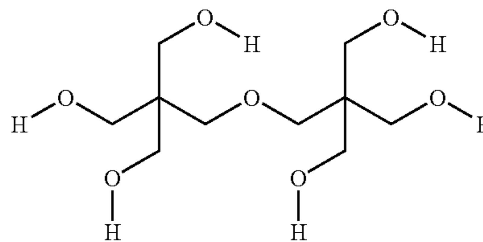
dipentaerythritol
