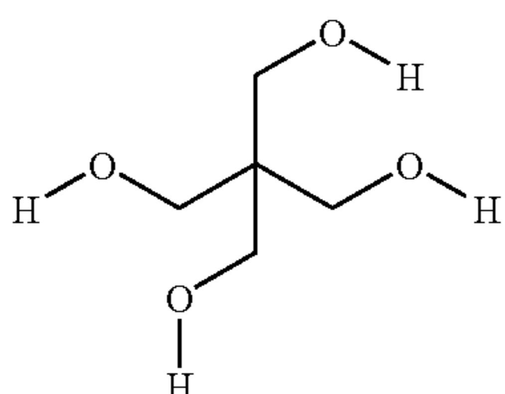
pentaerythritol
