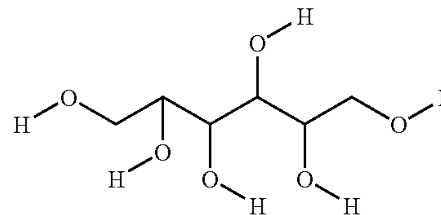
sorbitol
