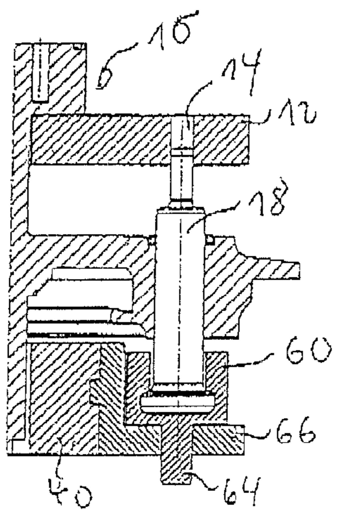
Section E - E
