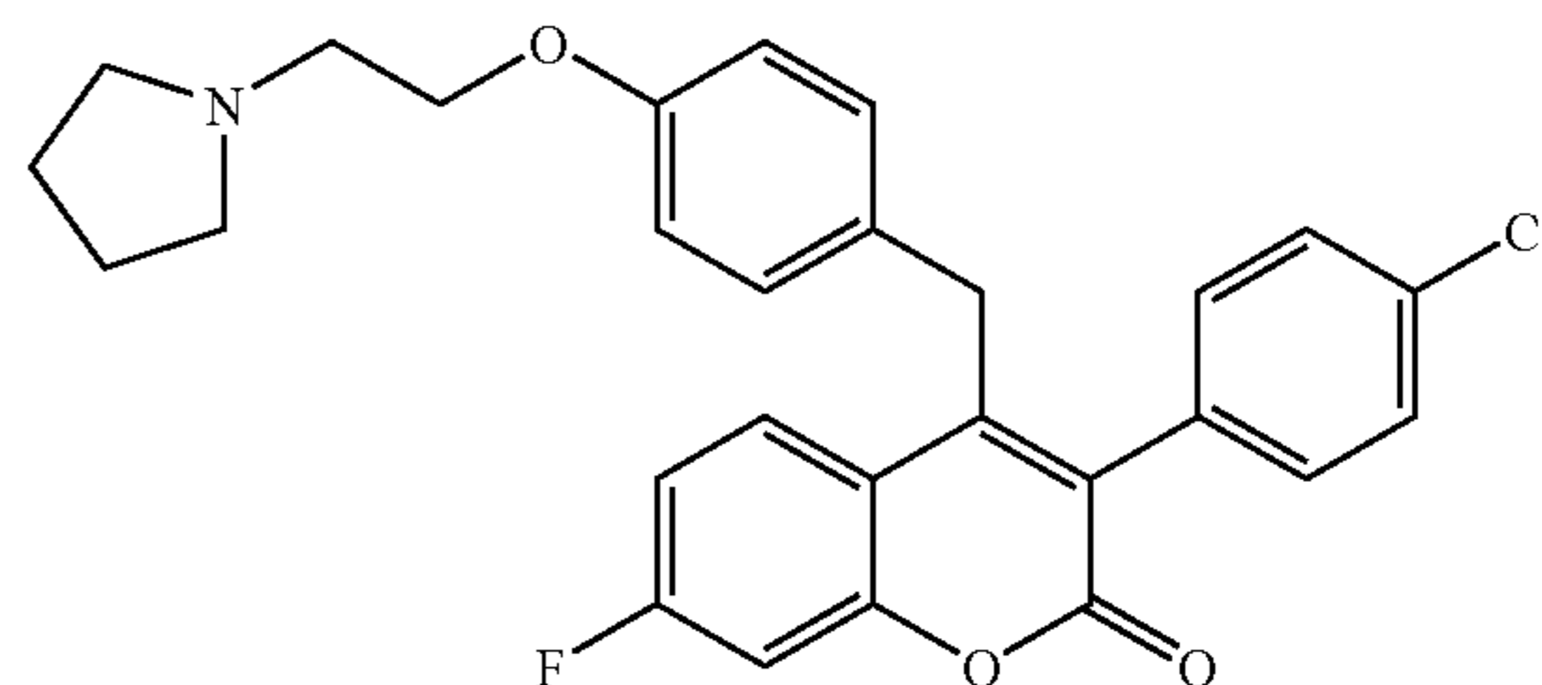
3-(4-Chloro-phenyl)-7-fluoro-4-[4-(2-pyrrolidin-1-yl-ethoxy)-benzyl]-chromen-2-one
