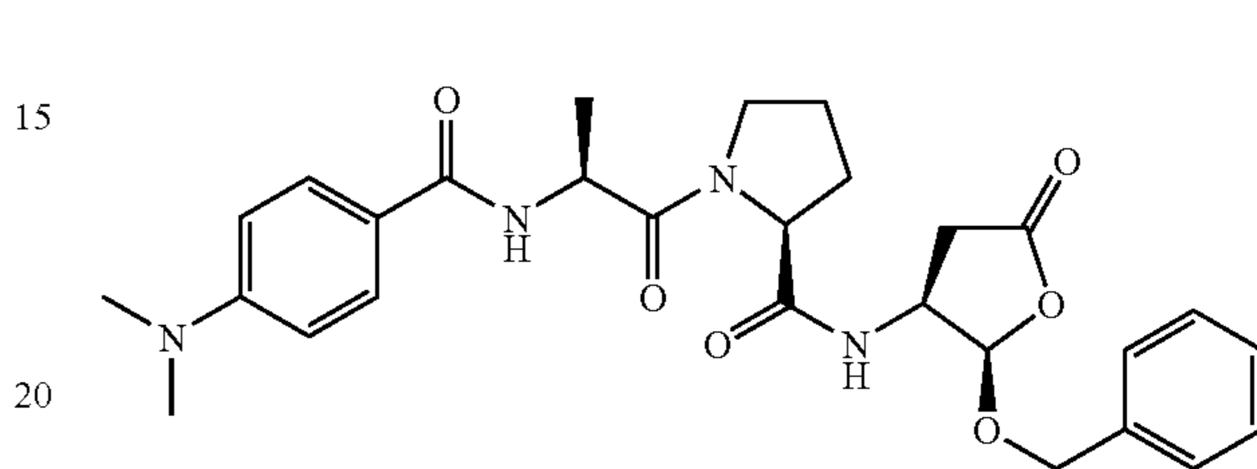
98al
