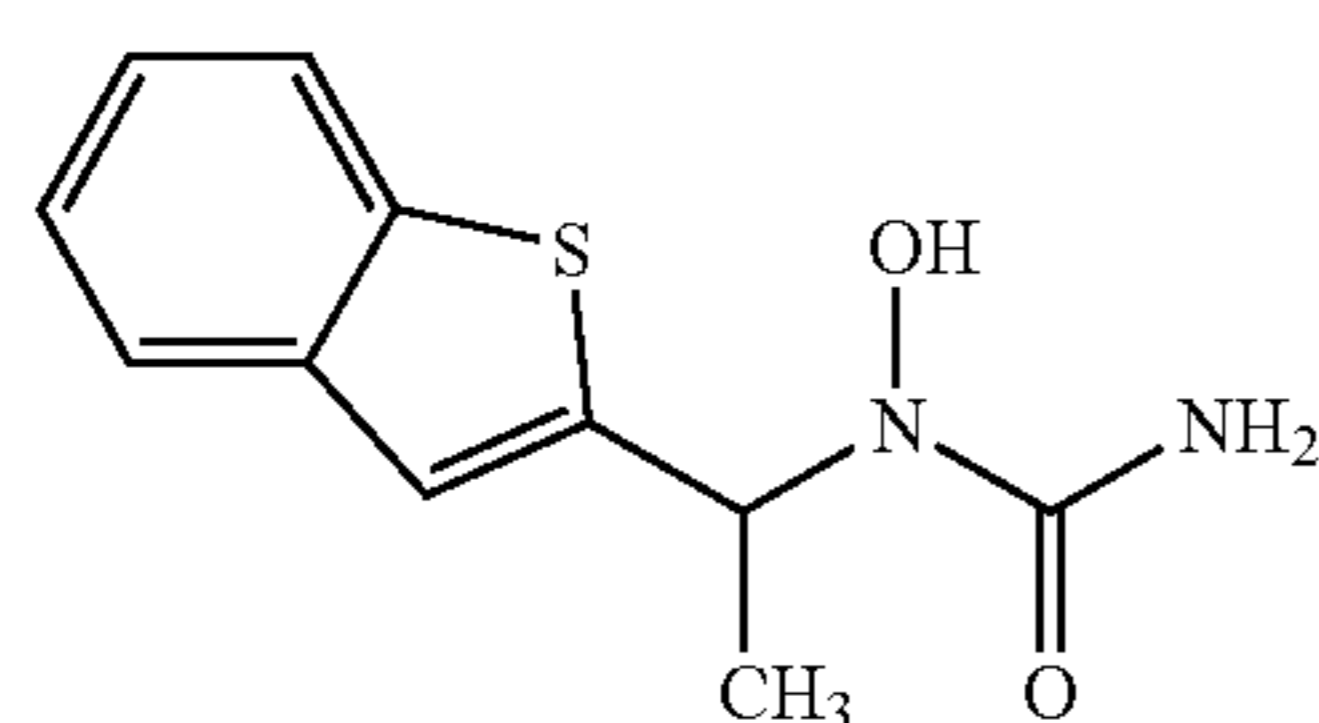
Zileuton
