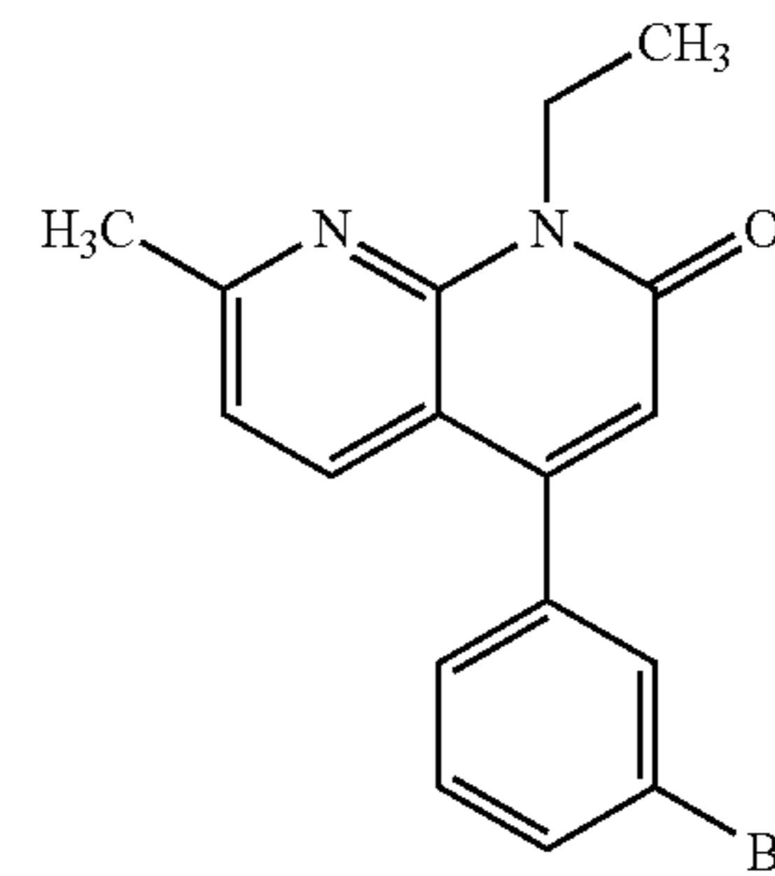
YM-58977
