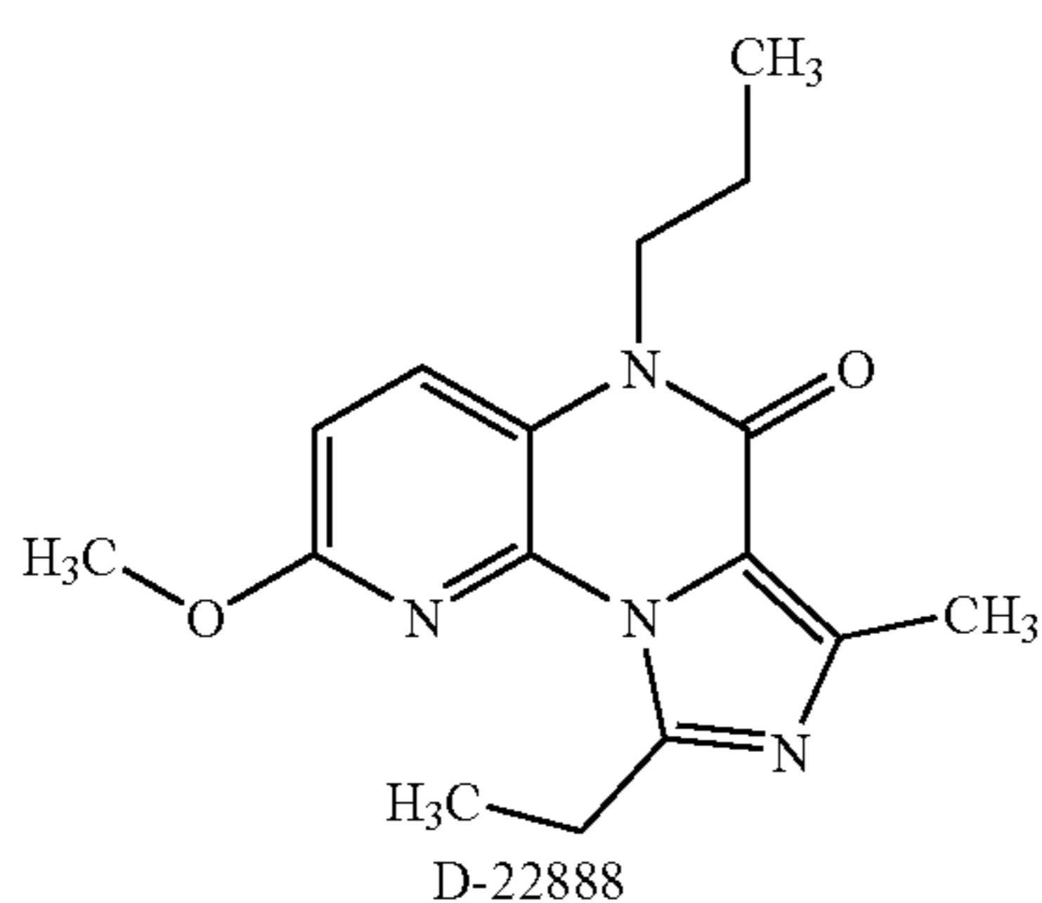
CDC-3052
