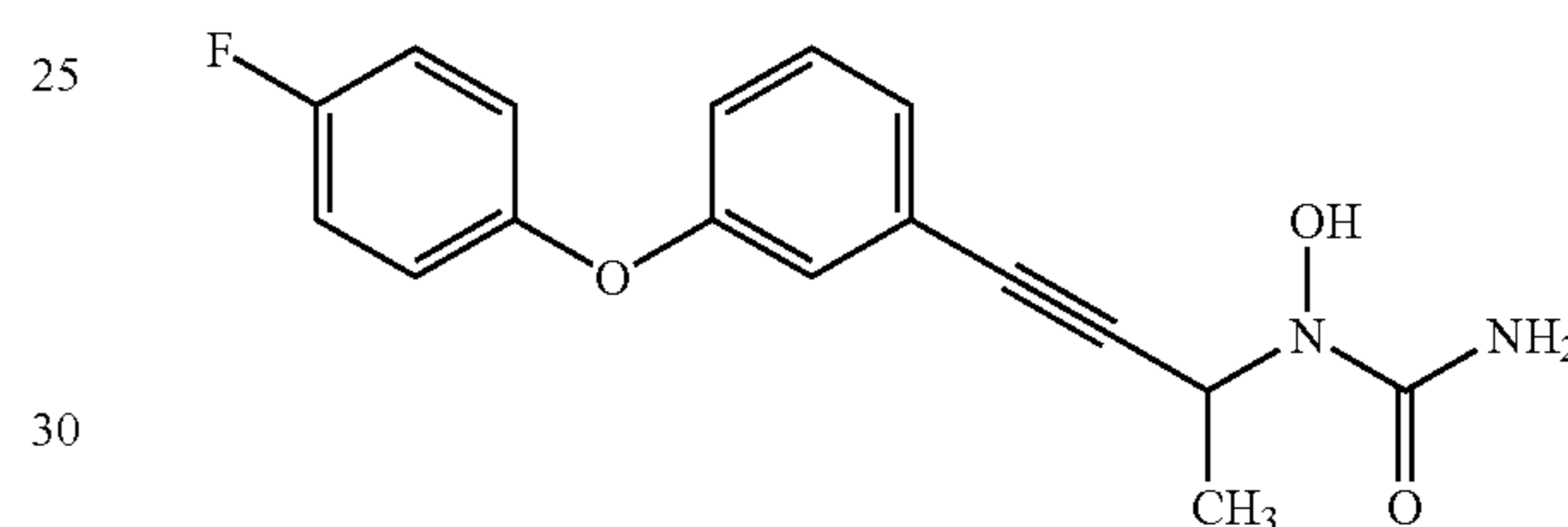
Fenleuton
