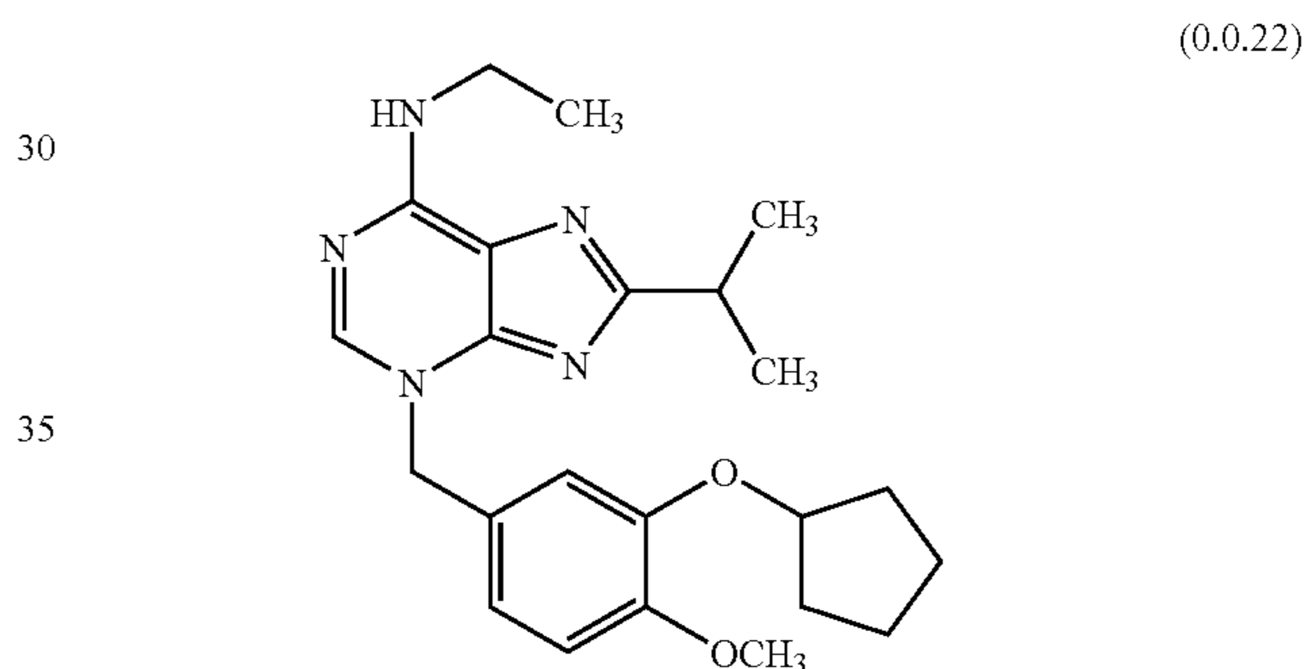
V-11294A
