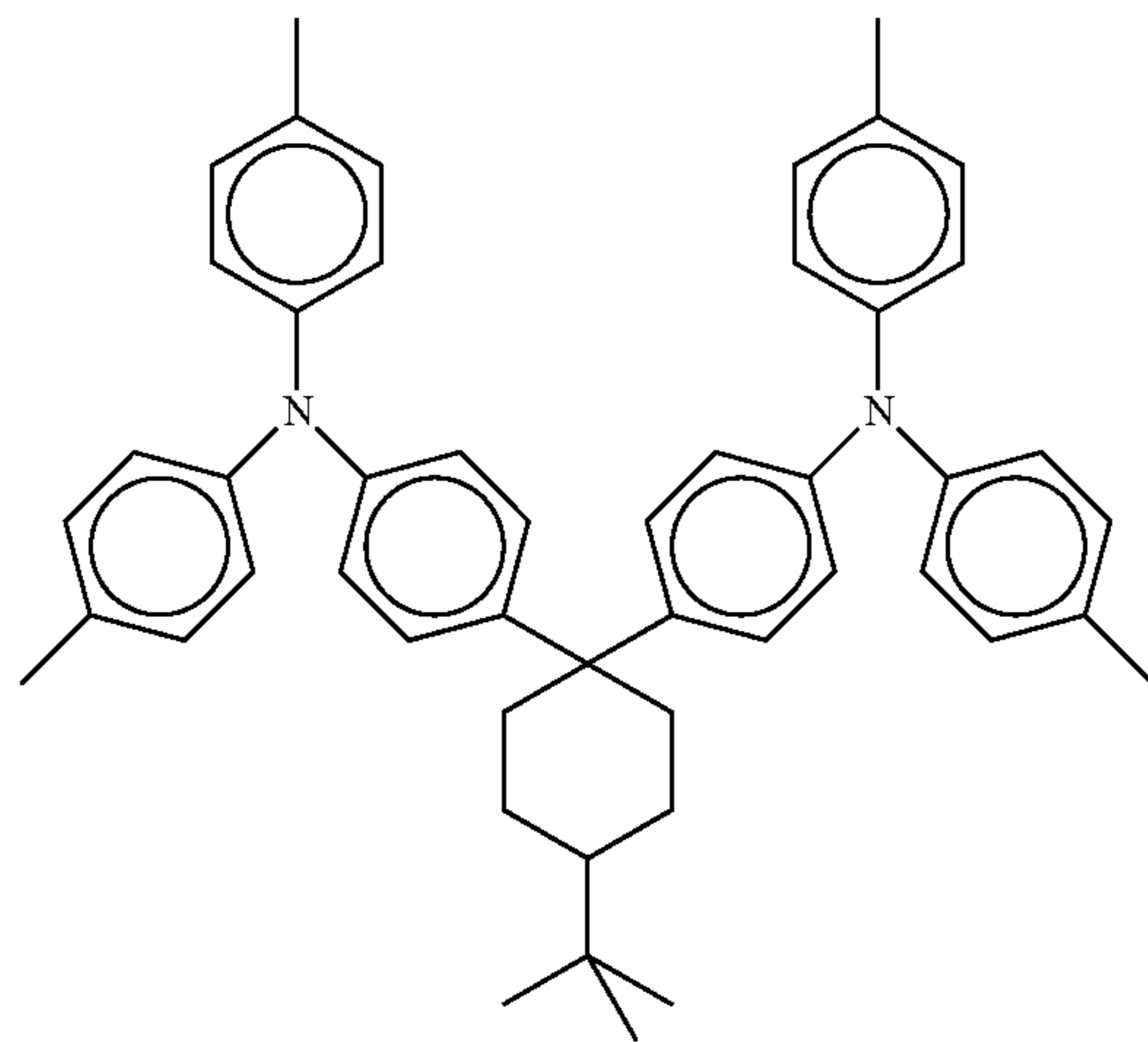
t-butylTAPC
