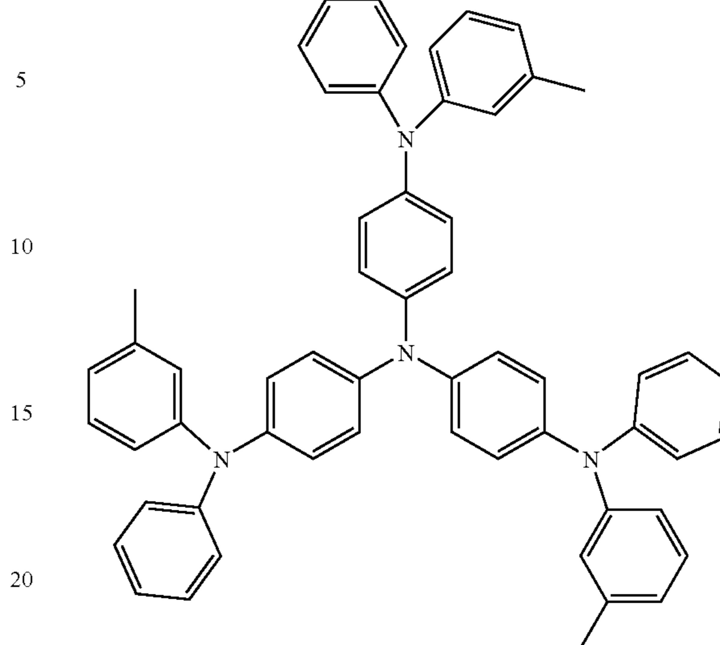
m-MTDATA
