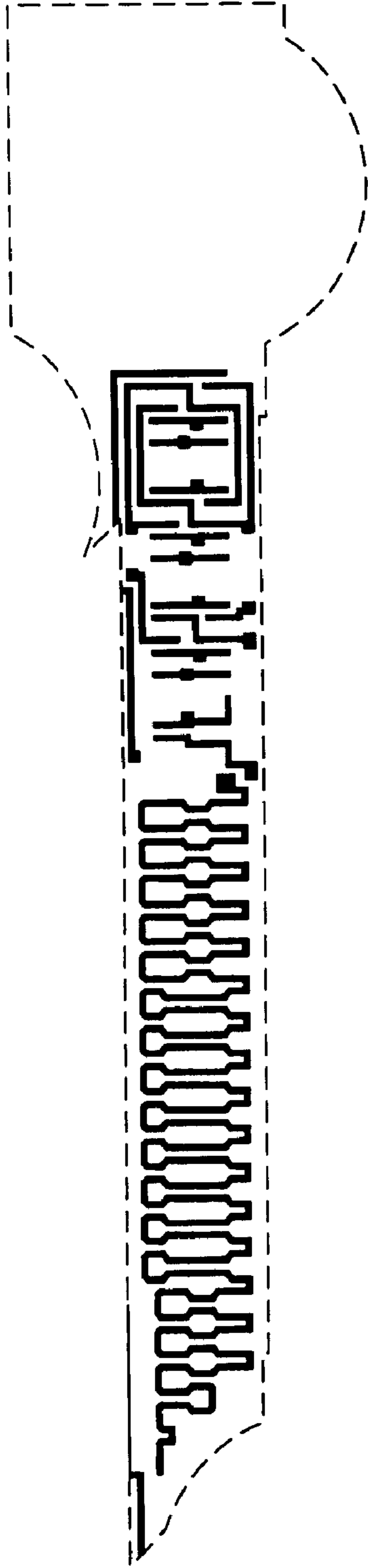
Poly mask
