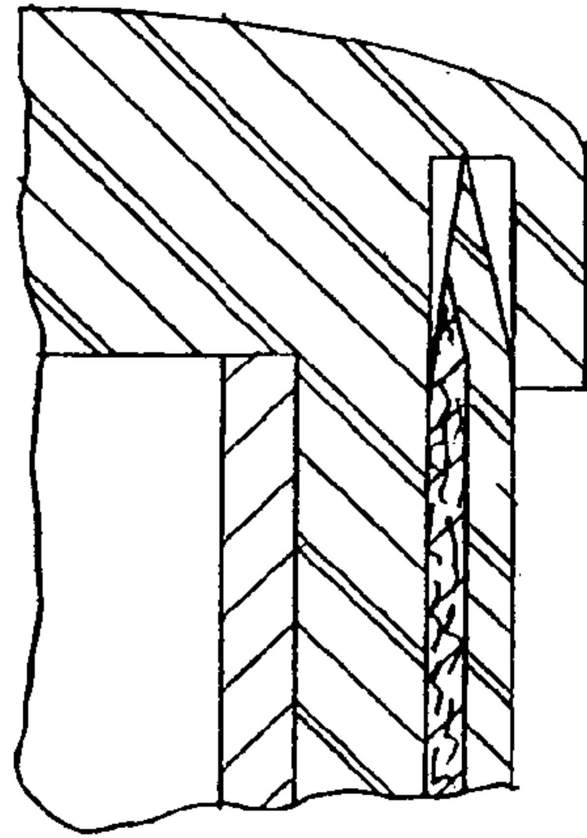
FIG. 24
