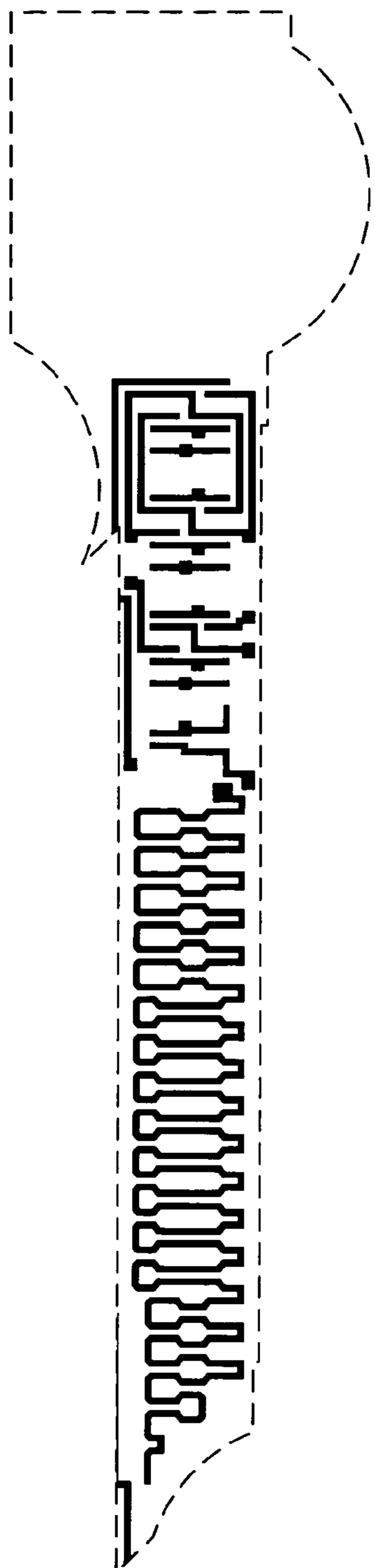
Poly mask
