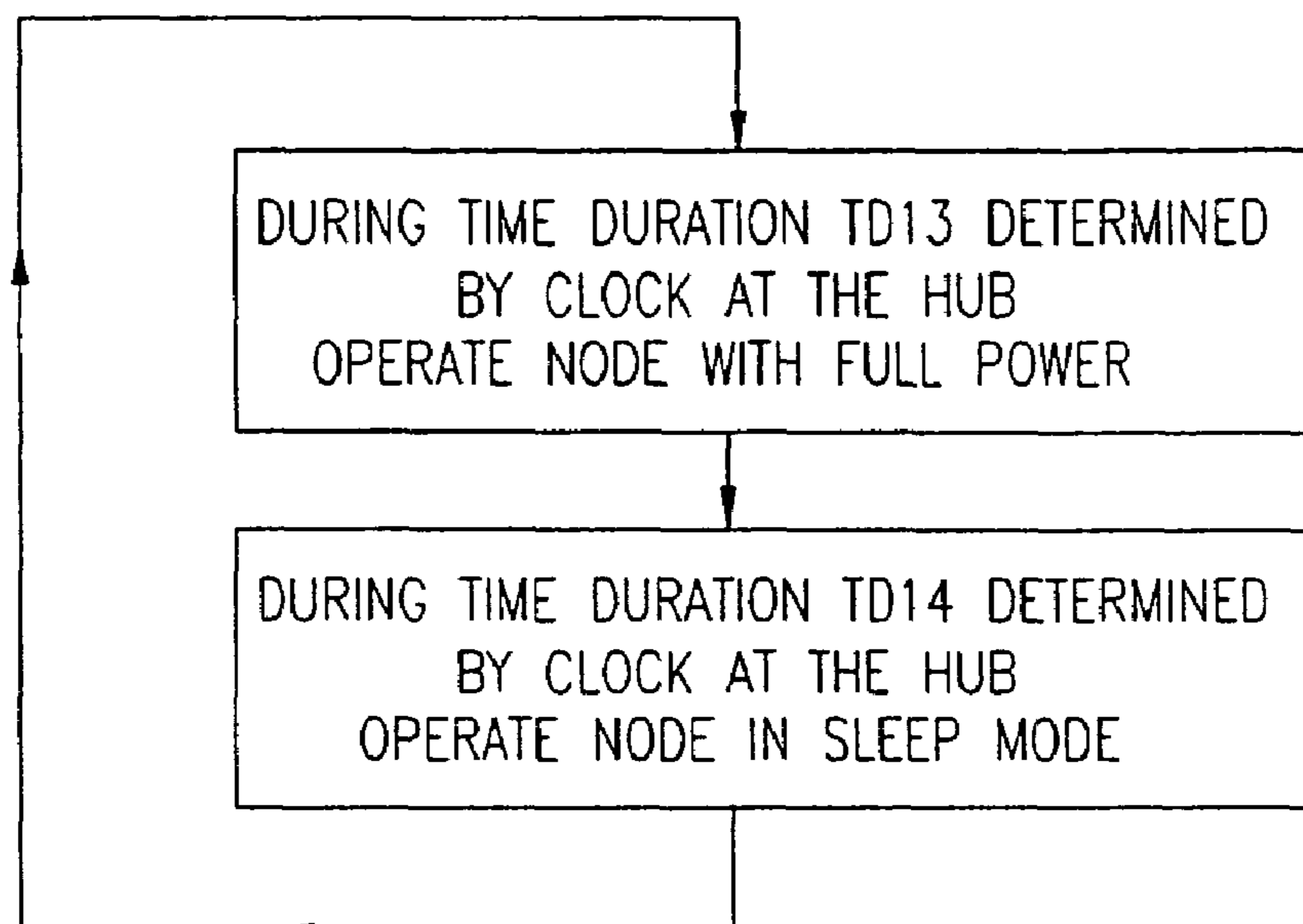
FIG. 22C
