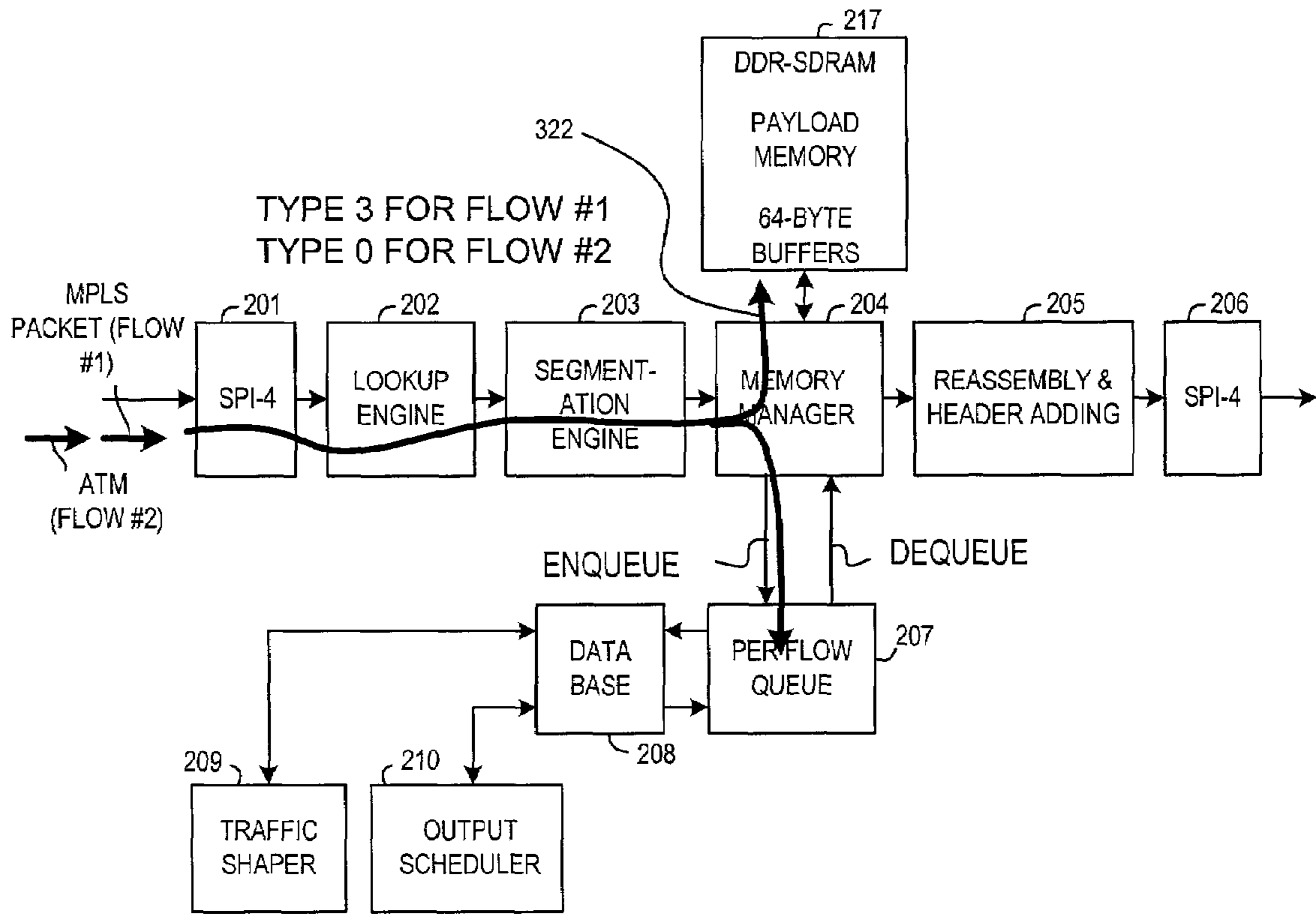
INGRESS MODE
