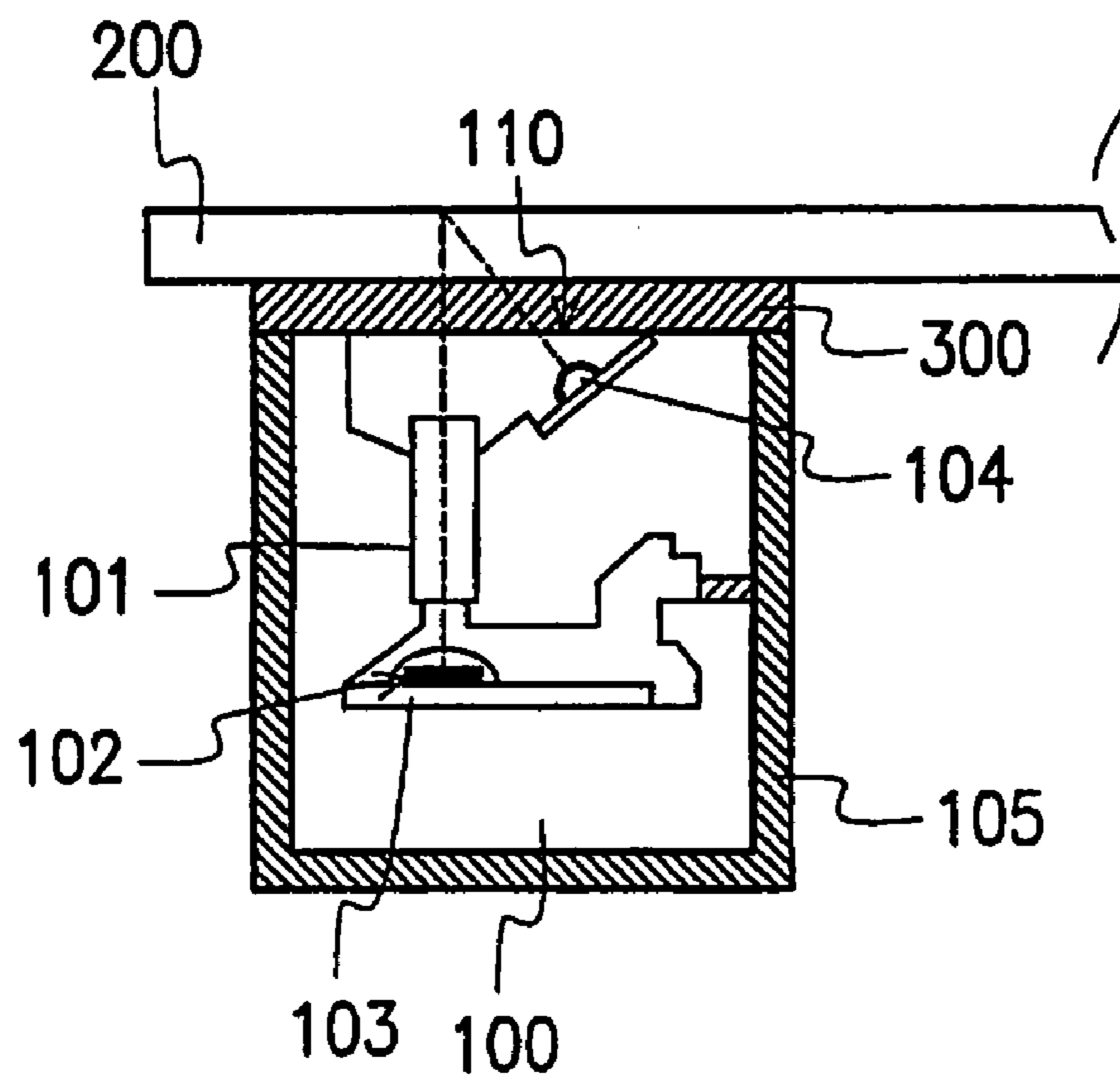
FIG. 1b(PRIOR ART)
