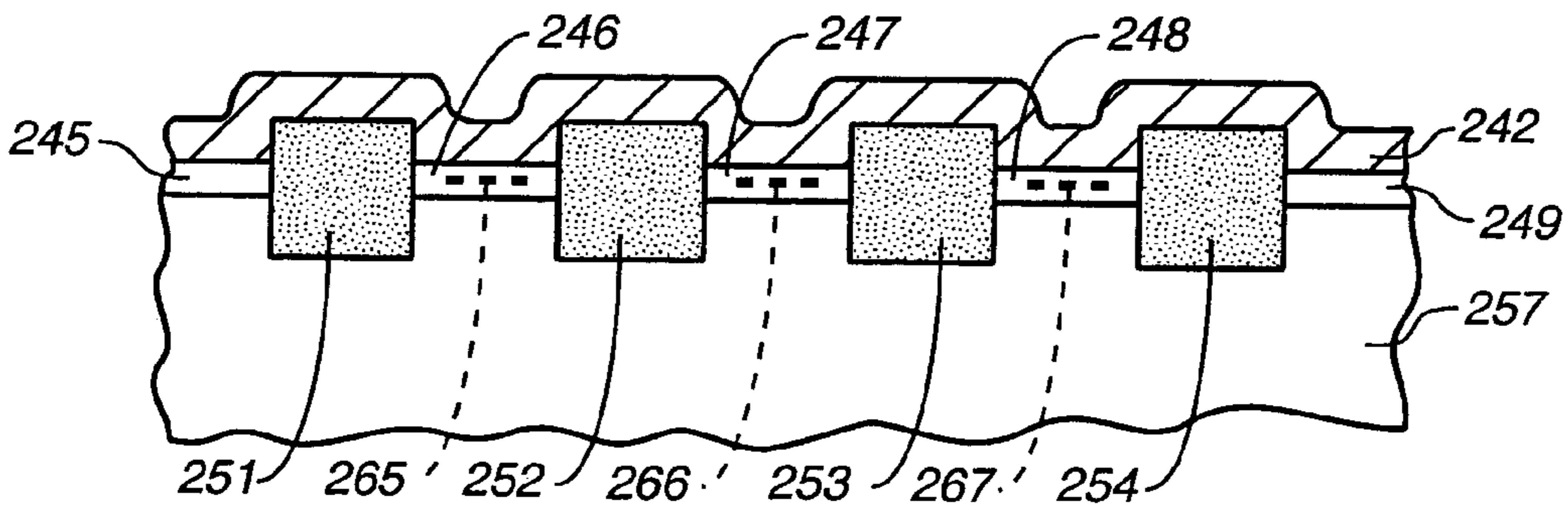
(SECTION VII-VII) FIG. 23A
