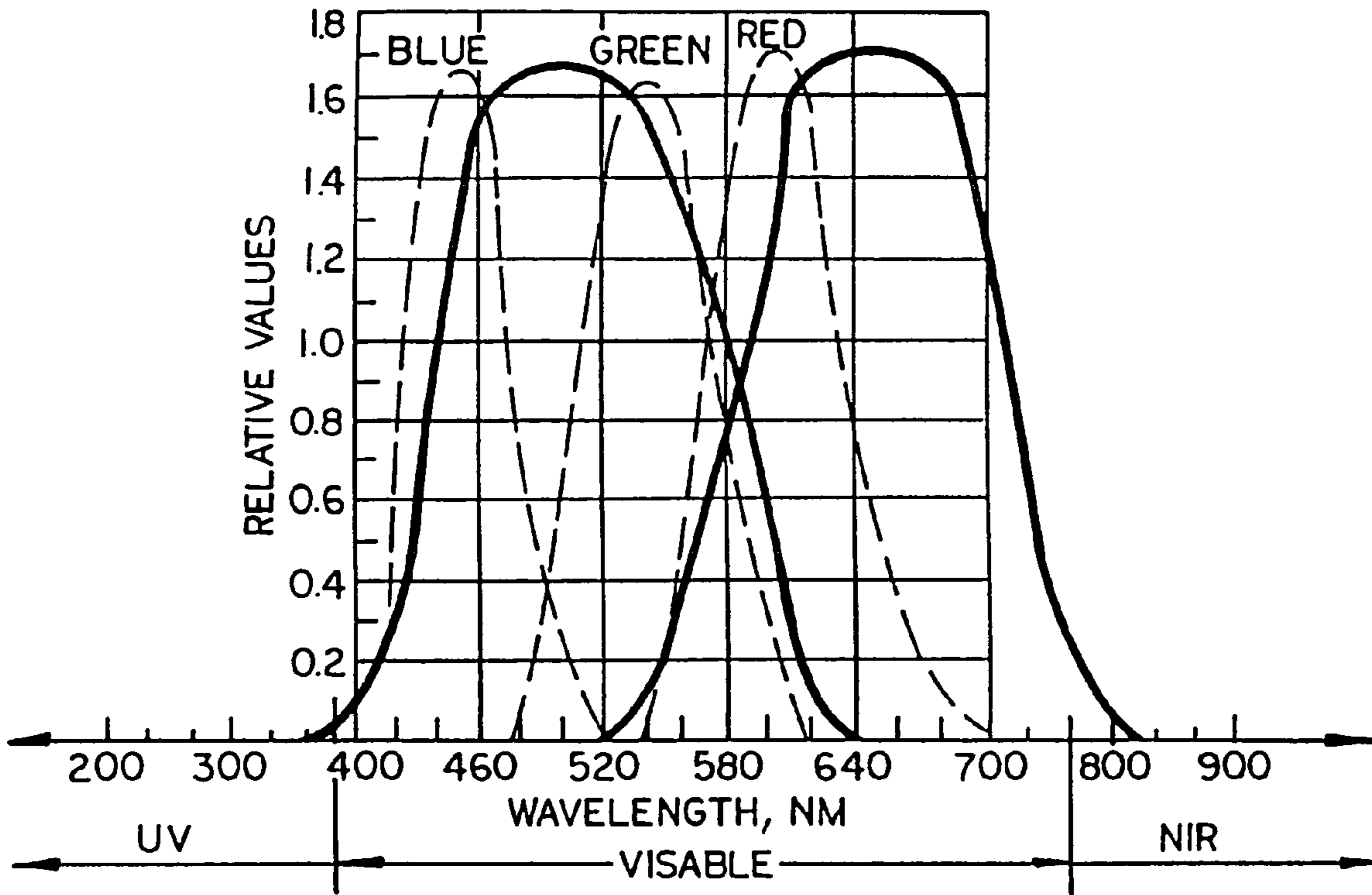
FIG. 8c
