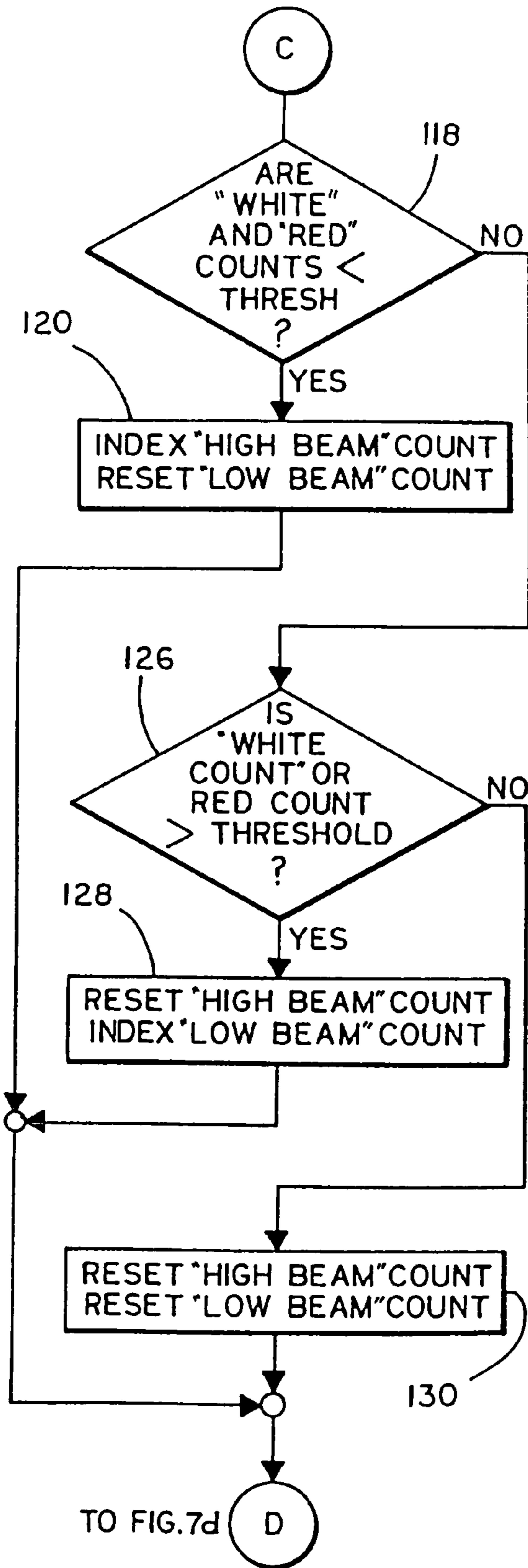
FIG. 7c
