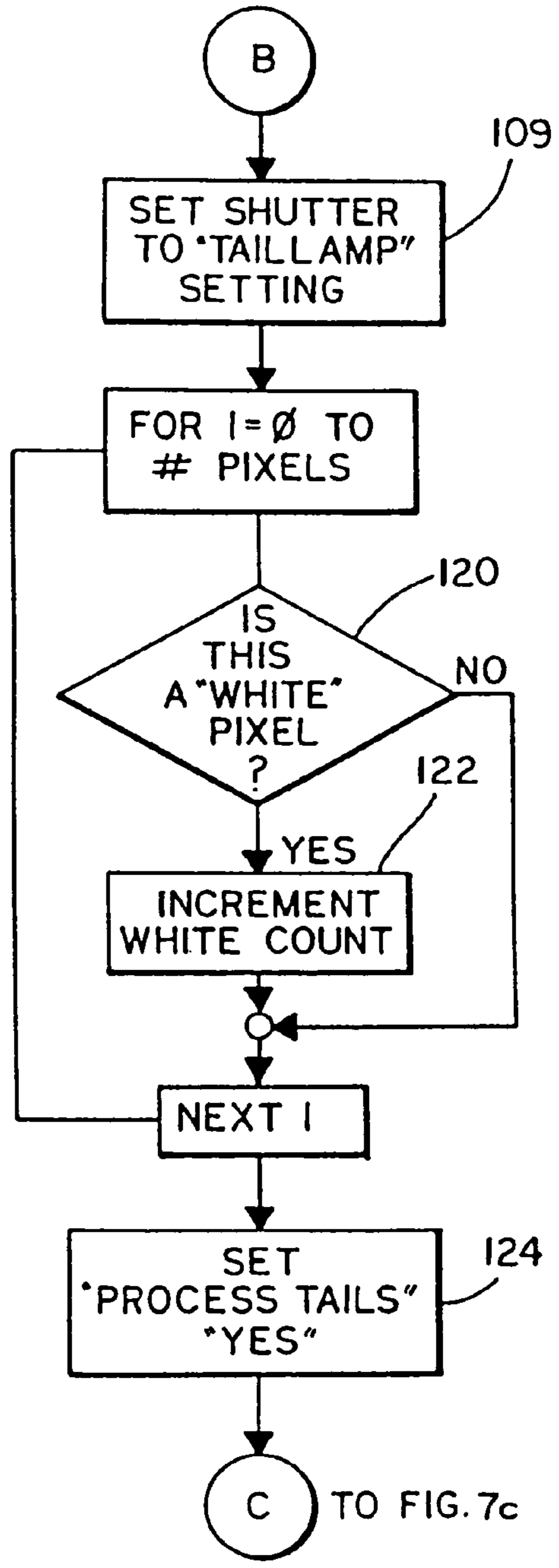
FIG. 7b
