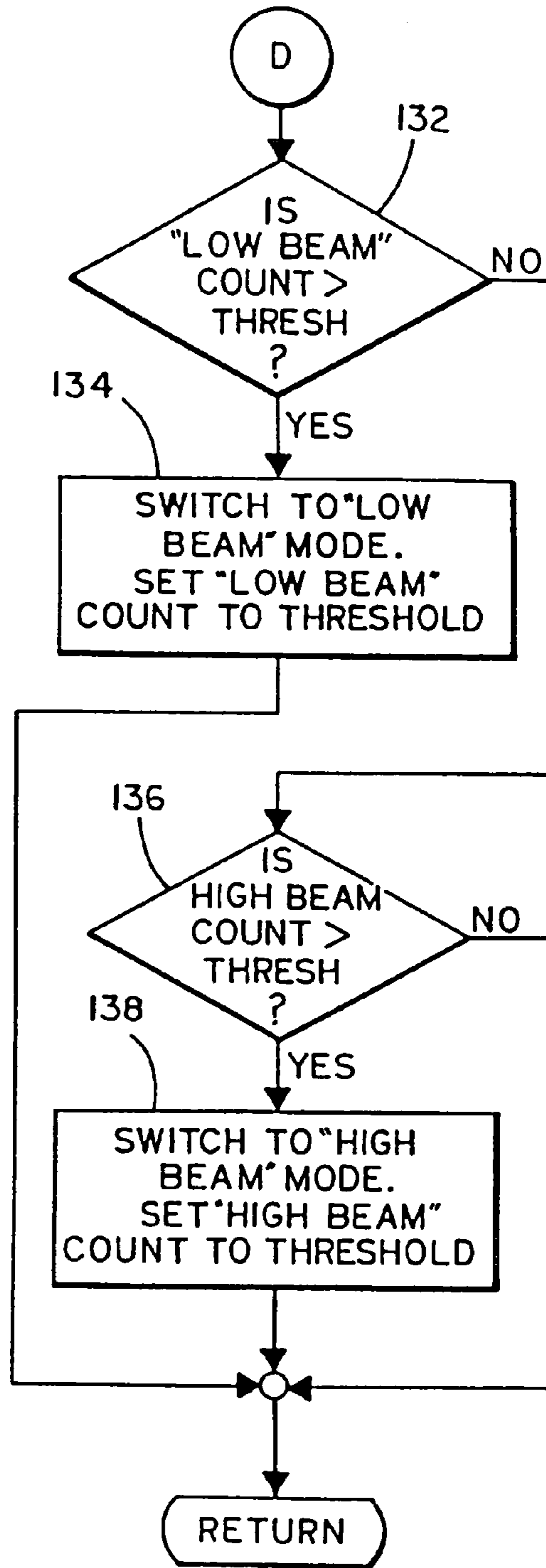
FIG. 7d
